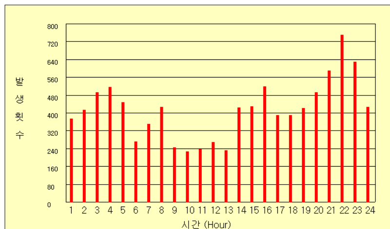
그림 40(b). 2007년 11월 시간별 낙뢰발생 횟수
