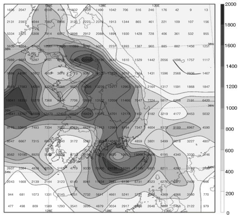
그림 17(a). 2007년 낙뢰발생 횟수 분포도
