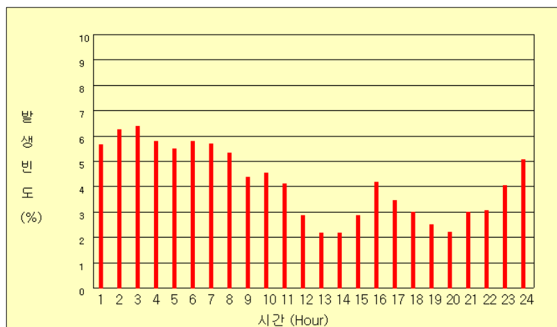
그림 46(b). 2003년 시간별 낙뢰발생 빈도
