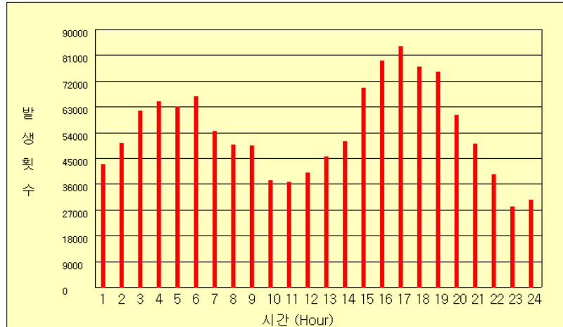
그림 46(e). 2005년 시간별 낙뢰발생 횟수
