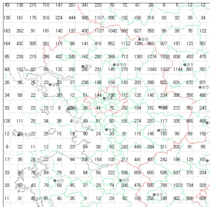
그림 24(d). 2007년 7월 경기도지역 낙뢰발생 횟수
