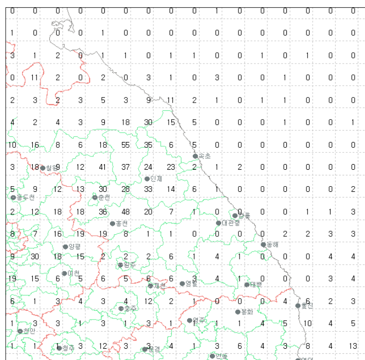
그림 25(f). 2007년 9월 강원도지역 낙뢰발생 횟수
