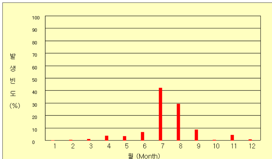
그림 47(d). 2004년 월별 낙뢰발생 횟수
