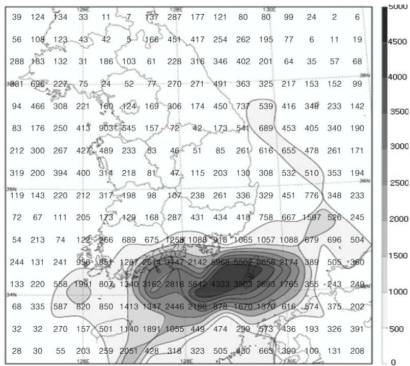
그림 15(a). 2007년 가을철의 낙뢰발생 횟수 분포도
