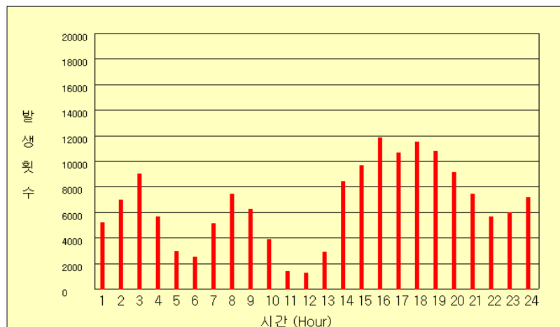
그림 35(b). 2007년 6월 시간별 낙뢰발생 횟수
