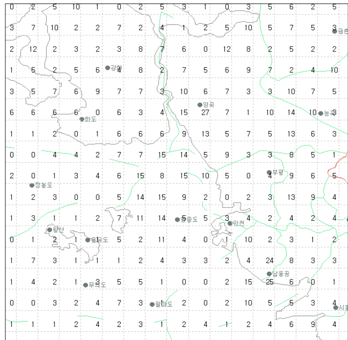
그림 22(e). 2007년 8월 인천지역 낙뢰발생 횟수
