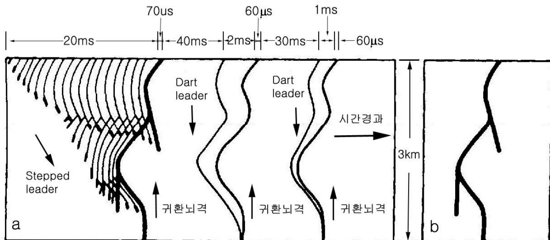
그림 C. 카메라에 잡힌 낙뢰발생과정의 모형도 (a)삼중낙뢰의 시간경과를 보이는 모델도 (b)정지도
