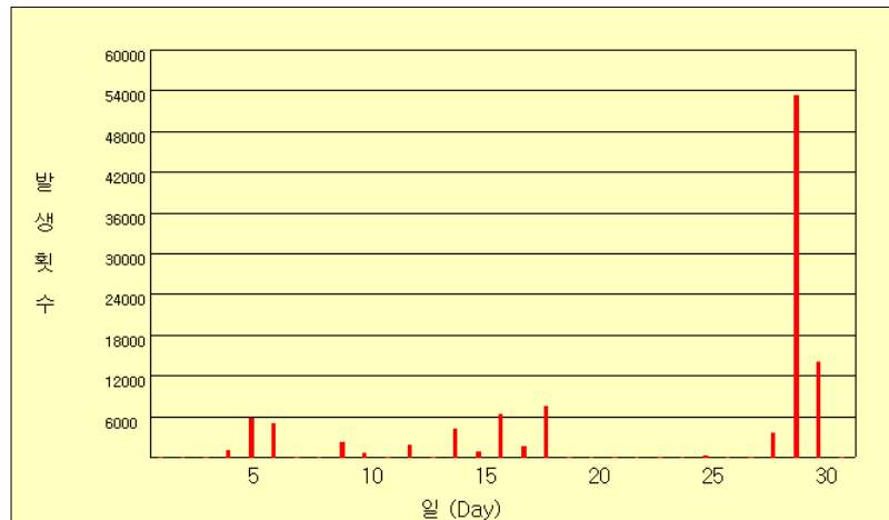
그림 34(a). 2007년 5월 일별 낙뢰발생 횟수
