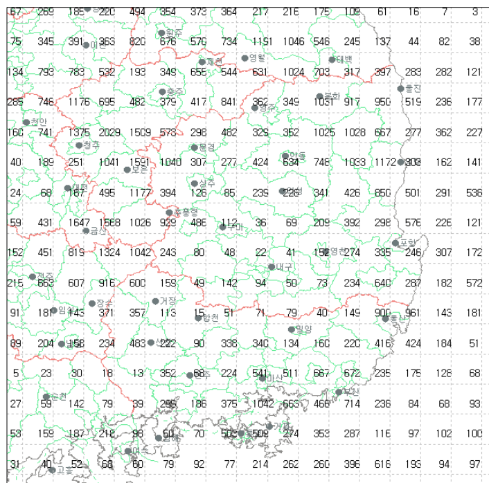
그림 27(d). 2007년 7월 경상도지역 낙뢰발생 횟수
