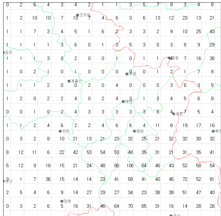
그림 20(d). 2007년 7월 대전지역 낙뢰발생 횟수
