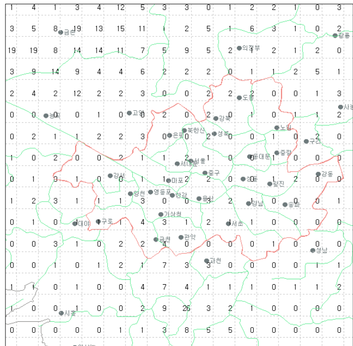
그림 18(b). 2007년 5월 서울지역 낙뢰발생 횟수
