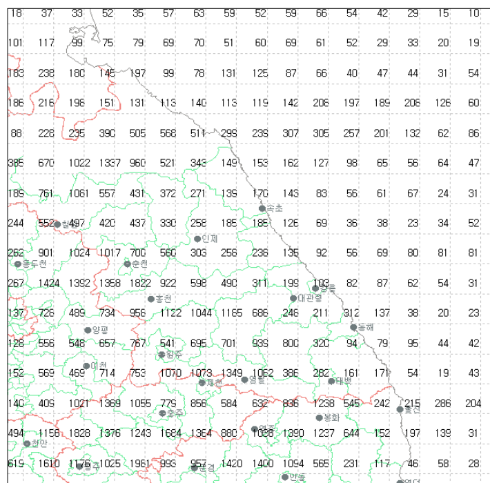
그림 25(e). 2007년 8월 강원도지역 낙뢰발생 횟수
