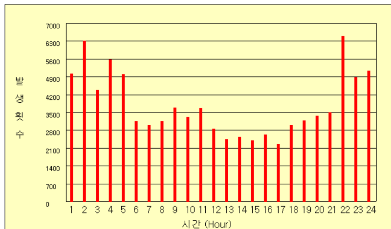
그림 38(b). 2007년 9월 시간별 낙뢰발생 횟수
