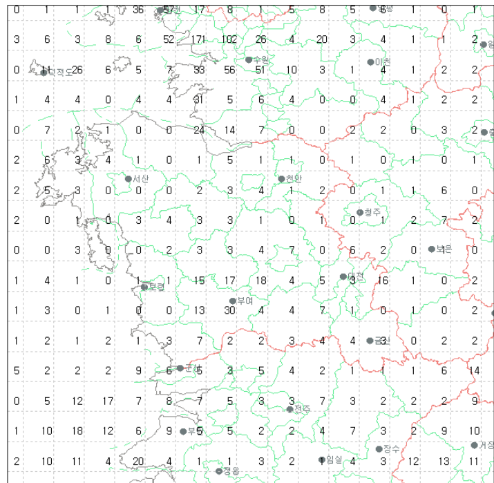
그림 26(f). 2007년 9월 충청도지역 낙뢰발생 횟수
