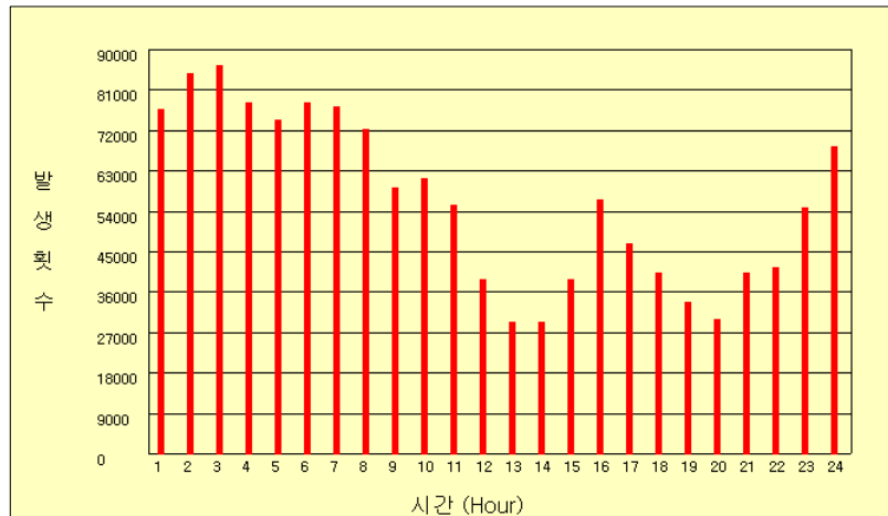
그림 46(a). 2003년 시간별 낙뢰발생 횟수
