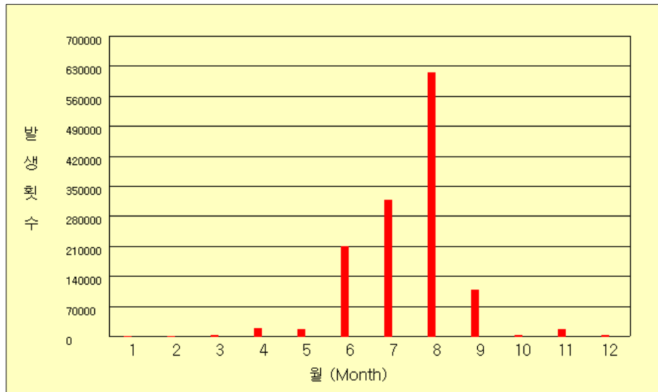
그림 47(e). 2005년 월별 낙뢰발생 횟수
