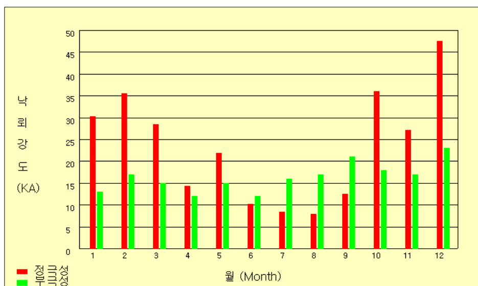
그림 48(b). 2004년 월별 평균 강도
