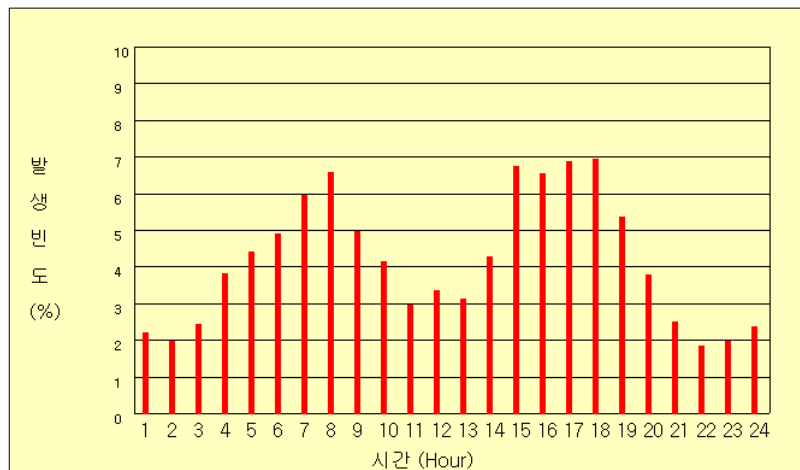
그림 46(d). 2004년 시간별 낙뢰발생 빈도
