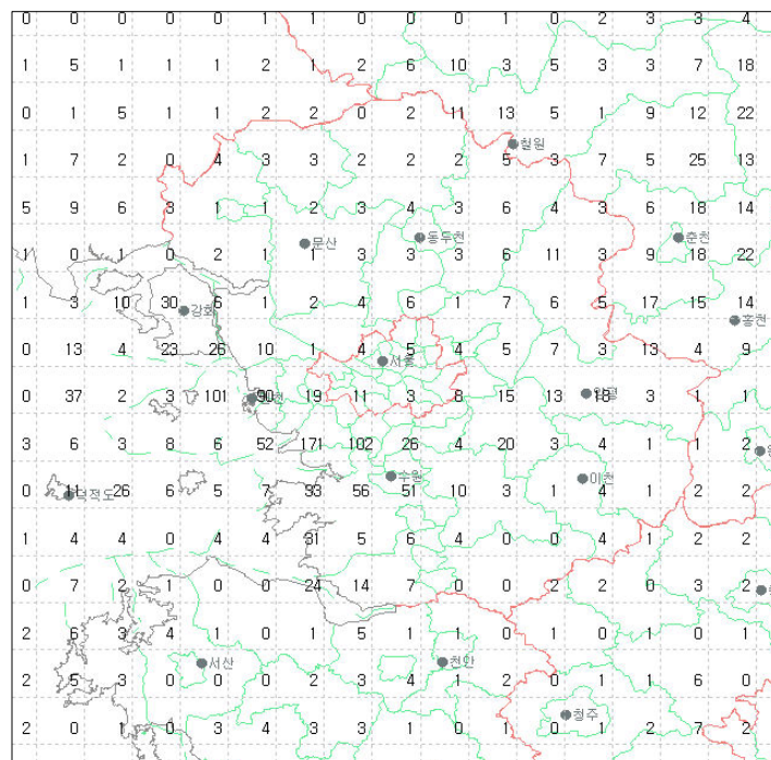
그림 24(f). 2007년 9월 경기도지역 낙뢰발생 횟수
