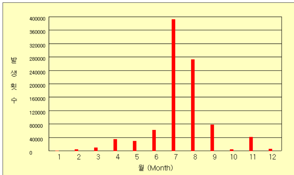
그림 47(c). 2004년 월별 낙뢰발생 횟수
