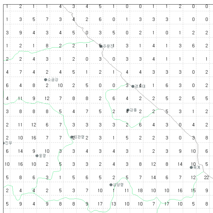
그림 23(e). 2007년 8월 강릉지역 낙뢰발생 횟수
