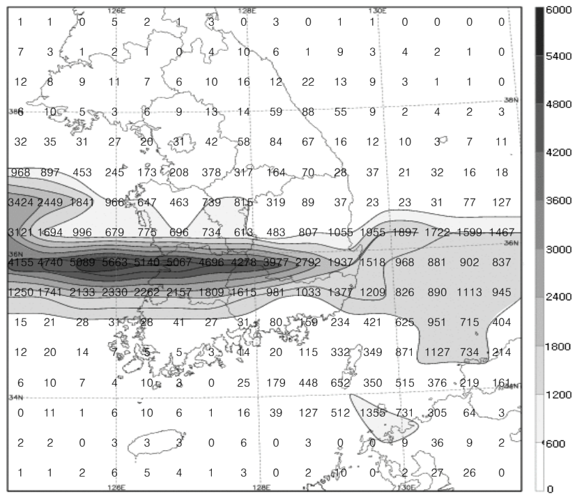
그림 3(a). 2007년 3월의 낙뢰발생 횟수 분포도
