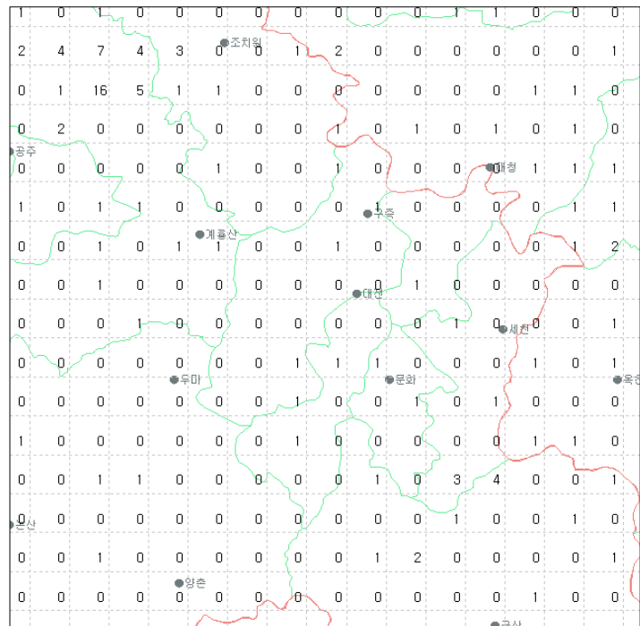
그림 20(b). 2007년 5월 대전지역 낙뢰발생 횟수
