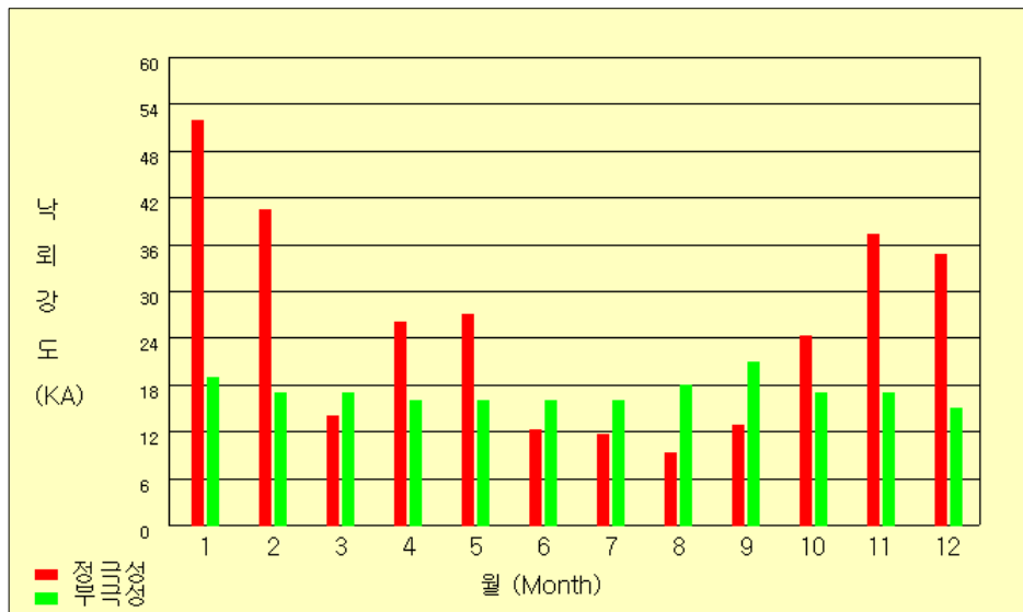
그림 48(e). 2007년 월별 평균 강도
