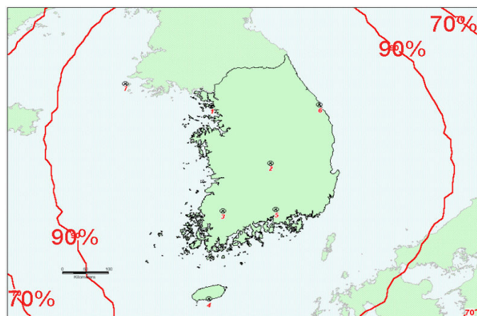
그림 12. 낙뢰탐지범위
