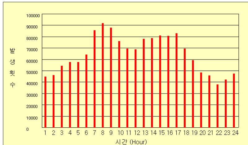
그림 46(i). 2007년 시간별 낙뢰발생 횟수
