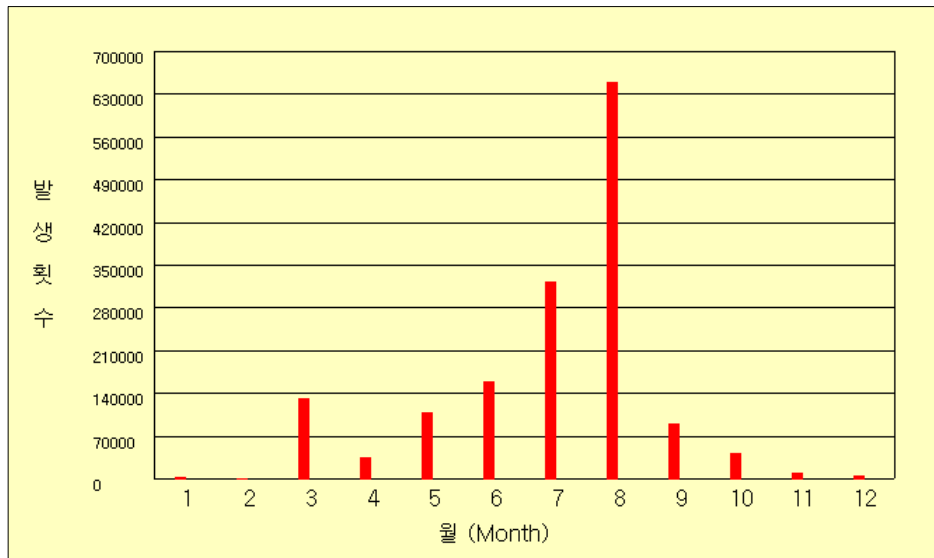
그림 47(i). 2007년 월별 낙뢰발생 횟수
