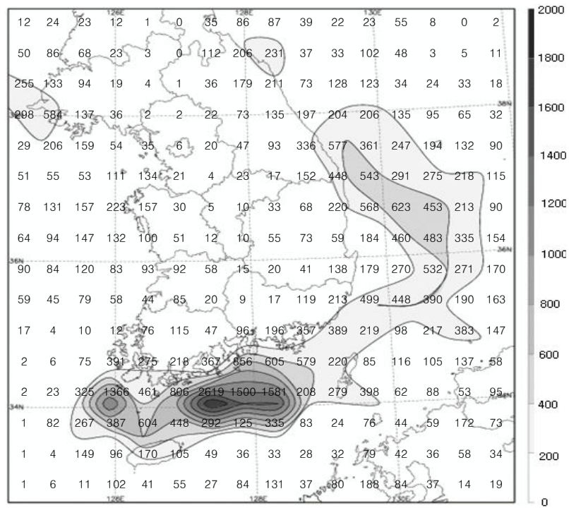
그림 10(a). 2007년 10월의 낙뢰발생 횟수 분포도
