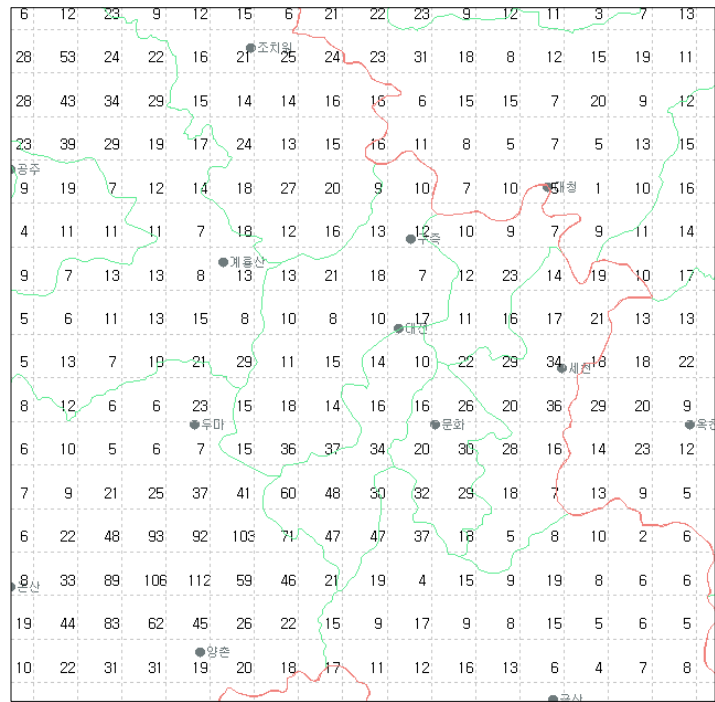
그림 20(e). 2007년 8월 대전지역 낙뢰발생 횟수
