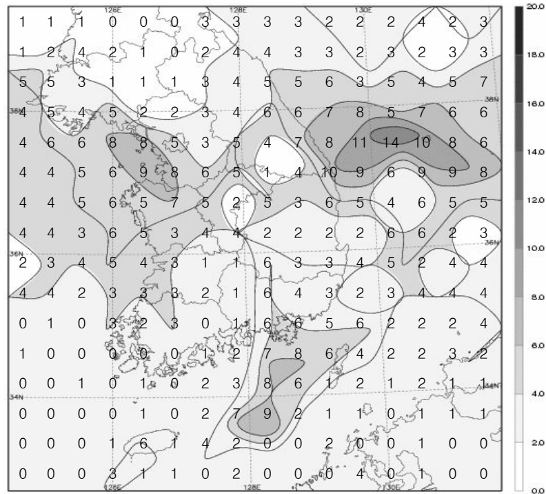
그림 11(b). 2007년 11월의 낙뢰발생 일수 분포도
