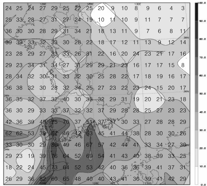
그림 14(b). 2007년 여름철의 낙뢰발생 일수 분포도
