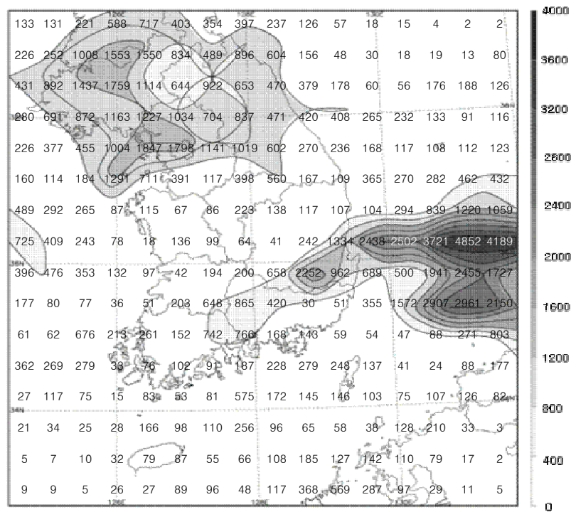
그림 5(a). 2007년 5월의 낙뢰발생 횟수 분포도
