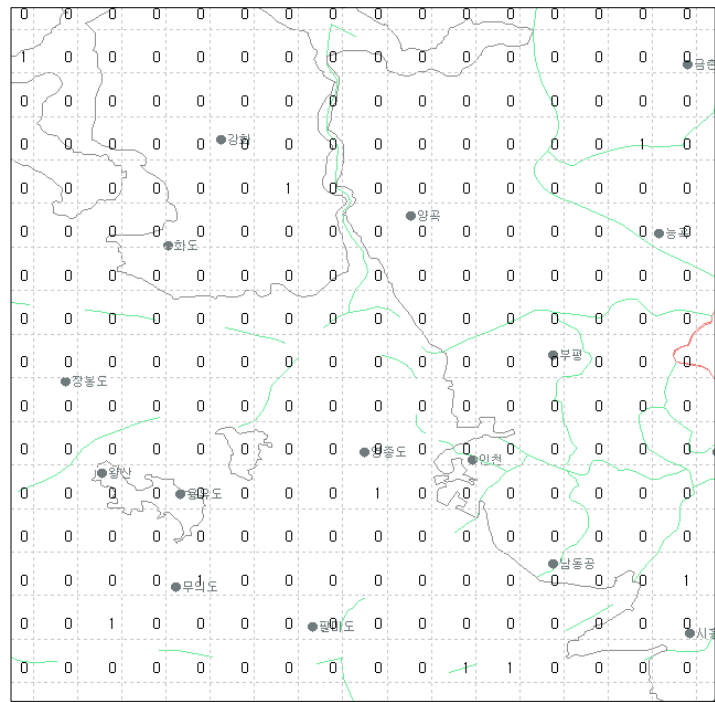
그림 22(a). 2007년 4월 인천지역 낙뢰발생 횟수
