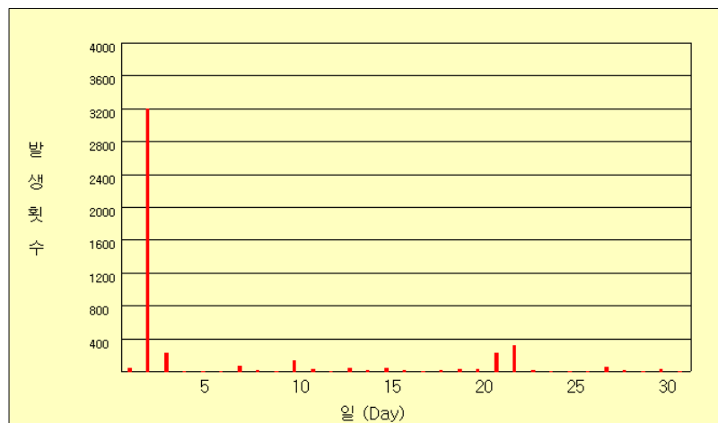
그림 41(a). 2006년 12월 일별 낙뢰발생 횟수
