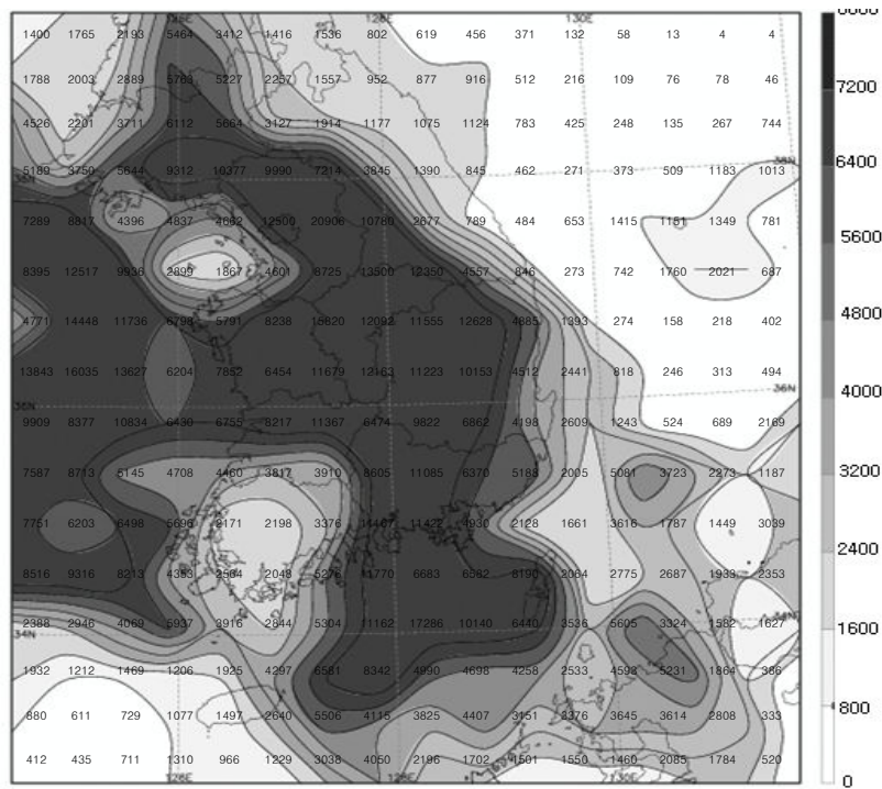
그림 14(a). 2007년 여름철의 낙뢰발생 횟수 분포도
