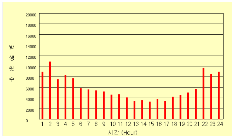
그림 44. 2007년 가을(9~11월) 시간별 낙뢰발생 횟수
