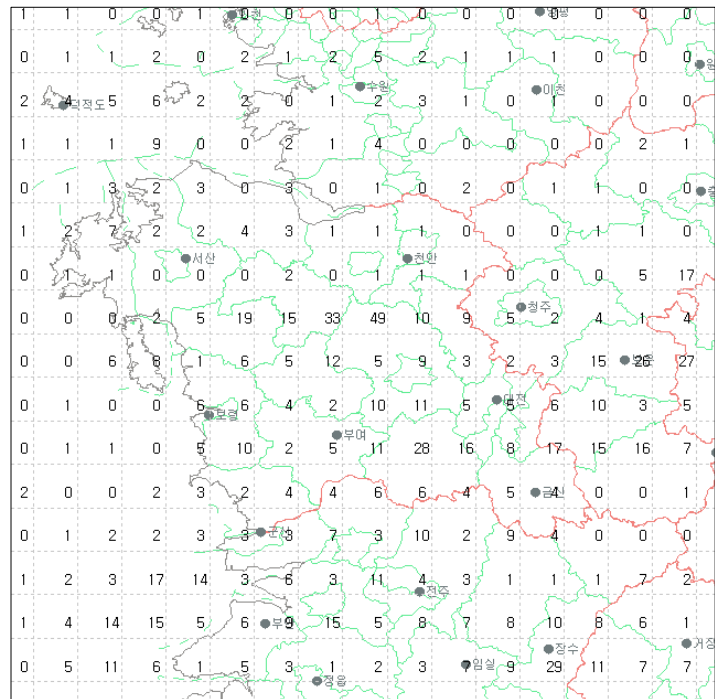
그림 26(a). 2007년 4월 충청도지역 낙뢰발생 횟수
