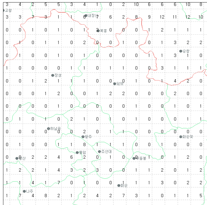
그림 21(d). 2007년 7월 광주지역 낙뢰발생 횟수
