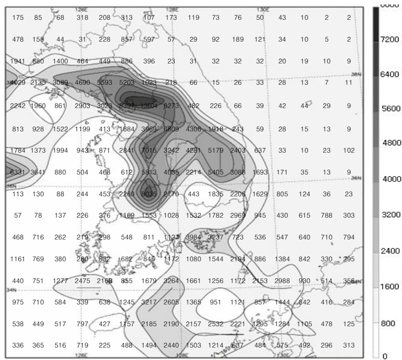
그림 7(a). 2007년 7월의 낙뢰발생 횟수 분포도
