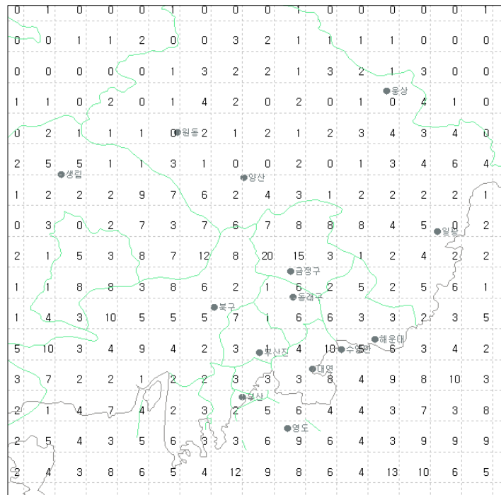
그림 19(a). 2007년 4월 부산지역 낙뢰발생 횟수
