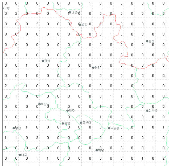
그림 21(a). 2007년 4월 광주지역 낙뢰발생 횟수
