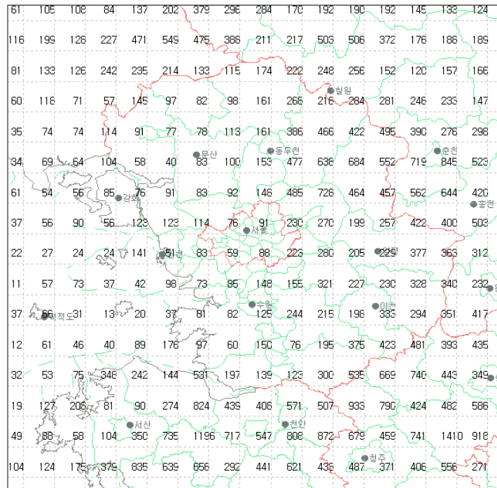
그림 24(e). 2007년 8월 경기도지역 낙뢰발생 횟수
