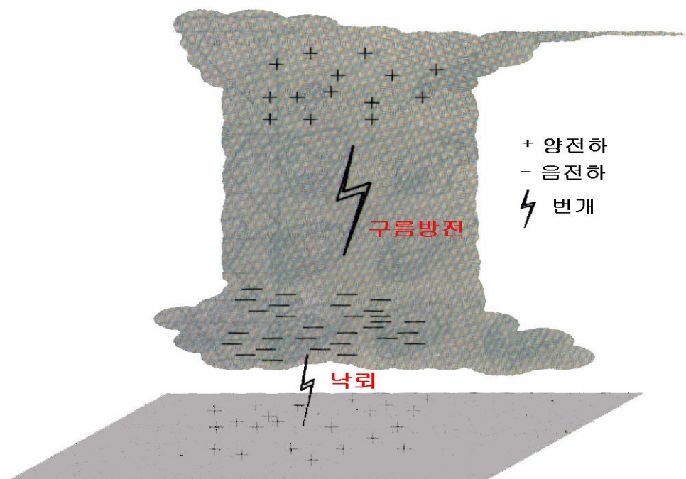
그림 3. 방전의 종류
