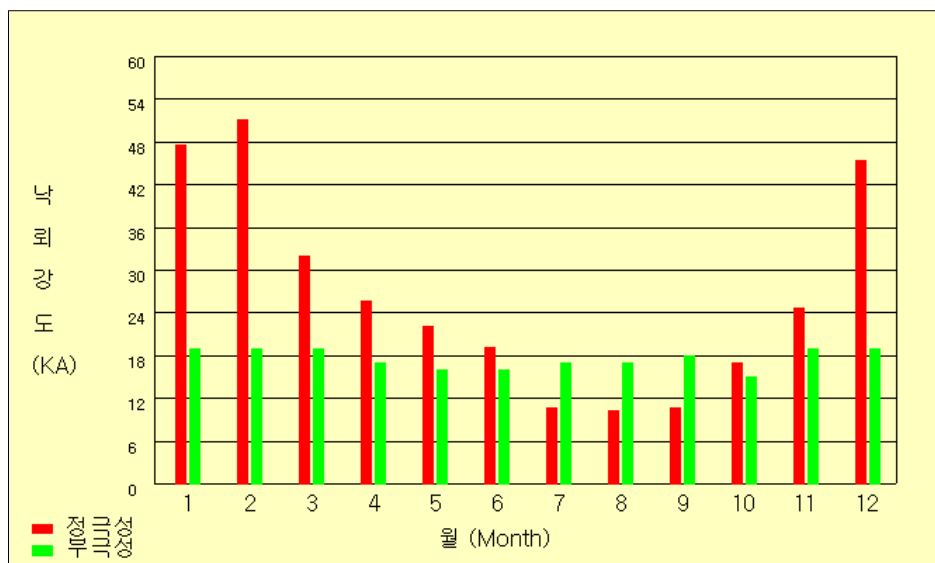
그림 48(a). 2003년 월별 평균 강도
