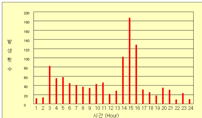
그림 31(b). 2007년 2월 시간별 낙뢰발생 횟수
