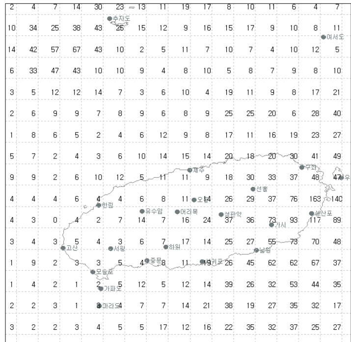
그림 29(e). 2007년 8월 제주도지역 낙뢰발생 횟수
