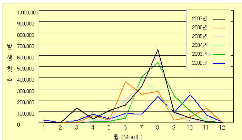
그림 53. 연도에 따른 월별 낙뢰발생 횟수
