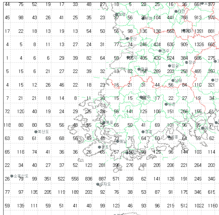
그림 28(c). 2007년 6월 전라도지역 낙뢰발생 횟수
