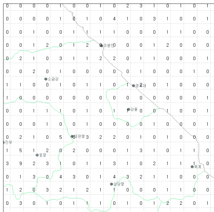
그림 23(b). 2007년 5월 강릉지역 낙뢰발생 횟수
