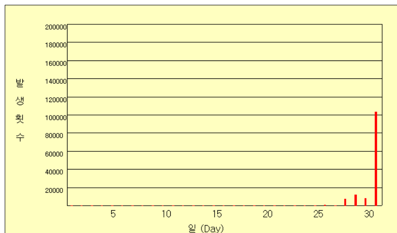
그림 32(a). 2007년 3월 일별 낙뢰발생 횟수
