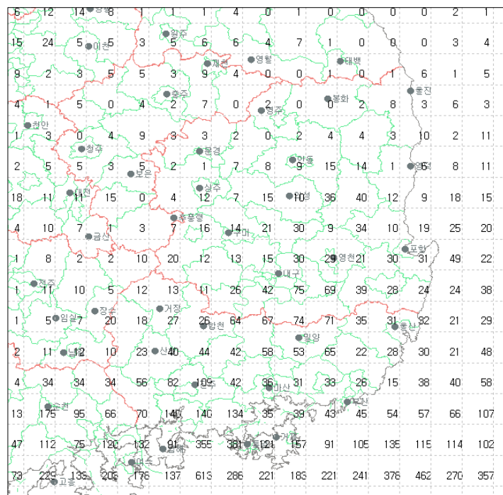
그림 27(f). 2007년 9월 경상도지역 낙뢰발생 횟수
