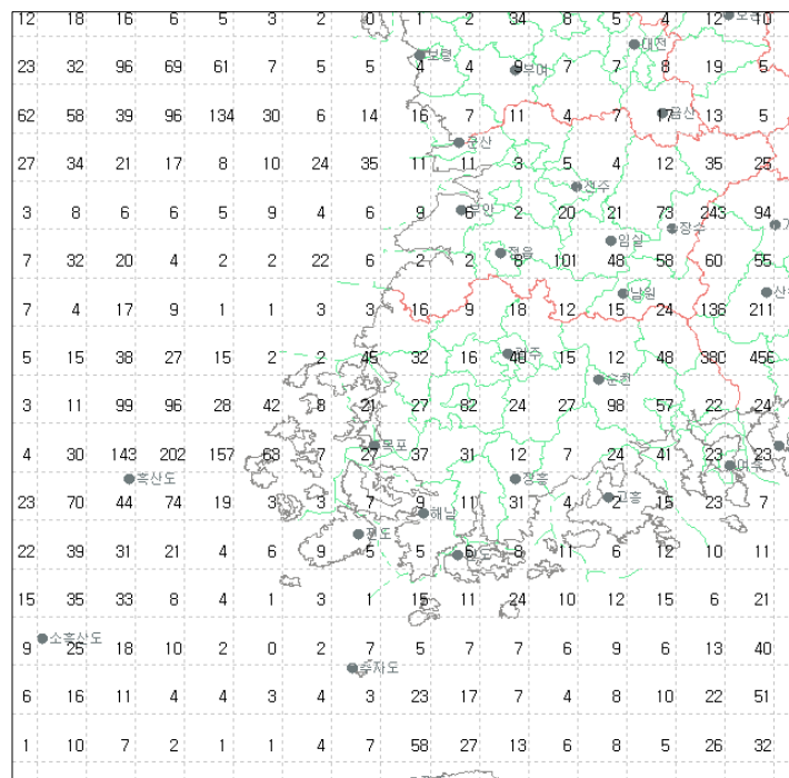
그림 28(b). 2007년 5월 전라도지역 낙뢰발생 횟수
