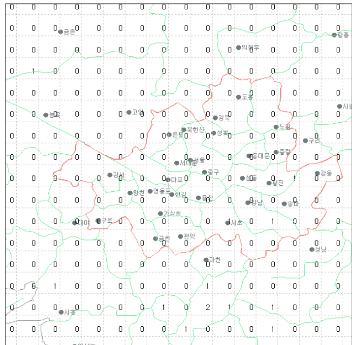
그림 18(a). 2007년 4월 서울지역 낙뢰발생 횟수
