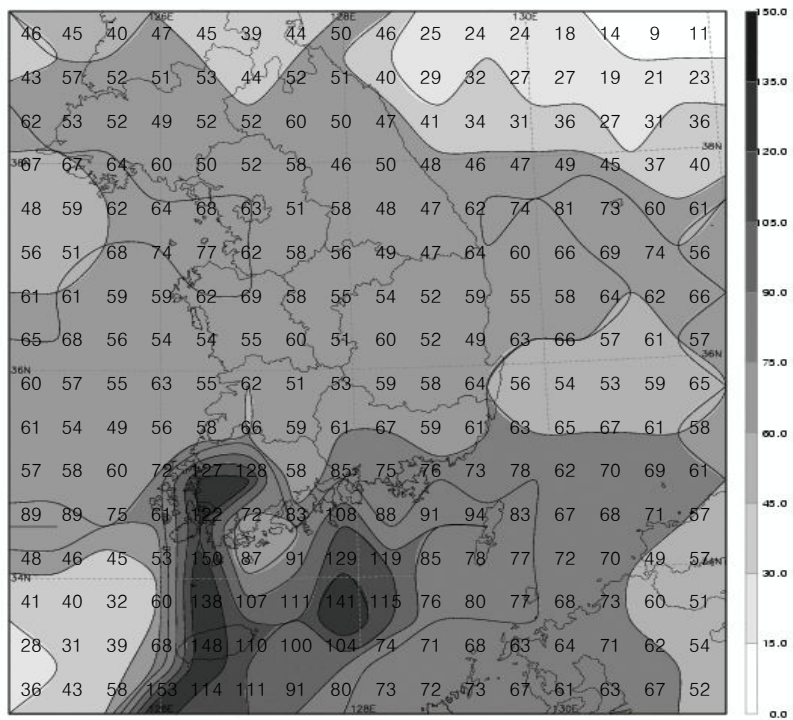
그림 17(b). 2007년 낙뢰발생 일수 분포도
