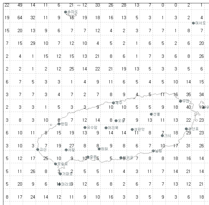
그림 29(d). 2007년 7월 제주도지역 낙뢰발생 횟수
