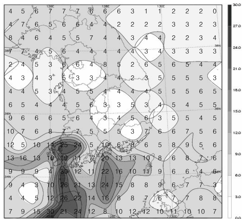
그림 6(b). 2007년 6월의 낙뢰발생 일수 분포도
