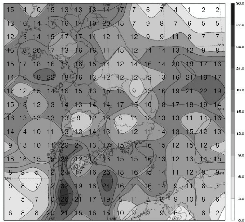
그림 13(b). 2007년 봄철의 낙뢰발생 일수 분포도
