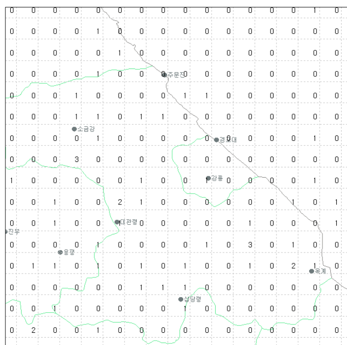
그림 23(a). 2007년 4월 강릉지역 낙뢰발생 횟수
