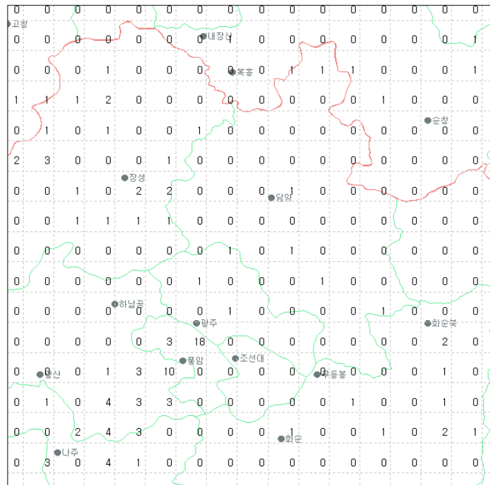
그림 21(c). 2007년 6월 광주지역 낙뢰발생 횟수
