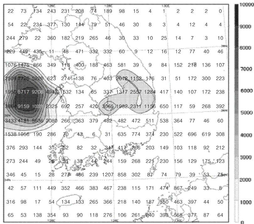
그림 6(a). 2007년 6월의 낙뢰발생 횟수 분포도
