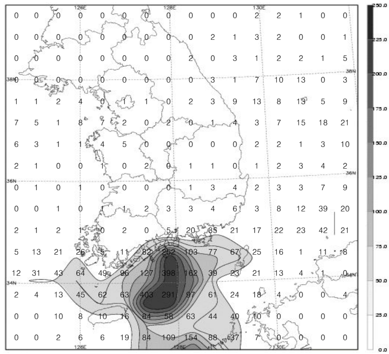
그림 12(a). 2007년 12월의 낙뢰발생 횟수 분포도
