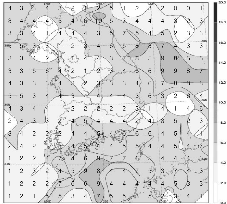
그림 4(b). 2007년 4월의 낙뢰발생 일수 분포도
