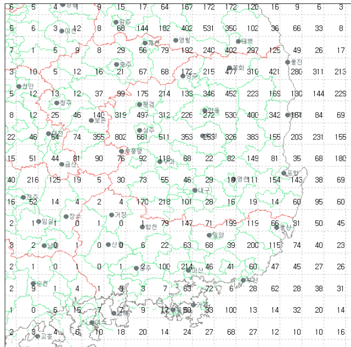
그림 27(c). 2007년 6월 경상도지역 낙뢰발생 횟수
