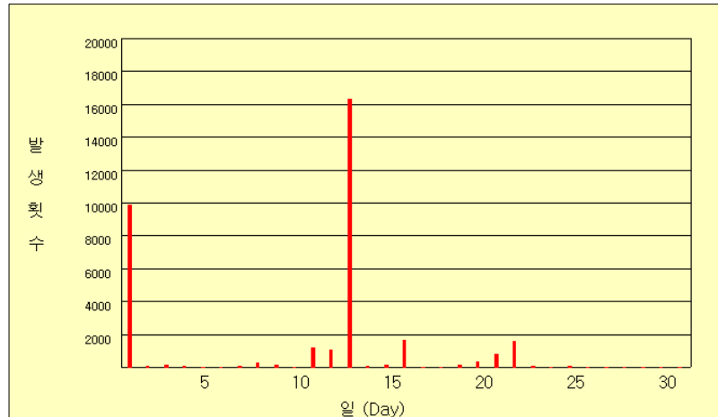
그림 33(a). 2007년 4월 일별 낙뢰발생 횟수
