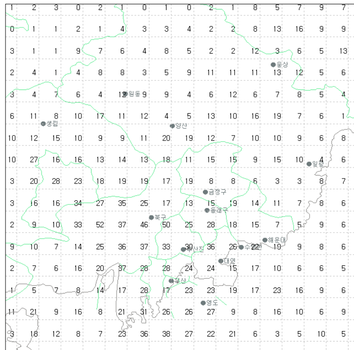
그림 19(d). 2007년 7월 부산지역 낙뢰발생 횟수
