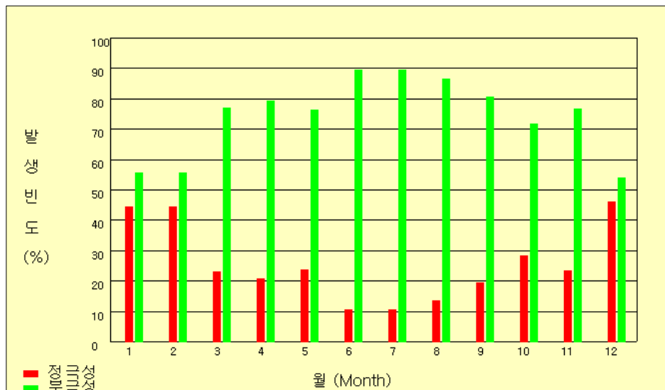
그림 49(c). 2005년 월별 극성율 빈도
