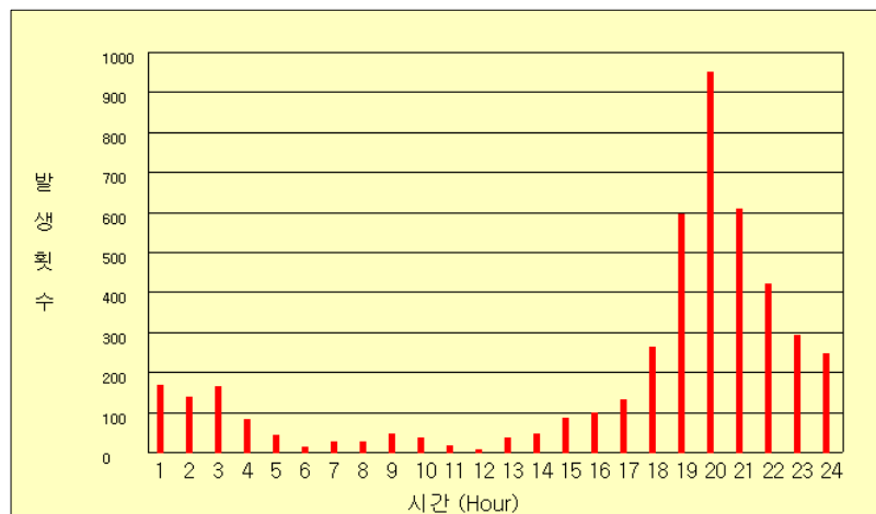
그림 41(b). 2007년 12월 시간별 낙뢰발생 횟수
