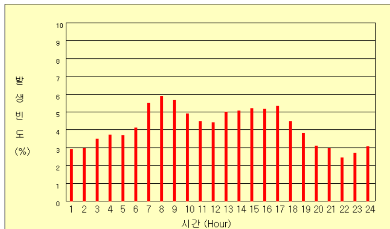
그림 46(j). 2007년 시간별 낙뢰발생 빈도
