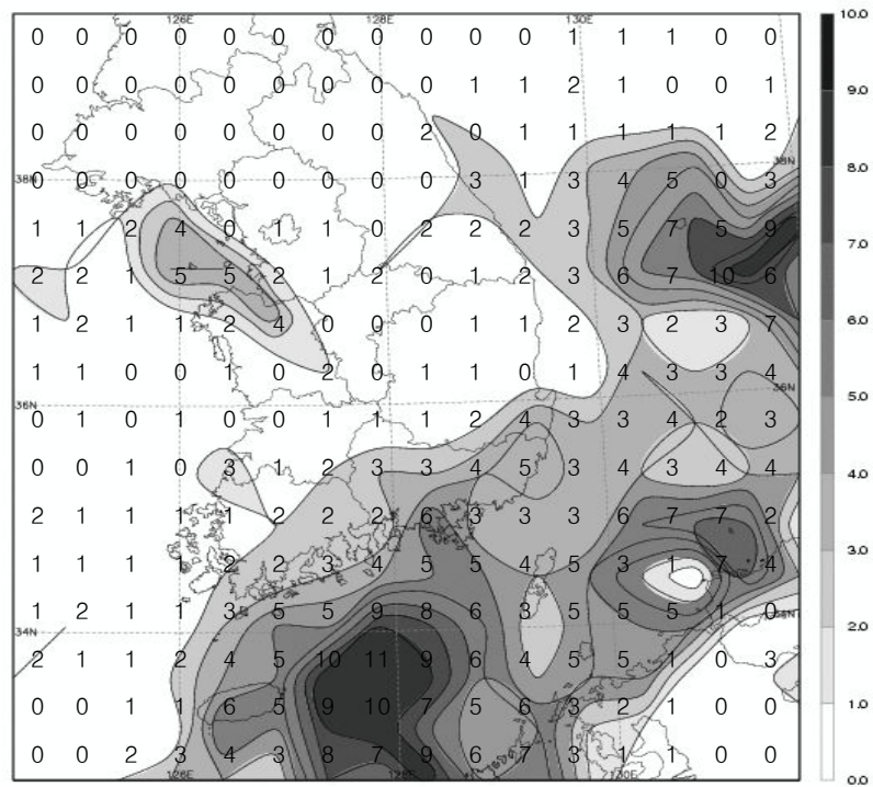
그림 16(b). 2007년 겨울철의 낙뢰발생 일수 분포도
