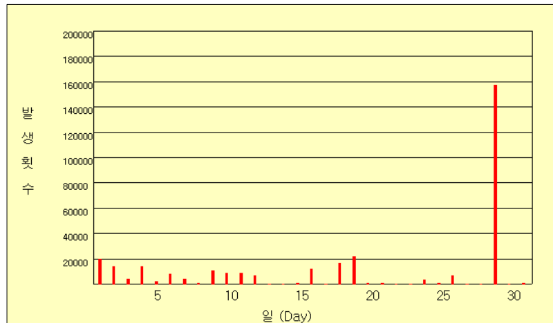
그림 36(a). 2007년 7월 일별 낙뢰발생 횟수
