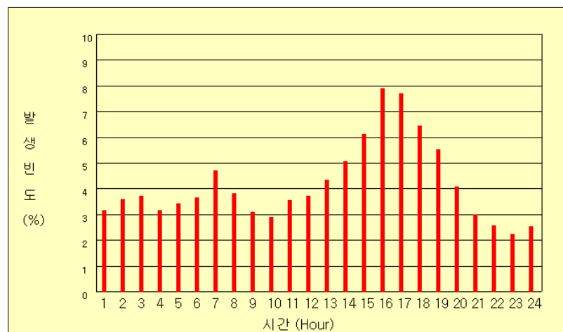
그림 46(h). 2006년 시간별 낙뢰발생 빈도
