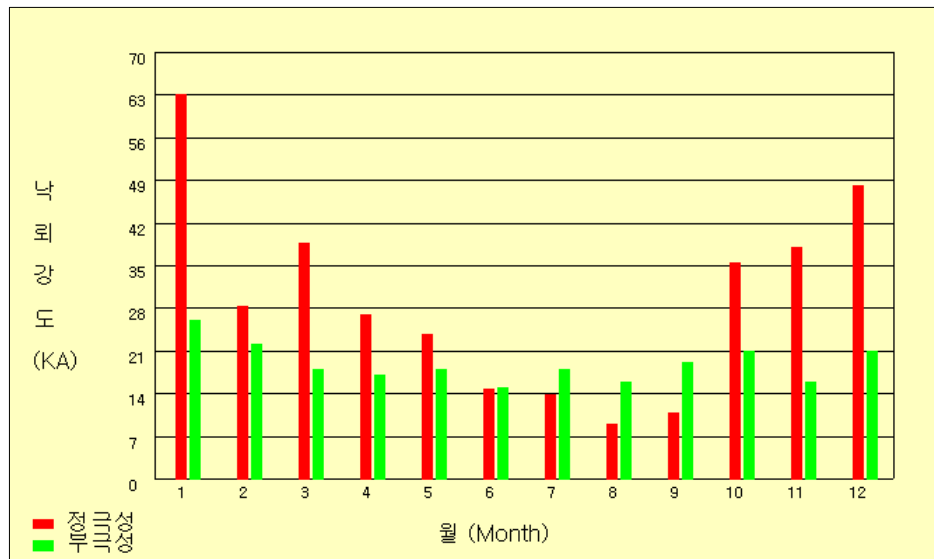
그림 48(c). 2005년 월별 평균 강도
