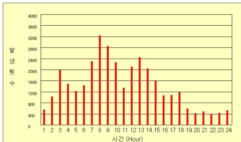
그림 33(b). 2007년 4월 시간별 낙뢰발생 횟수
