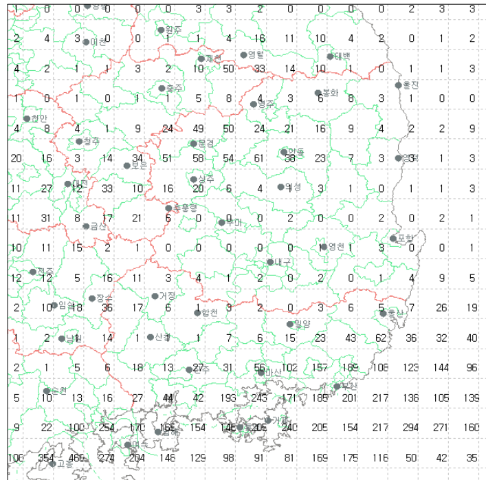
그림 27(a). 2007년 4월 경상도지역 낙뢰발생 횟수
