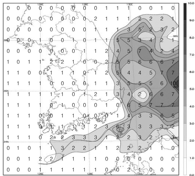
그림 1(b). 2007년 1월의 낙뢰발생 일수 분포도
