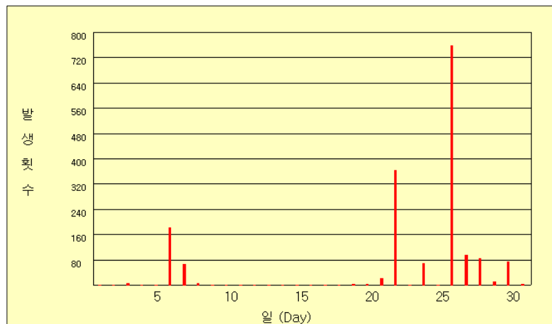
그림 30(a). 2007년 1월 일별 낙뢰발생 횟수
