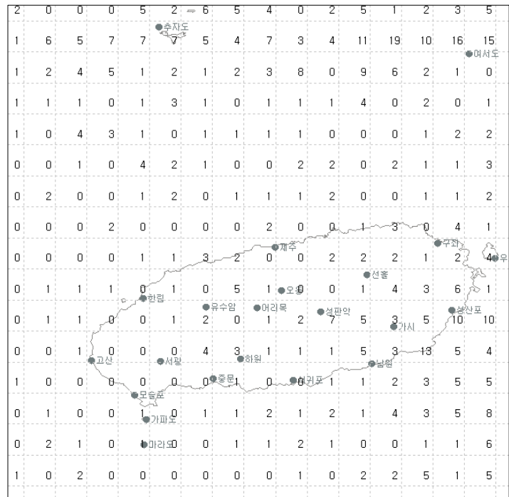
그림 29(a). 2007년 4월 제주도지역 낙뢰발생 횟수
