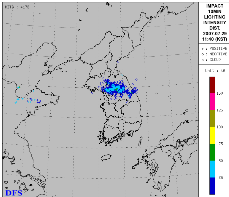
그림 16. 낙뢰영상
