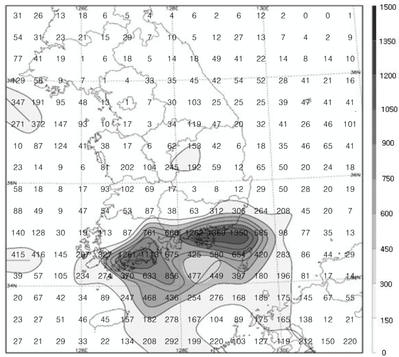
그림 4(a). 2007년 4월의 낙뢰발생 횟수 분포도
