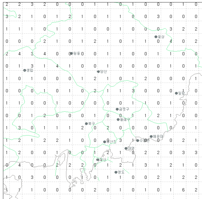
그림 19(f). 2007년 9월 부산지역 낙뢰발생 횟수
