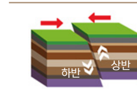
역단층
