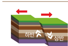
정단층
