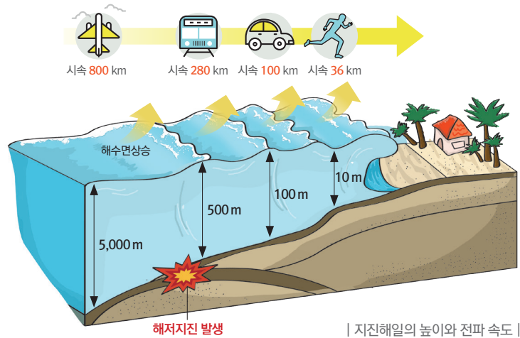
| 지진해일의 높이와 전파 속도 |
