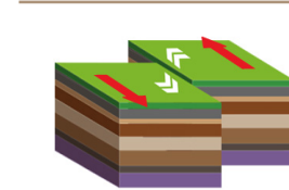
주향이동단층
