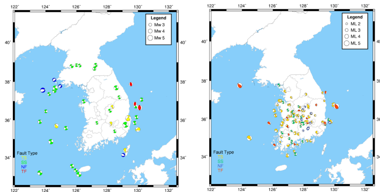
한반도 주요 지진의 단층면해
