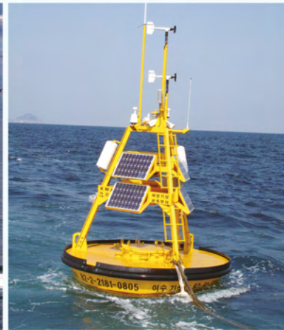
해양기상부이
