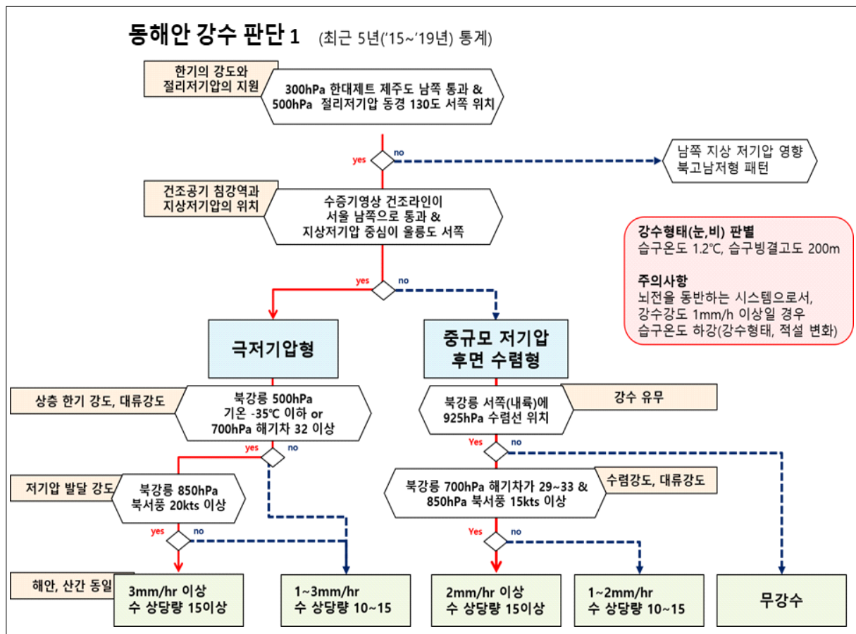
그림 4-25. ‘극저기압형(직접영향)’, ‘중규모저기압 후면 수렴형(간접영향)’ 강설 판단 흐름도
