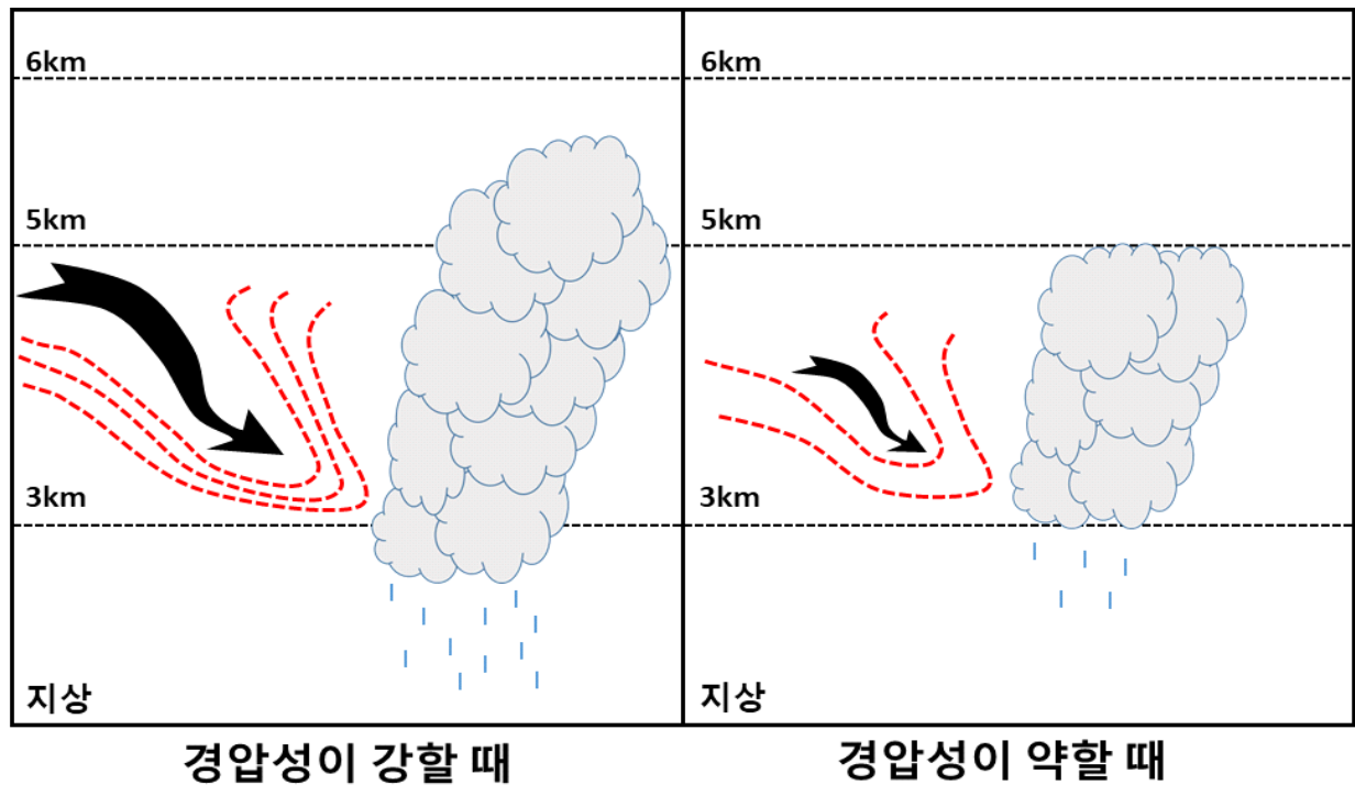
그림 5-15. 중층 경압성 강도에 따른 구름발달 모식도
