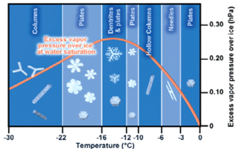
그림 3-10. 기온에 따른 얼음에 대한 수증기압 초과 값(hPa)과 눈 결정체 모양(출처: COMET) -22°C 이하의 낮은 기온에서는 큰 입자의 눈송이가 만들어지기 어려움
