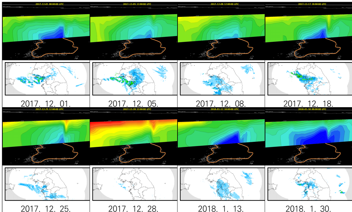
그림 1-25. 중부지방 연직단면도 온위(260~280K)
