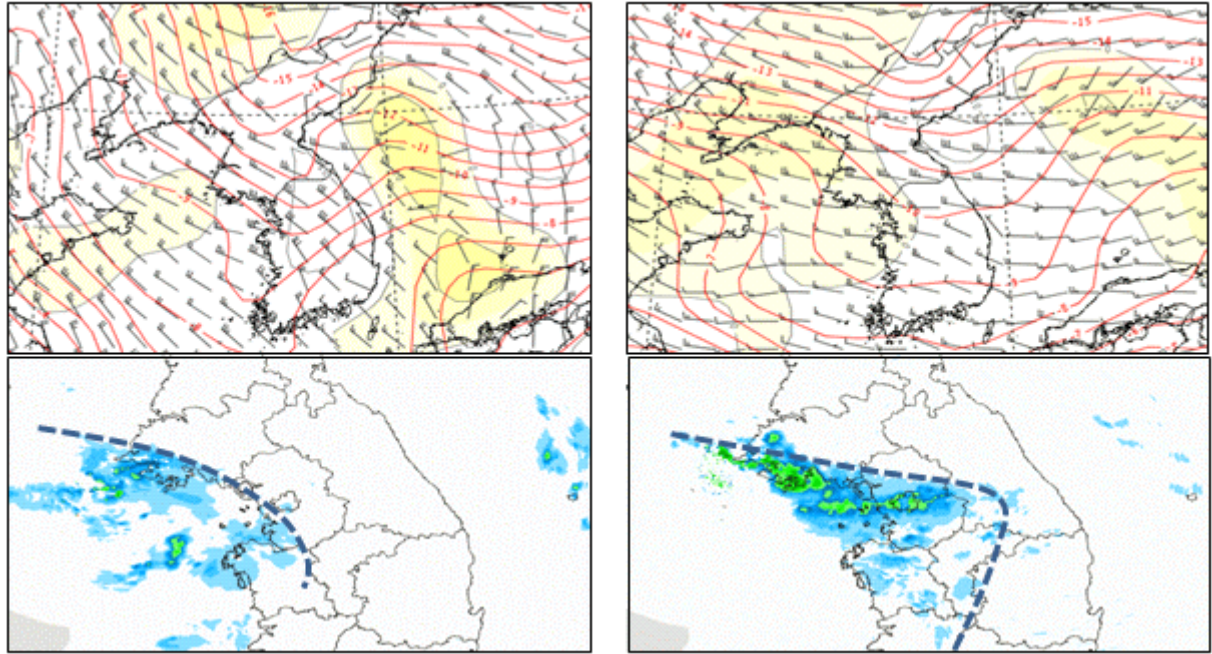
그림 1-14. 850hPa 기온, 바람, P속도, 레이더합성 (2017. 12. 8. 21시)
