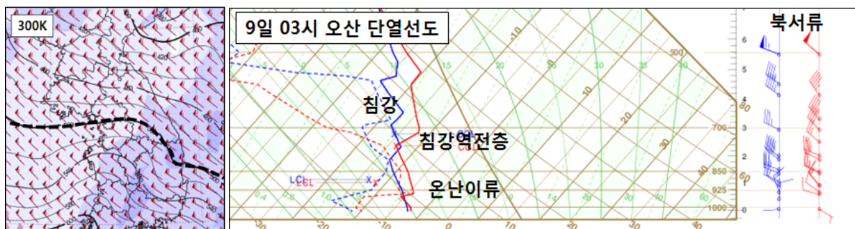
그림 1-21. 2017. 12. 9. 03시 (좌) 300K 등온위면, (우) 오산 단열선도 분석장
