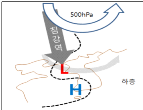
그림 1-17. 상층골 이동에 따른 침강역 모식도
