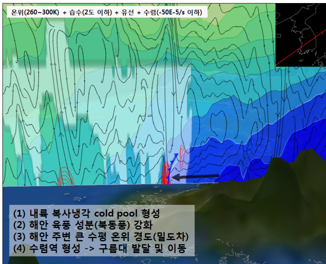
그림 3-32. 2018년 1월 24일 09시 UM국지모델 분석장의 Gloview를 이용한 온위(푸른색~연두색), 습수(투명한 흰색), 유선(검은색), 수렴 변수(붉은 실선)의 연직단면 분석
