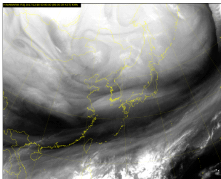
그림 2-1. 발해만 저기압이 발달할 때의 수증기 영상 (2017.12.18. 09시 히마와리 수증기 영상 (6.2 \mu m))
