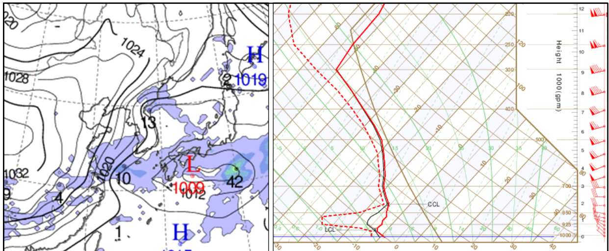
그림 5-16. 2019년 12월 24일 21시 모델이 예측한 2019년 12월 26일 12시 UM 예상일기도 (좌) 해면기압/누적강수량 예상, (우) 서울 단열선도
