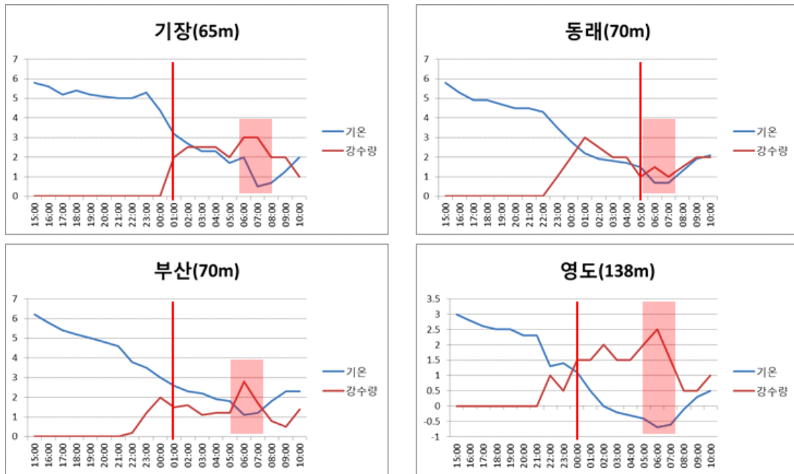
그림 6-11. 부산 주요지점별 2018년 3월 20일 15시~21일 10시까지 매 시각 기온, 강수량 분포도 (붉은색 수직선: 강수가 시작되는 시점으로서, 상대습도 90% 이상을 나타내기 시작한 시각, 붉은색 사각형 구간: 강수가 증가된 시각)
