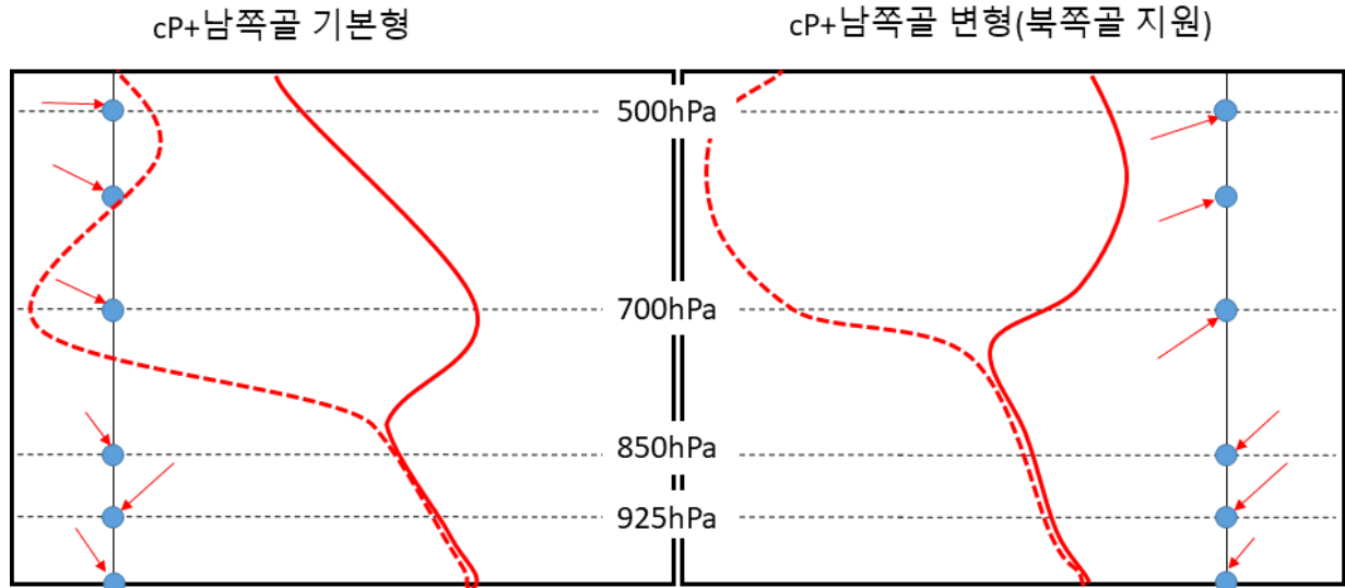
그림 4-34. 'cP확장+남쪽저기압형' 열역학선도 모식도 기본형(좌) 북쪽골이 동반되는 유형(우)
