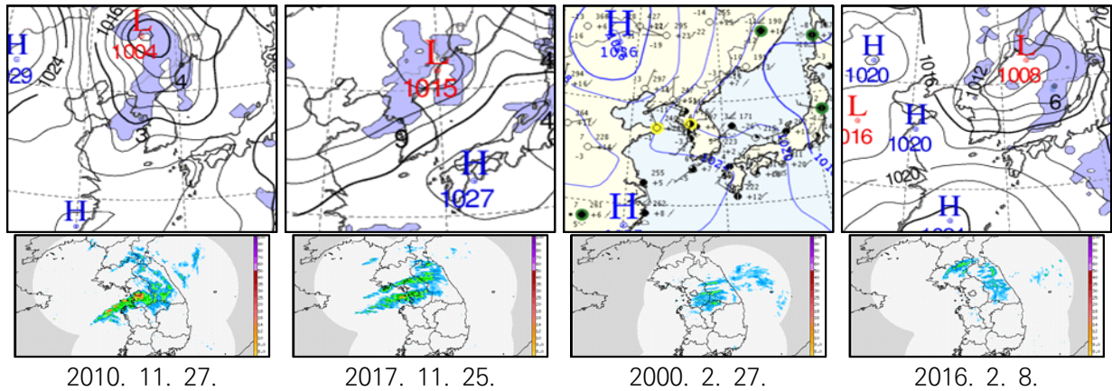
그림 1-5. 지상일기도(상), 레이더 PPI0 실태(하)
