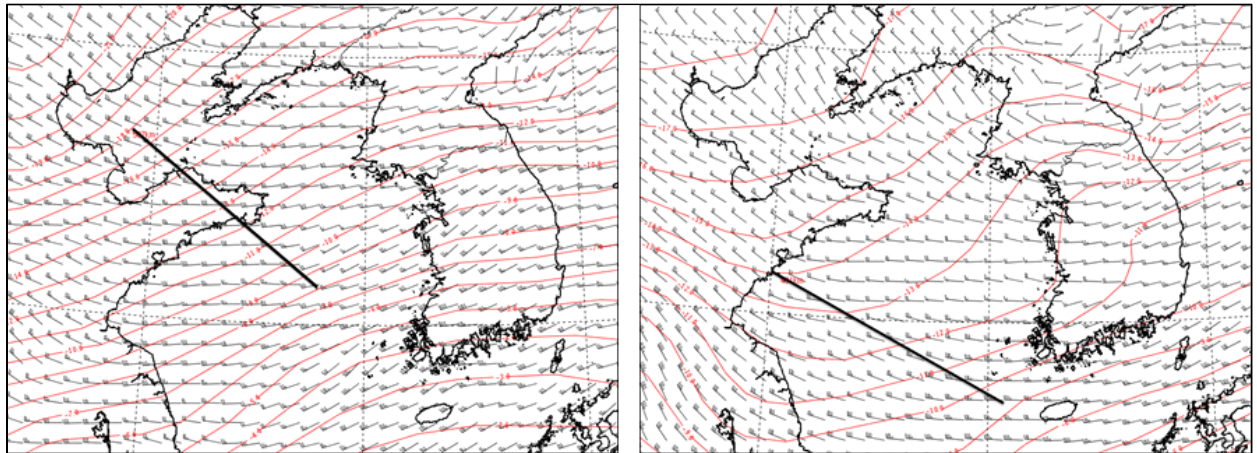
그림 5-13. 700hPa의 바람과 등온선/왼쪽 2019년 12월 26일 09시, 오른쪽 2020년 1월 12일 03시
