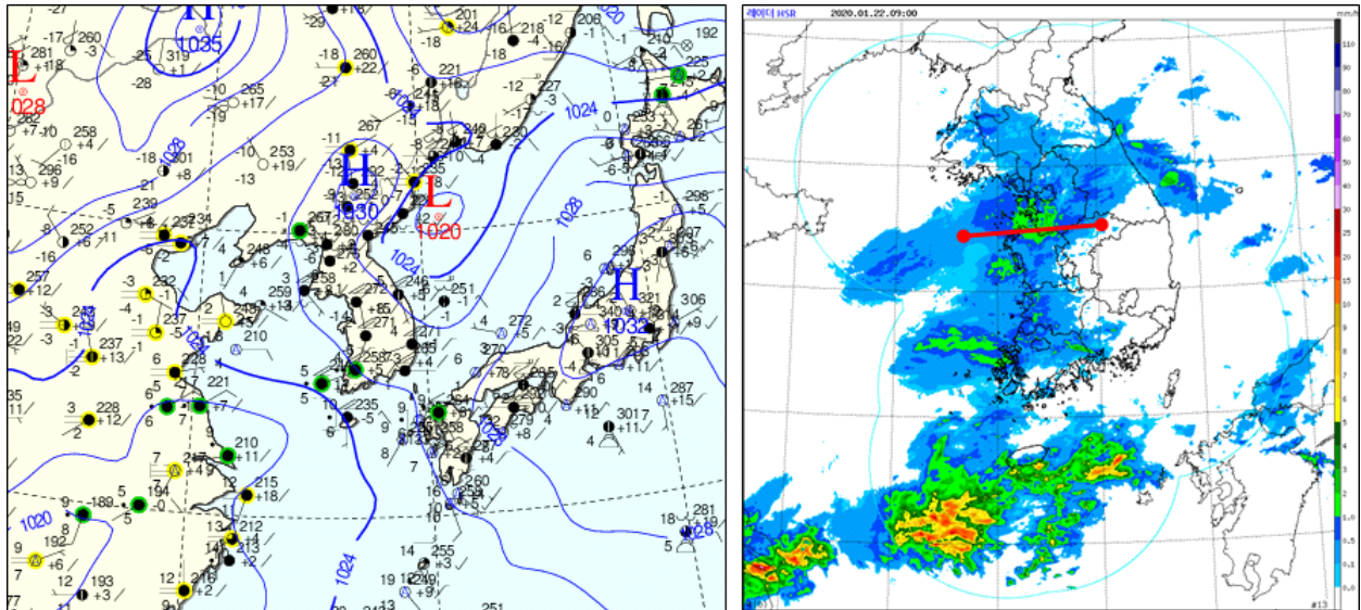
그림 5-10. 2020년 1월 22일 09시 지상일기도와 레이더합성영상(HSR)
