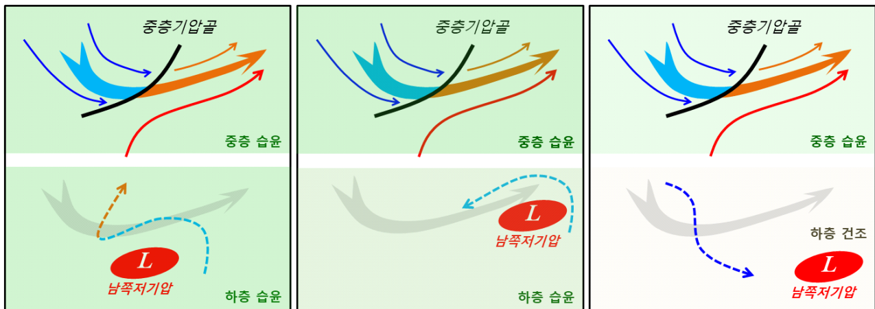
그림 5-5. 남쪽저기압 북상 정도에 따른 중층기압골과 연관성 (파란 점선: 하층기류, 빨간 점선: 상층기류)
