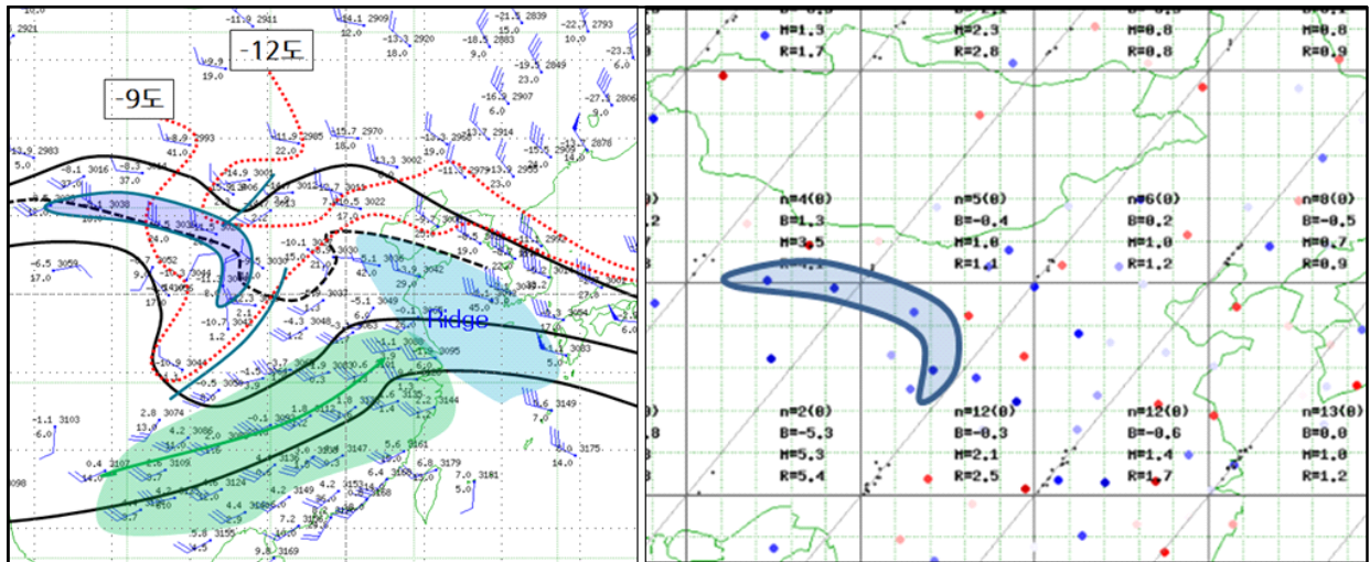
그림 5-18. 2019년 1월 10일 21시 700hPa GTS일기도(좌), UM모델(분석장) 풍속 편차(우)
