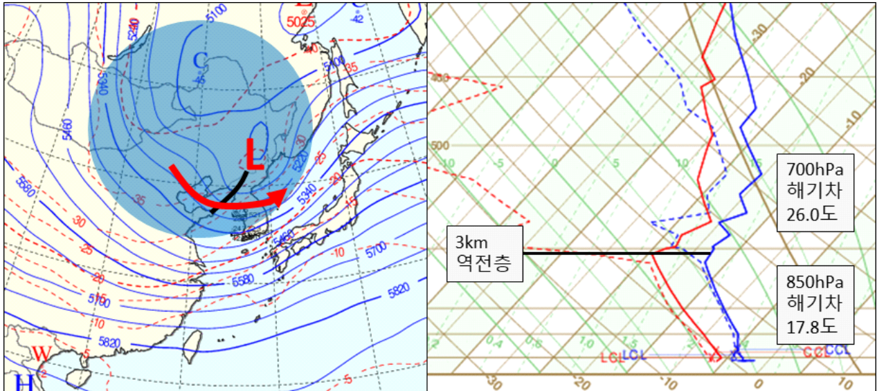
그림 3-23. 2018년 1월 9일 03시 500hPa 일기도와 광주 단열선도
