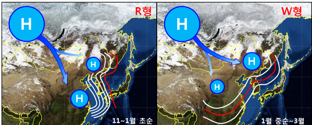
그림 4-3. 기후학적인 겨울철 대륙고기압 확장경로와 해면기압 형태
