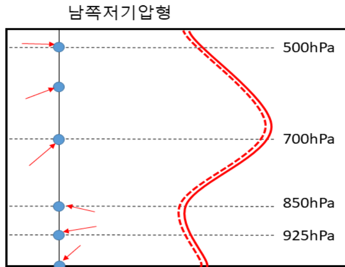
그림 4-35. '남쪽저기압형' 열역학선도 모식도
