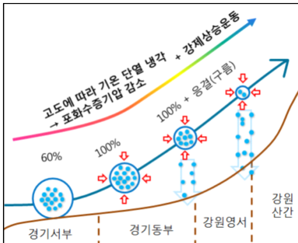
그림 1-22. 산간지역 강제상승에 의한 강수 모식도
