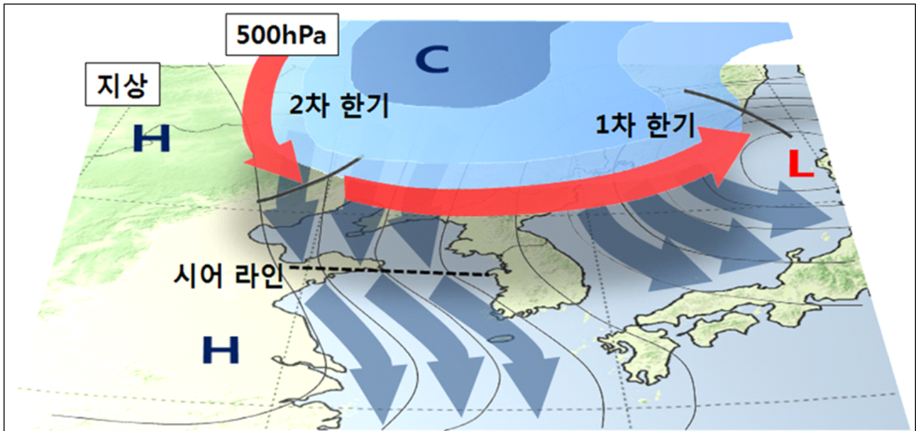
그림 3-26. 상층 기압골 영향으로 서해상에 기류 수렴이 형성되는 기압계의 모식도
