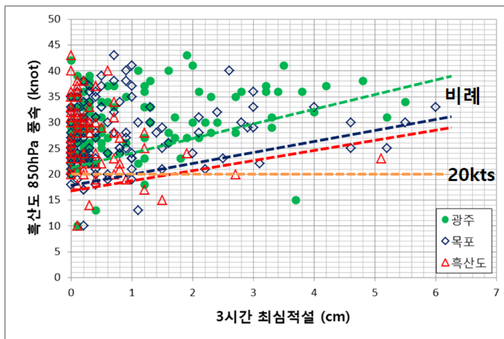
그림 3-11. 2003~2017년 겨울철(11월~2월) 호수 효과에 의한 서해안 강설 사례 중 흑산도 850hPa 풍속과 광주, 목포, 흑산도의 3시간 최심적설 분포 20kts 이상에서 대부분 적설이 나타나며, 강한 강도에는 강한 풍속이 필요함
