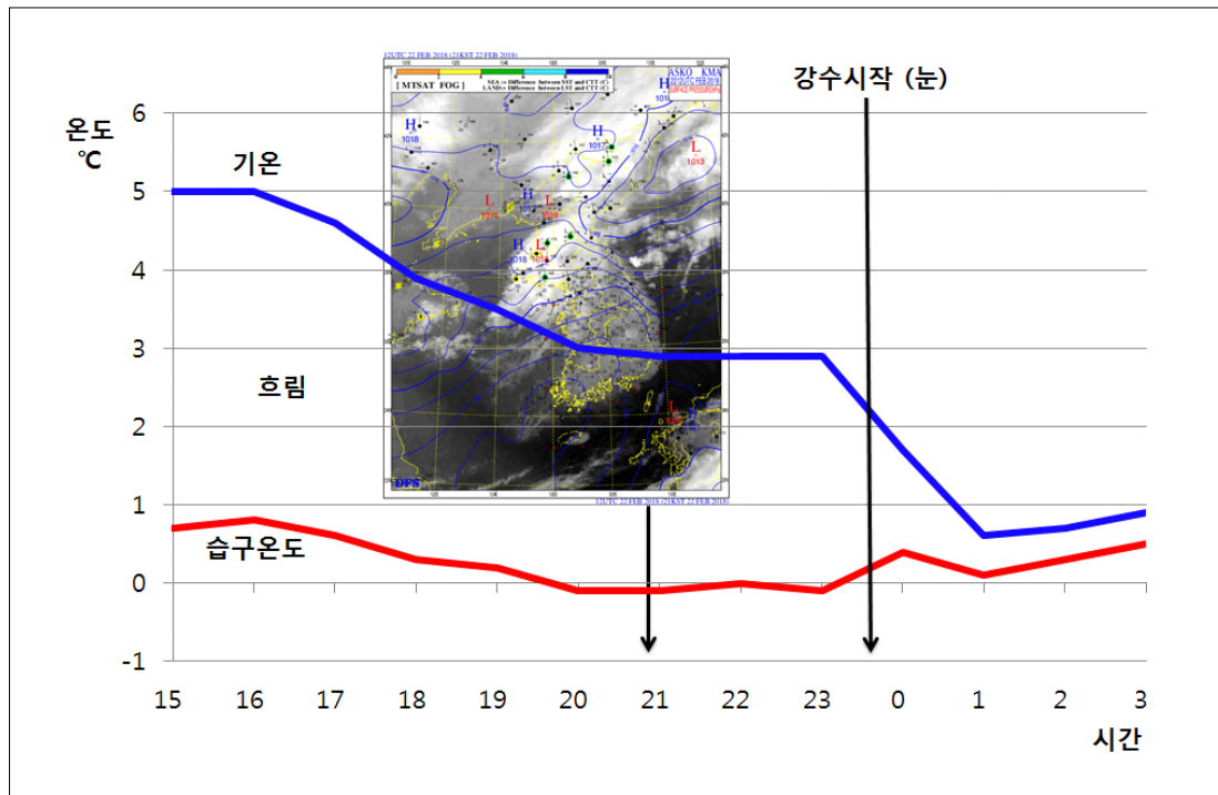
그림 6-4. 구름이 끼고 비(눈)이 내린 날씨의 기온과 습구온도 변화 (2018년 2월 22일 15시에서 23일 03시까지의 서울의 기온과 습구온도)
