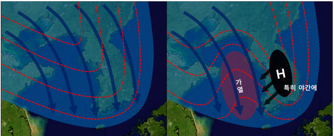
그림 3-29. 서해안형 강설이 발생할 때 전반(왼쪽)과 후반(오른쪽)의 지상 또는 하층의 모식도. 전반에는 서해상과 한반도로 강하게 한기가 남하, 시간이 지나면 해상은 따뜻해지고 내륙은 냉각되면서 온도구조가 달라짐.
