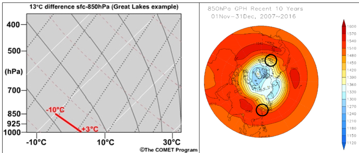
그림 3-3. (좌) 미국 오대호 지역에서 호수 효과 강설에 필요한 850hPa 해기차와 열역학선도 예시 건조단열감률 이상의 기울기가 필요함을 알 수 있음
