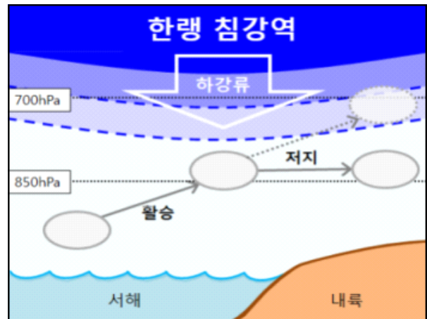
그림 1-18. 하강류에 의한 구름 발달 제한 모식도
