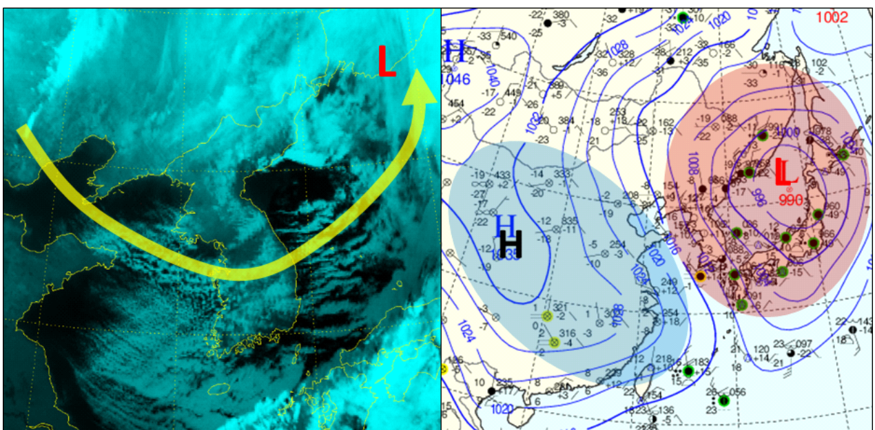
그림 3-22. 2018년 1월 9일 03시 천리안위성 합성영상과 지상일기도
