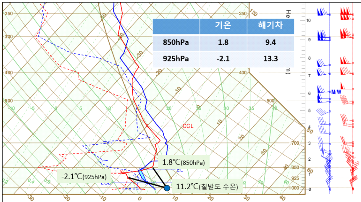
그림 3-8. 2019년 12월 18일 09시 흑산도 단열선도
