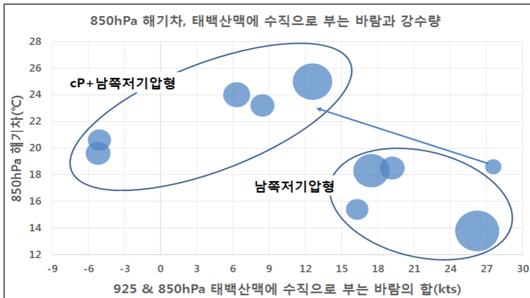
그림 4-27. 850hPa 해기차와 태백산맥(330도 방향)에 수직으로 부는 두 고도(925hPa, 850hPa) 바람의 합과 강수량(동심원의 크기)
