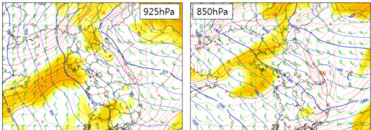
그림 2-7. 2019. 1. 15. 09시 925hpa(좌) 850hpa(우) 일기도
