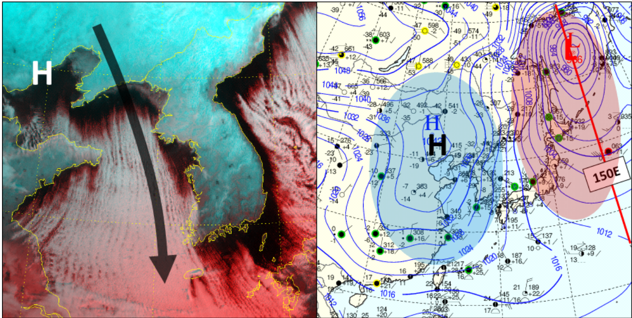
그림 3-20. 2018년 1월 26일 09시 천리안위성 합성영상과 지상일기도
