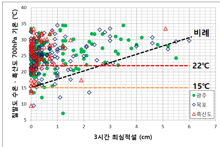
그림 3-6. 2003~2017년 겨울철(11월~2월) 호수 효과에 의한 서해안 강설 사례 중 칠발도-흑산도 700hPa 해기차와 광주, 목포, 흑산도의 3시간 최심적설 분포 15℃ 이상에서 대부분 적설이 나타나며, 22℃ 이상에서 3cm/3hr 강도의 적설이 발생 해기차가 작아질수록 강한 강도의 적설이 나타나기 어려움
