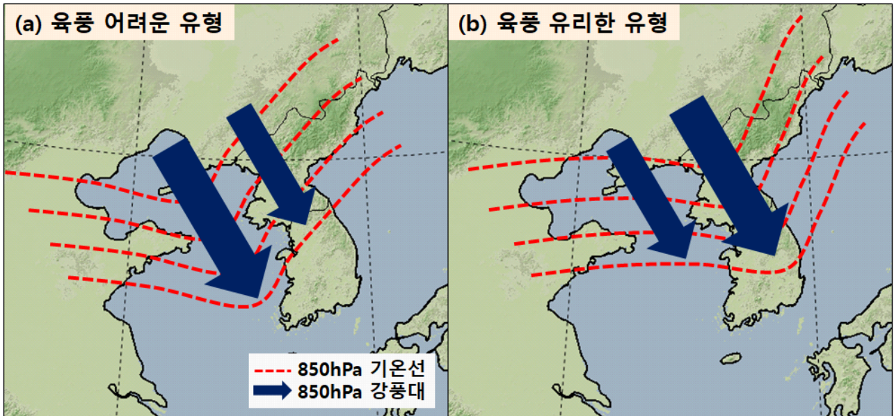
그림 3-31. 850hPa 등온선분포와 강풍대 위치에 따른 육풍이 어려운 유형(a), 유리한 유형(b)
