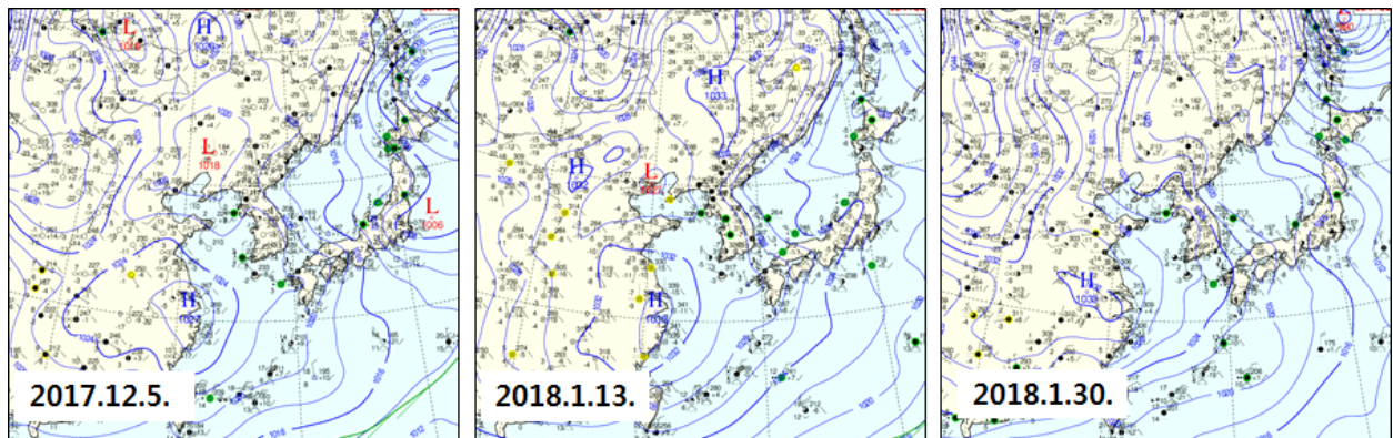
그림 2-2. 수도권 지역 5cm 내외의 적설을 기록한 사례의 지상 일기도
