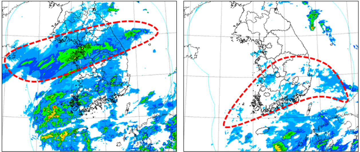
그림 5-14. 레이더합성영상(HSR) / 왼쪽 2019년 12월 26일 09시, 오른쪽 2020년 1월 12일 03시 (빨간색 점선: 중층기압골에 의한 강수대에 해당)
