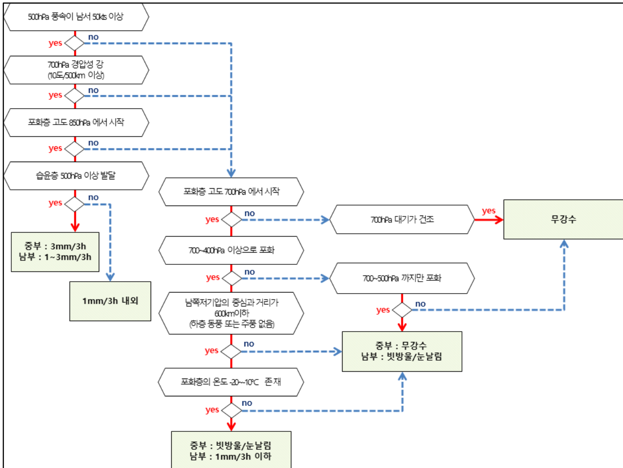
그림 5-23. 중층기압골에 의한 강수 예보 흐름도
