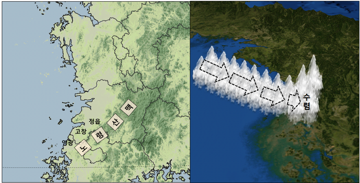
그림 3-27. 노령산맥 풍상측의 영광, 고창 정읍의 위치와 지형 수렴에 의한 구름대 발달 모식도
