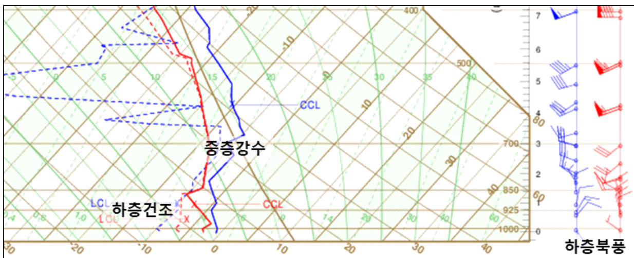
그림 5-1. 2019. 12. 26. 09시 오산 단열선도 (중층강수 사례)
