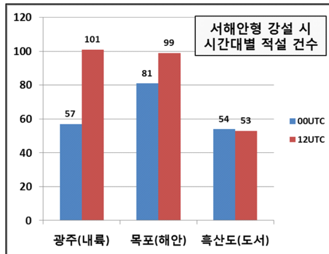
그림 3-33. 2008~2012년 겨울철(11월~2월) 시간대별(00/12UTC) 서해안형 강설의 지점별 적설 일수, 내륙인 광주 지점은 육풍 효과가 강한 00UTC 시간대에 적설 빈도가 절반으로 줄어듦
