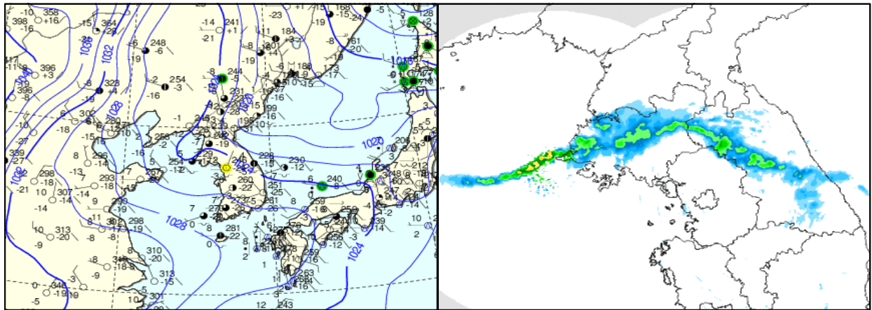
그림 2-3. 발해만 기압골이 동반된 온난이류형 강수 (2017. 12. 18. 15시)
