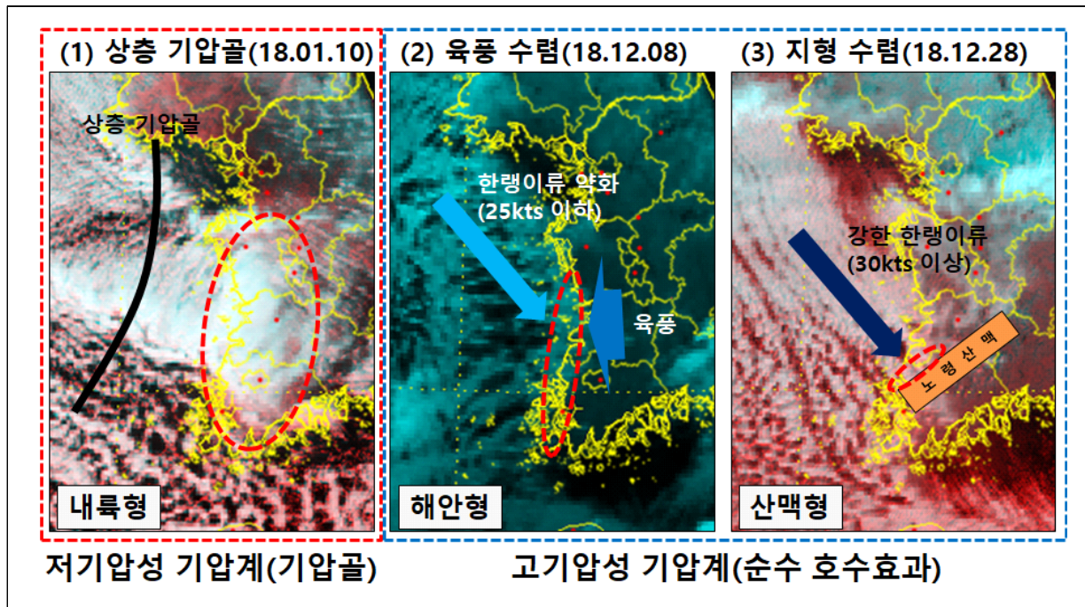
그림 3-24. 서해안형 강설 중 10cm 이상 대설이 가능한 세 가지, 상층 기압골 영향을 받는 저기압성 기압계(기압골) (1)내륙형, (2)해안형, (3)산맥형
