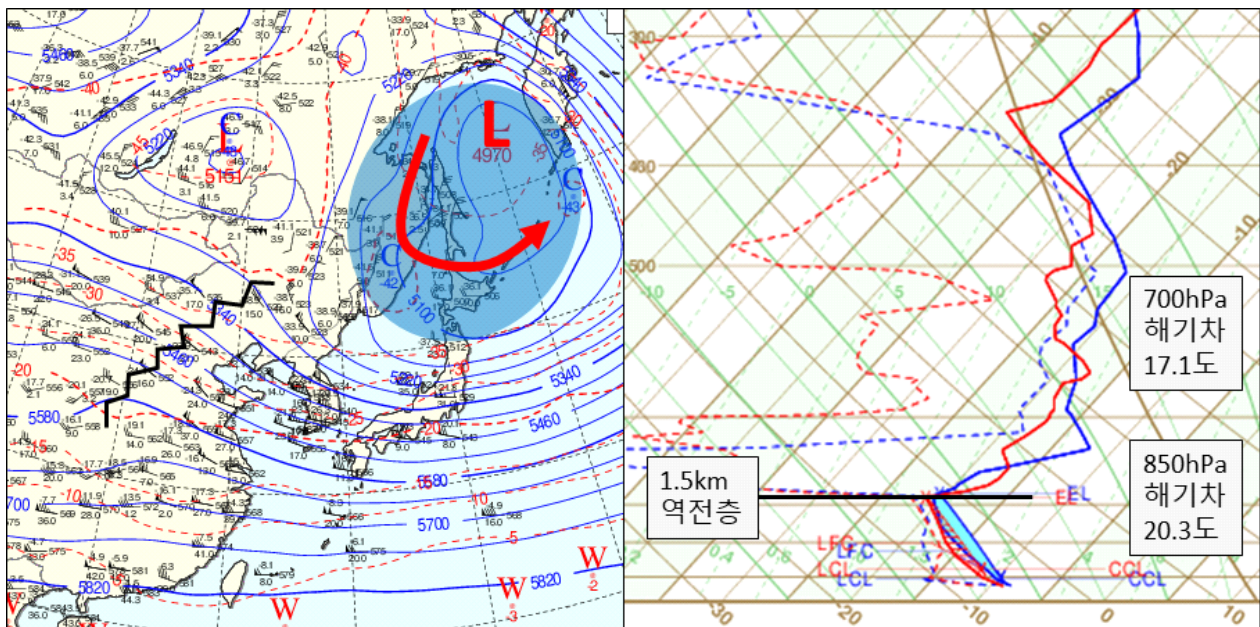
그림 3-21. 2018년 1월 26일 09시 500hPa 일기도와 흑산도 단열선도
