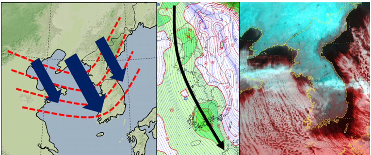
그림 3-28. 지형 수렴형 대설에 유리한 하층 강풍축과 등온선 모식도 (2018년 12월 28일 850hPa 유선장과 위성 합성영상) 강풍축과 온도골이 서해안으로 집중되면서 노령산맥 풍상측에 지형 수렴이 강해질 수 있는 상황
