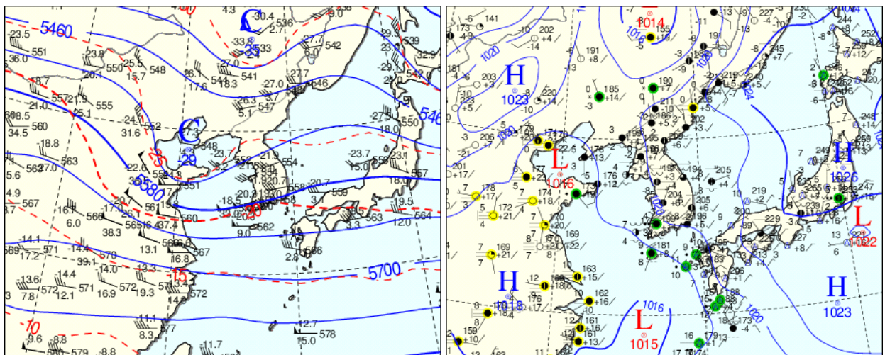
그림 5-20. 2020년 3월 7일 09시 500hPa 일기도(좌), 지상일기도(우)
