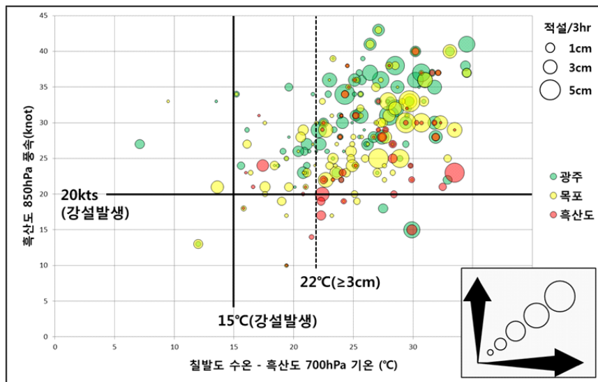
그림 3-18. 700hPa 해기차와 바람 통합 차트
