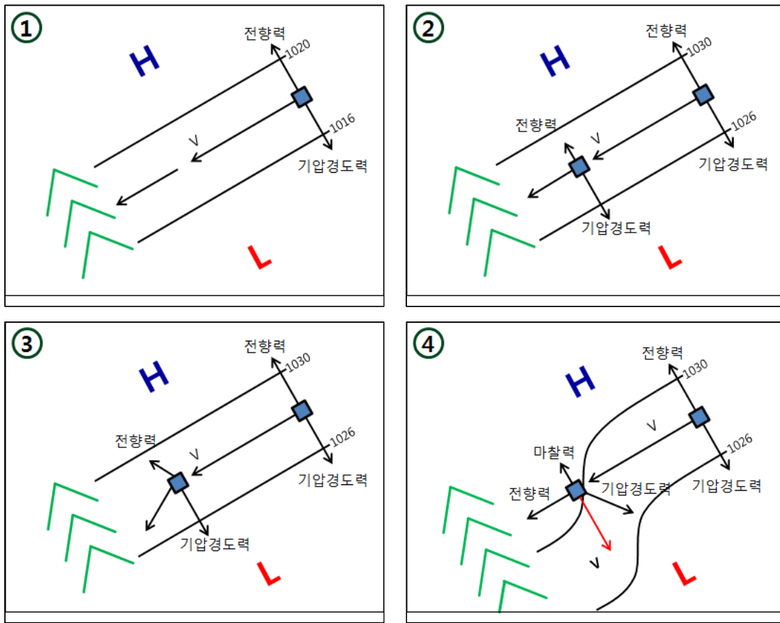
그림 4-16. 태백산맥 동쪽 사면으로 찬 공기가 쌓이는 기본적인 역학
