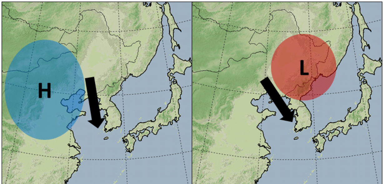
그림 3-19. 서해상에 강한 북풍 계열 기류로 한기를 남하시키는 대표적인 두 지상 기압계 왼쪽은 고기압의 전면, 오른쪽은 저기압의 후면을 따라 한기가 유입
