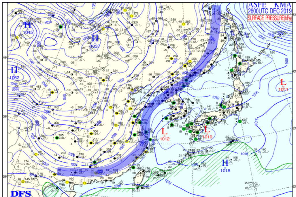
그림 5-2. 2019. 12. 26. 09시 3시간 지상일기도와 대륙고기압의 경계(파란색 선)
