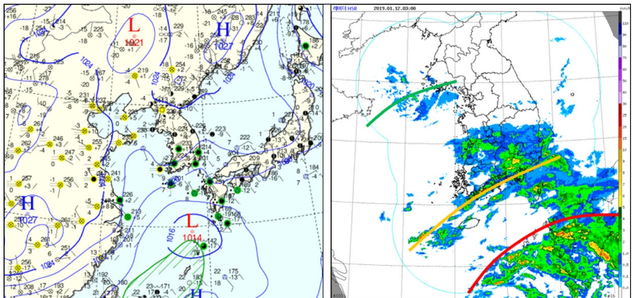
그림 5-6. 2019년 1월 12일 03시 지상일기도와 레이더합성영상(HSR)
