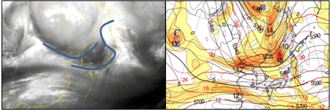
그림 2-6. 2019. 1. 15. 09시 수증기영상(좌), 500hPa 일기도(우) (파란선: Dry line)
