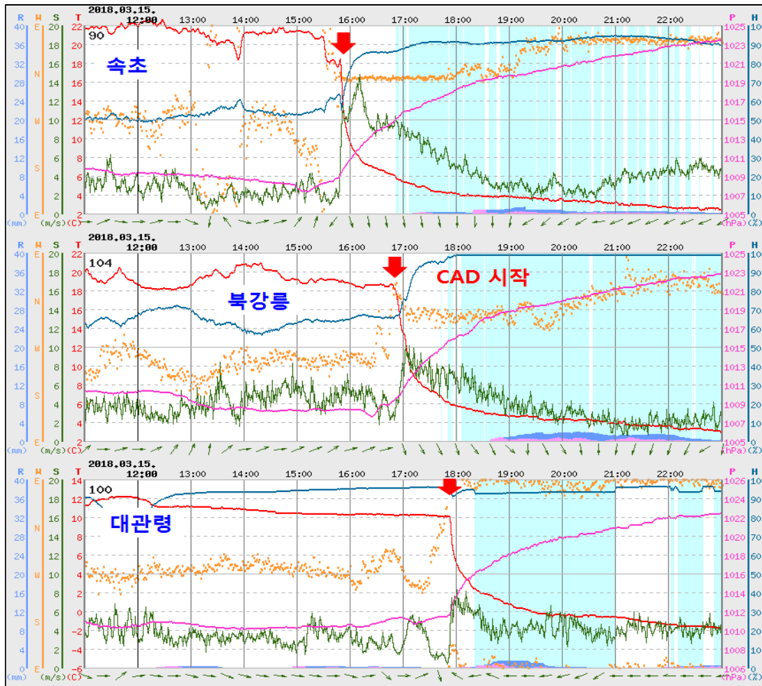
그림 4-18. 속초, 북강릉, 대관령 AWS 시계열
