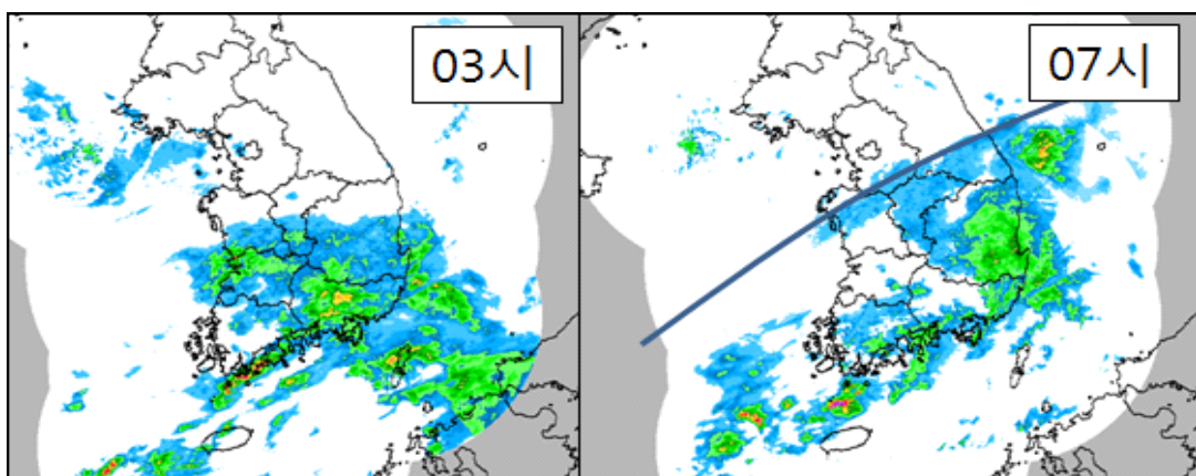
그림 5-19. 2019년 1월 12일 레이더 합성영상(HSR) (좌) 03시 관측, (우) 07시 관측 (실선: 지상 강수가 관측된 경계)
