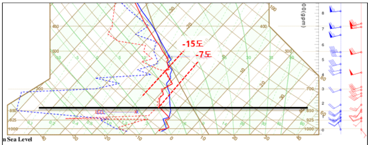
그림 5-11. 2020년 1월 22일 09시 오산 단열선도
