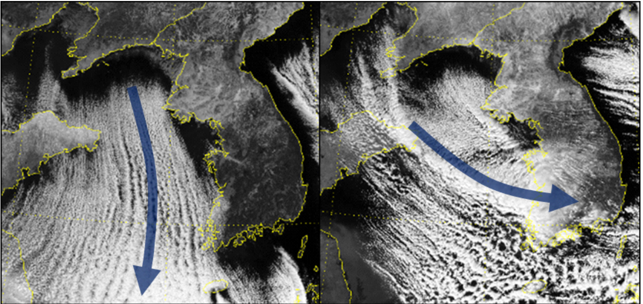
그림 3-25. 천리안 위성 가시영상 (좌) 2018년 1월 26일 12시, (우) 2018년 1월 10일 13시 왼쪽은 고기압성 회전, 오른쪽은 저기압성 회전으로 나타남
