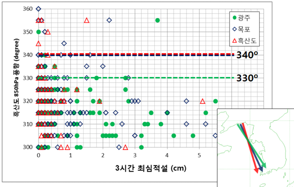
그림 3-13. 2003~2017년 겨울철(11월~2월) 호수 효과에 의한 서해안형 강설 사례 중 흑산도 850hPa 풍향과 광주, 목포, 흑산도의 3시간 최심적설 분포(점선은 90%이상 빈도를 보인 풍향)와 지점별 풍향에 따른 구름대 유입 경로 예시
