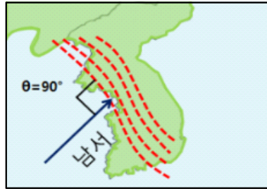
그림 1-9. 온도이류 모식도(서풍) 그림 1-10. 온도이류 모식도(남서) 그림 1-11. 온도이류 모식도(북서)
