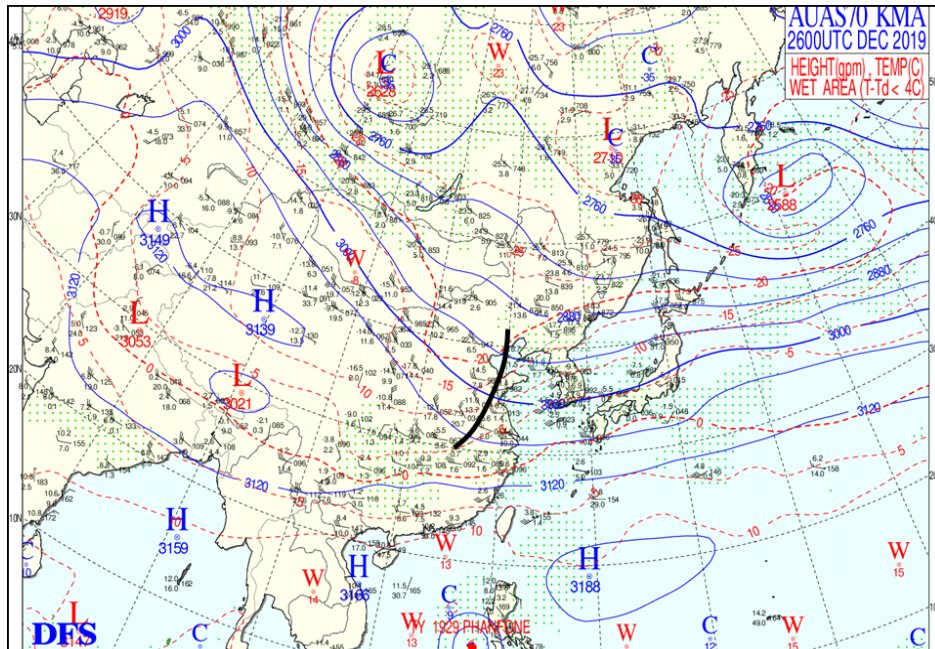
그림 5-3. 2019. 12. 26. 09시 700hPa 일기도와 기압골(검은색)
