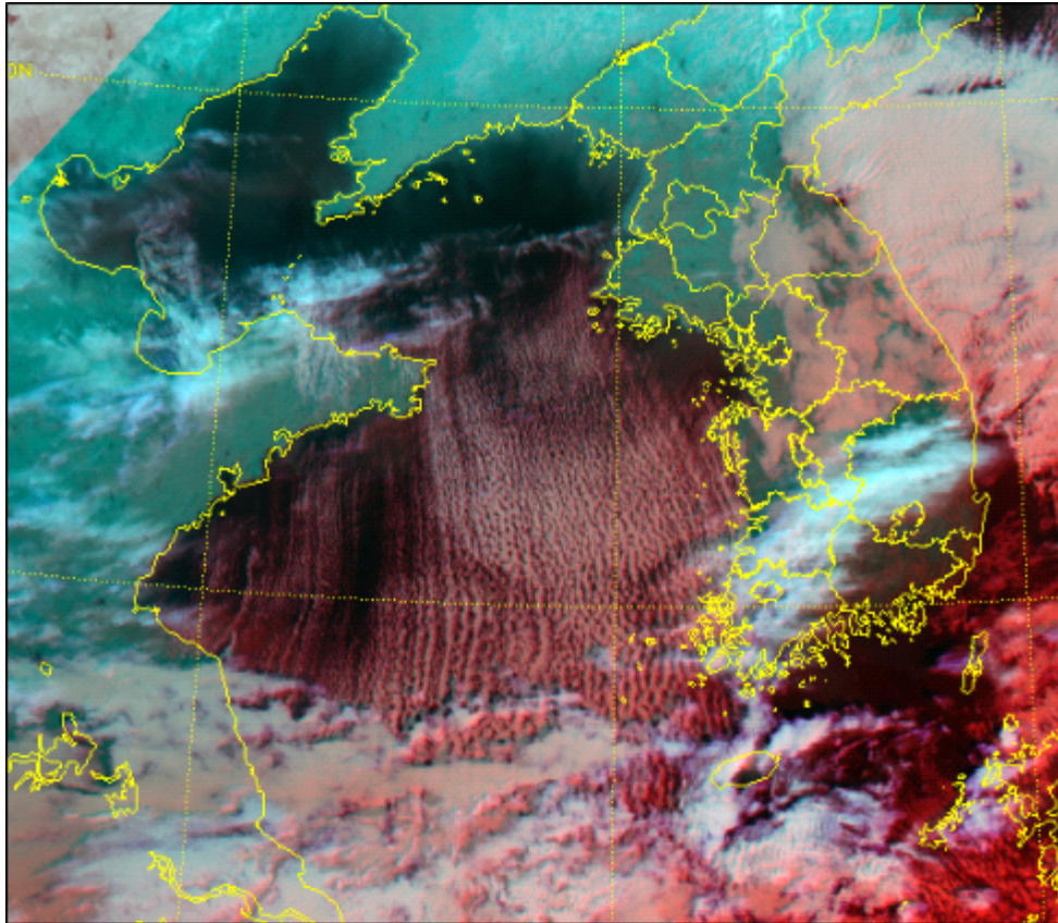
그림 3-7. 2019년 12월 18일 09시 천리안위성2A 합성영상 서해상에 해기차에 의한 대류운열이 뚜렷하게 발달한 모습
