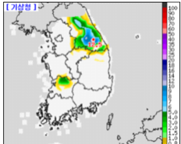
그림 1-23. 2016. 2. 8. 신적설 분포(온난이류 사례)
