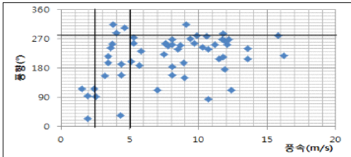
그림 1-16. 서울지역 적설 시 UM지역모델의 925hPa 풍향·풍속(2011~2016년)
