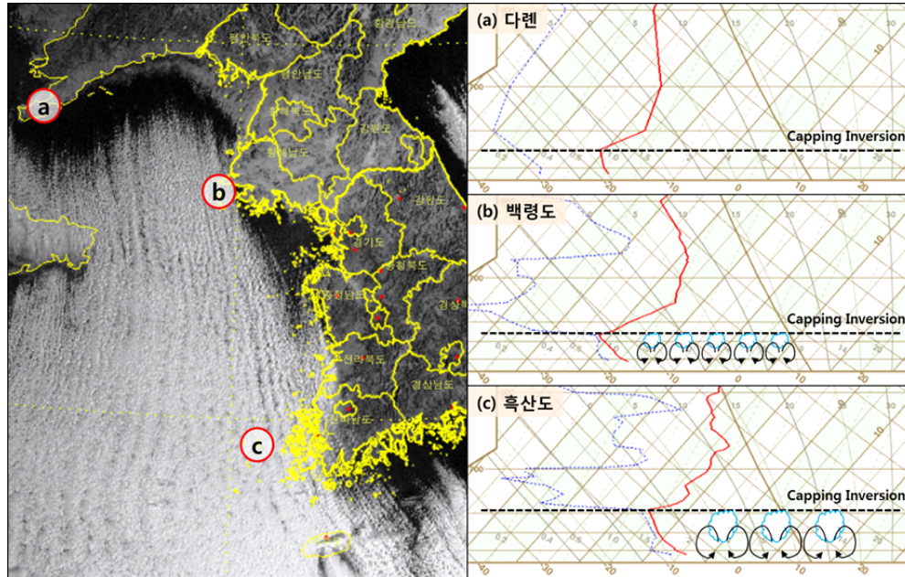
그림 3-15. (좌) 2018년 1월 26일 09시 천리안위성 가시영상 (우) 다렌(a), 백령도(b), 흑산도(c)의 GTS 고층자료 현황 (capping inversion(착모역전) 고도에 따른 대류 순환 규모 예시), 취주거리가 길어질수록 대류가 깊어져 구름열의 깊이와 폭도 증가함을 알 수 있음
