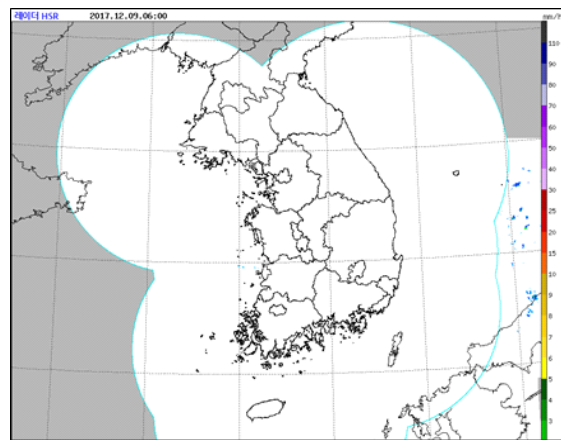
그림 1-20. 레이더 합성영상 (2017. 12. 9. 06시)
