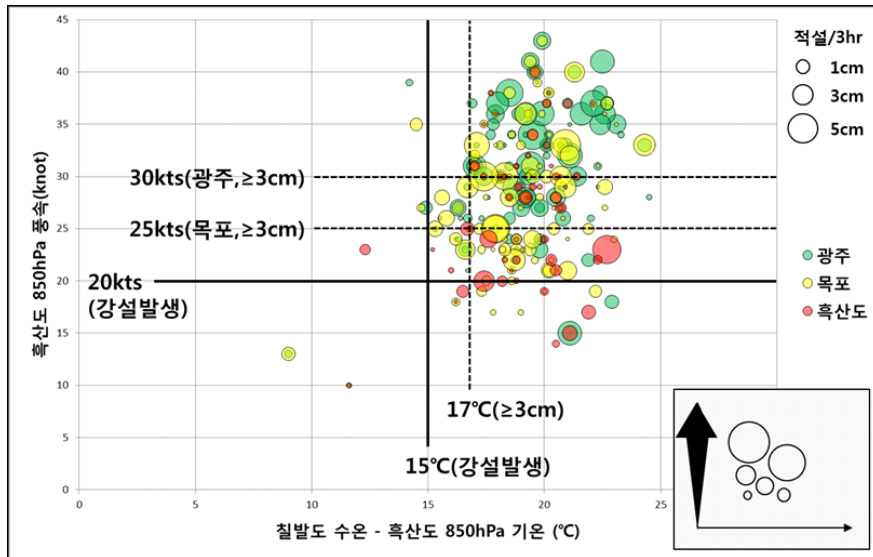
그림 3-17. 850hPa 해기차와 바람 통합 차트
