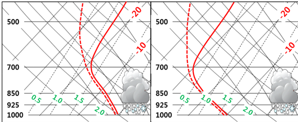
그림 3-9. 같은 두께로 발달한 구름이지만 기온의 연직 분포가 다른 두 경우 혼합비가 높은 왼쪽이 더 많은 수증기를 포함할 수 있어 많은 강수에 유리
