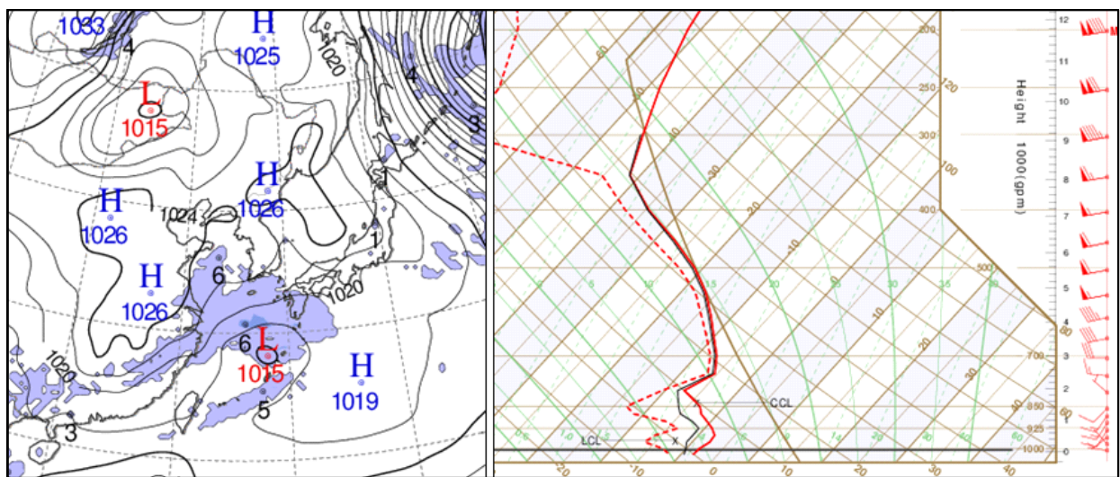
그림 5-17. 2019년 1월 10일 21시 모델이 예측한 2019년 1월 12일 03시 UM 예상일기도
