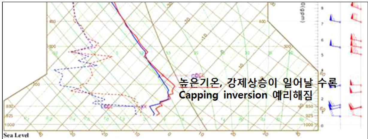
그림 1-24. 대관령 단열선도(2018. 2. 14. 09시)
