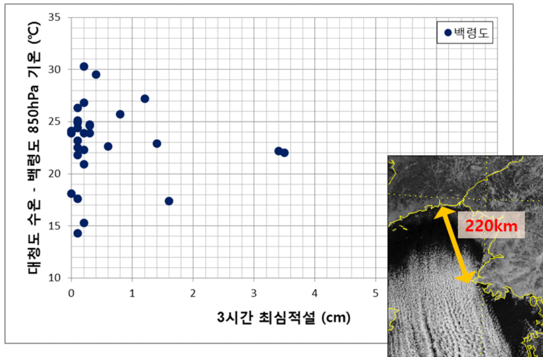
그림 3-16. 2008~2012년 겨울철(11월~2월) 호수 효과에 의한 서해안형 강설 사례 중 백령도 850hPa 해기차와 3시간 최심적설 분포 취주거리가 충분하지 않아 대부분 1cm 미만의 적설만 기록됨
