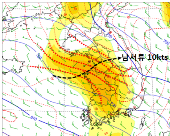
그림 1-19. 925hPa 상세바람장 (2017. 12. 9. 06시)
