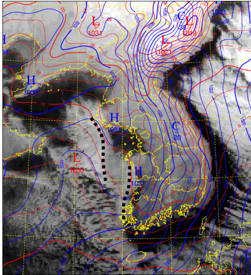
그림 3-30. 2018년 1월 24일 09시 한반도 기압(청색)/온위(적색) 분석장+적외영상과 수렴대(검정 점선) 표현
