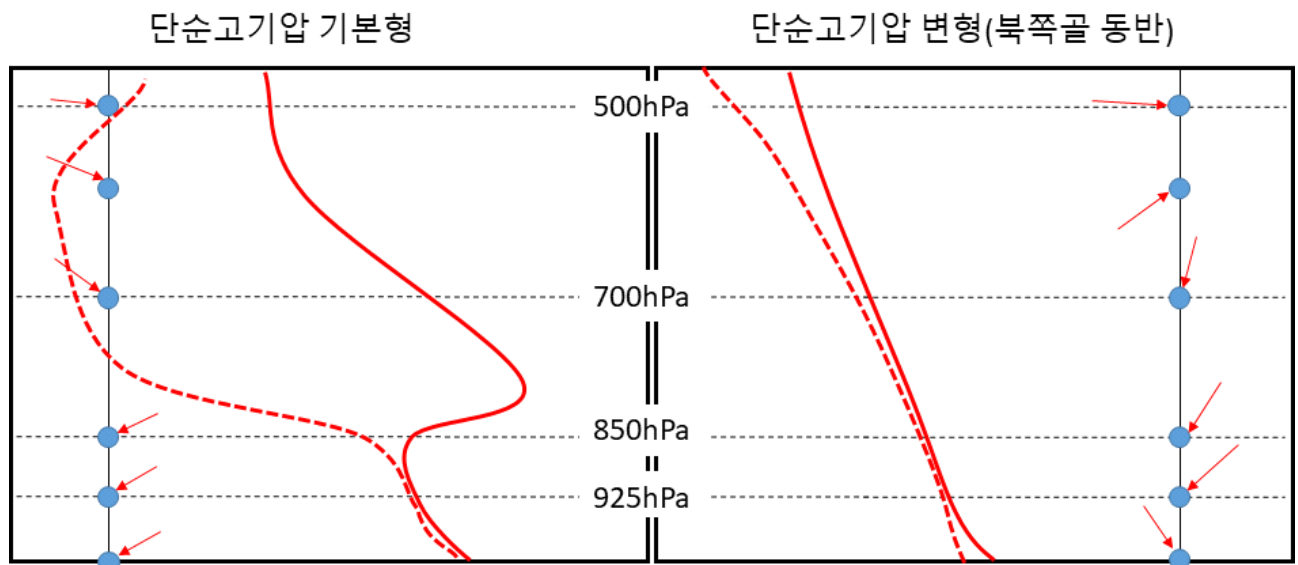
그림 4-42. 'cP확장형'의 열역학선도 모식도 기본형(좌, 2020년 1월 24일), 변형(우, 2019년 11월 3일)
