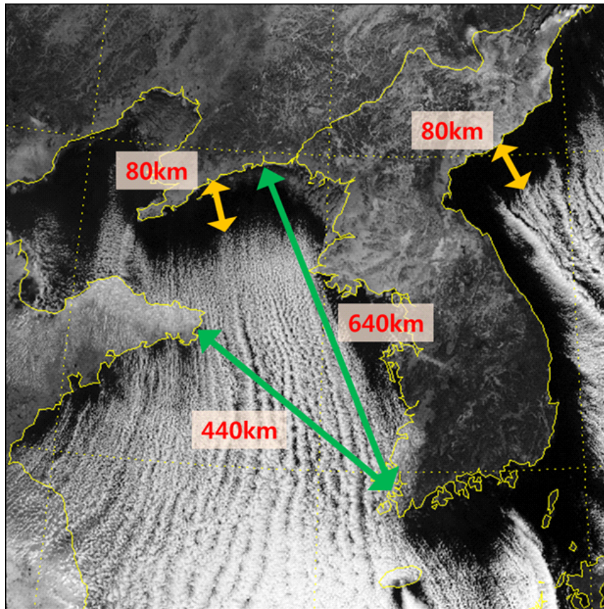
그림 3-14. 2018년 1월 26일 12시 천리안위성 가시영상, 80km 이상의 취주거리부터 구름열이 발생하는 것을 알 수 있으며, 목포의 경우 취주거리가 충분한 거리에 위치하고 있음
