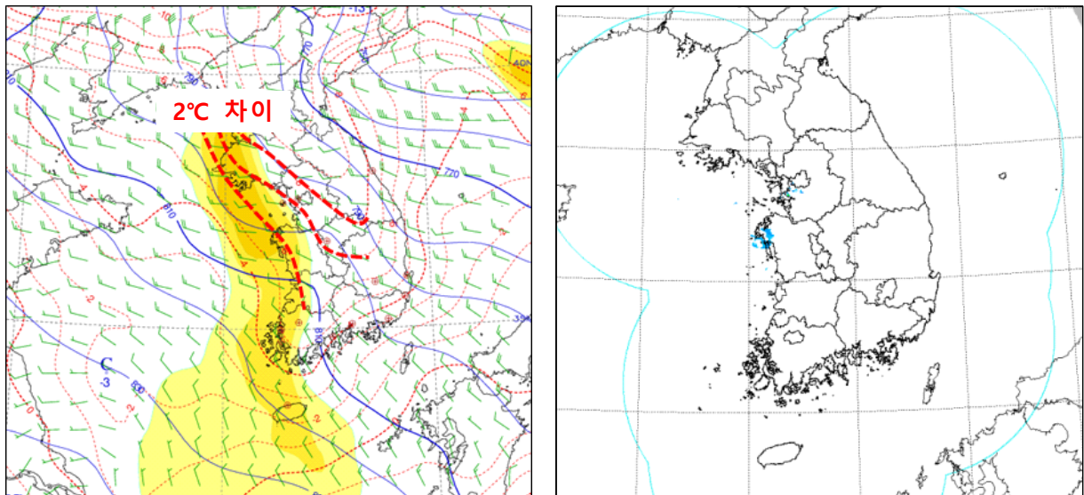
그림 1-7. 2017. 12. 25. 21시의 (좌) 925hPa 상세바람장 (우) 레이더 합성영상
