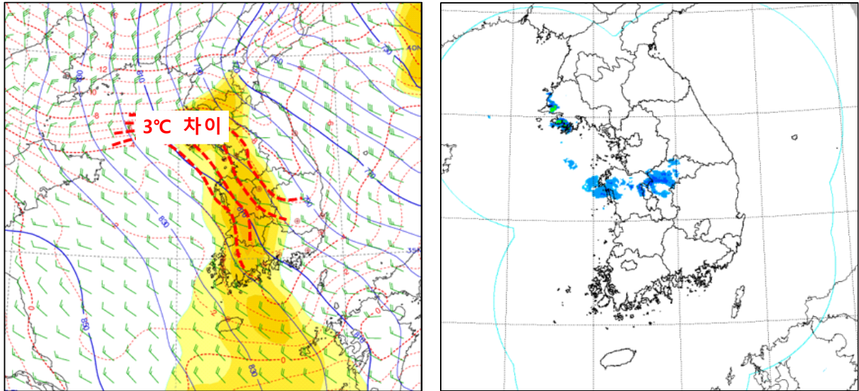
그림 1-8. 2017. 12. 26. 03시 (좌) 925hPa 상세바람장 (우) 레이더 합성영상
