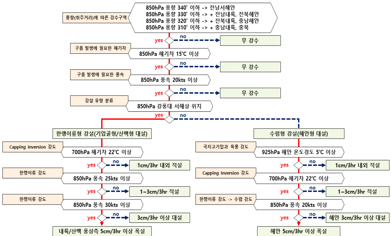
그림 3-34. 서해안형 강설 판단을 위한 흐름도
