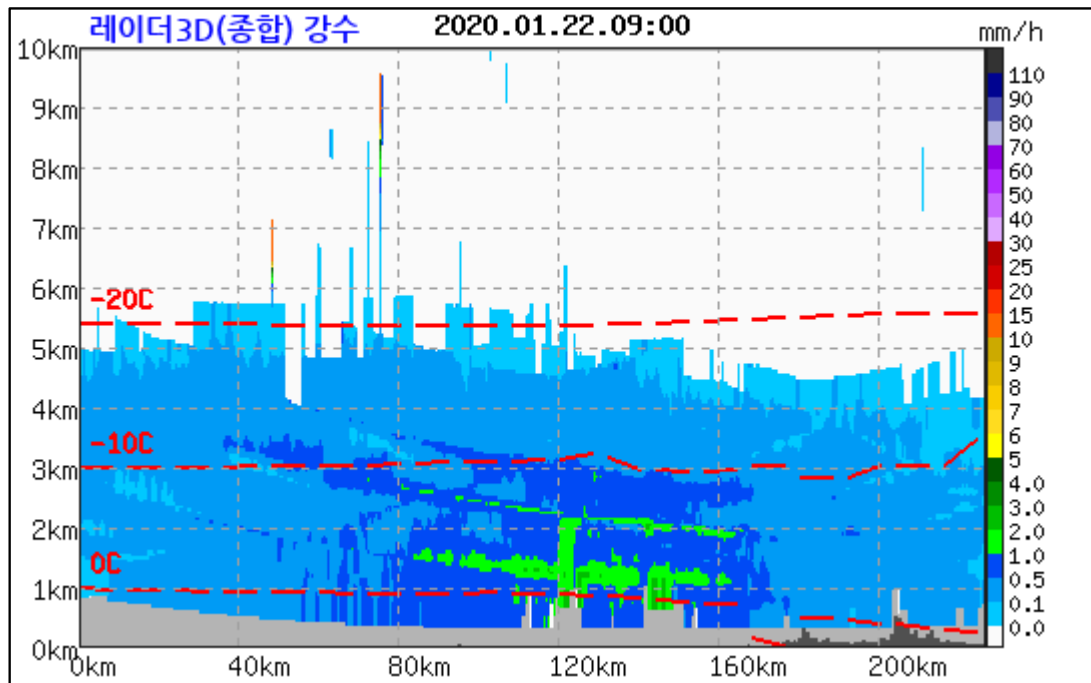
그림 5-12. 2020년 1월 22일 09시 레이더 단면도(그림 5-10 오른쪽 영상의 빨간선 단면)
