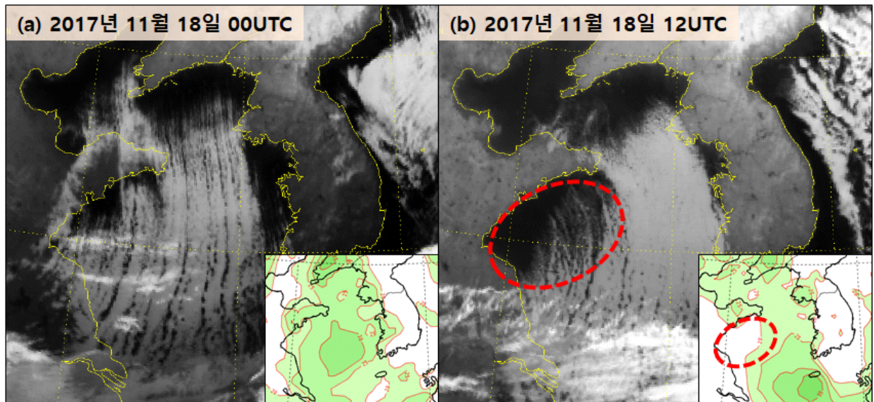
그림 3-12. 2017년 11월 18일 00UTC(좌), 12UTC(우) 천리안위성 적외영상 및 850hPa 등풍속선 (녹색 음영: 풍속 20kts 이상, 붉은 점선: 850hPa 풍속 20kts 이하로 구름대 약화된 구역)
