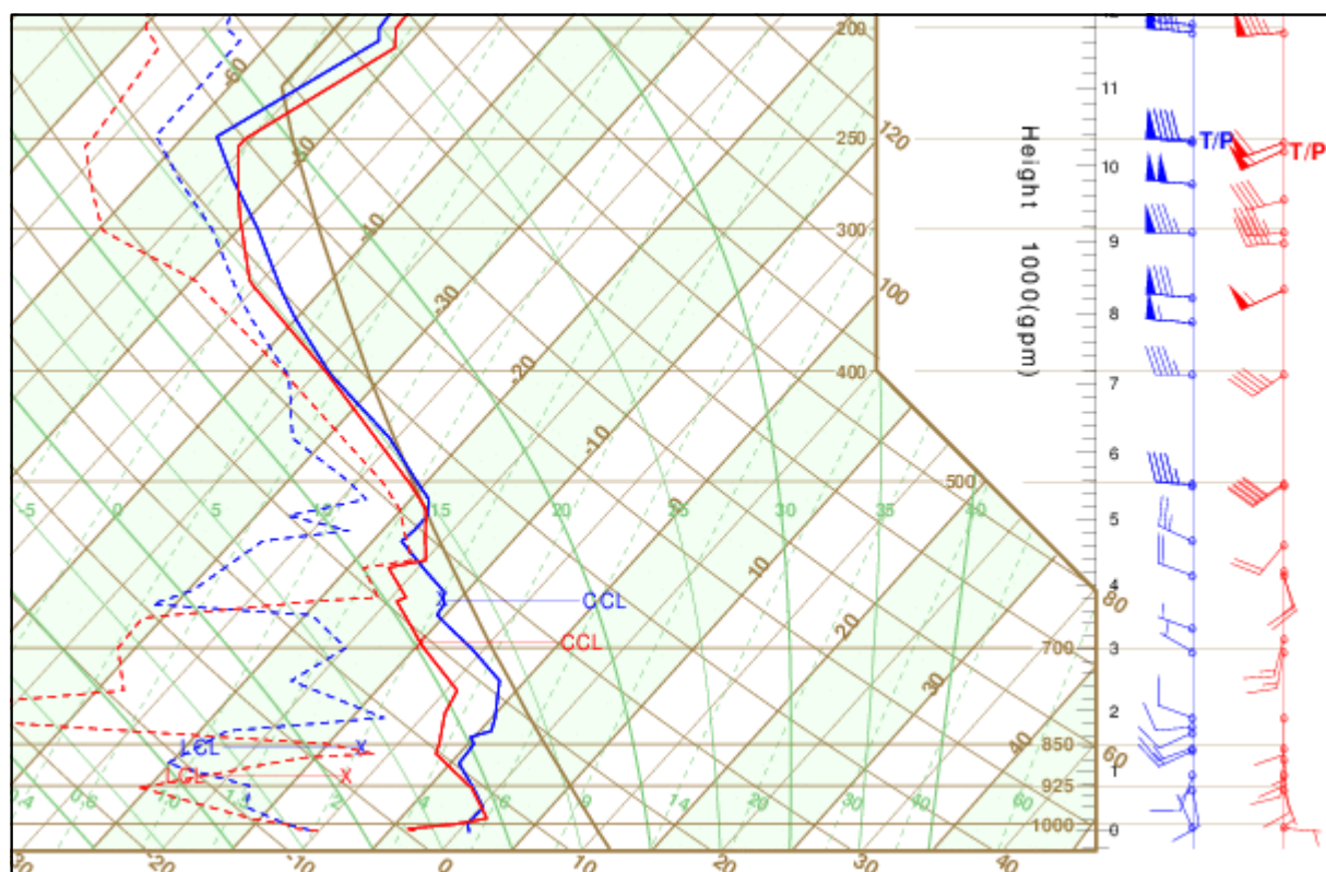
그림 5-21. 2020년 3월 7일 09시 오산 단열선도
