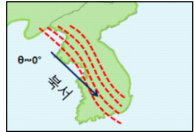
그림 1-9. 온도이류 모식도(서풍) 그림 1-10. 온도이류 모식도(남서) 그림 1-11. 온도이류 모식도(북서)
