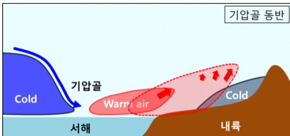
그림 2-4. 한랭역 지원에 의한 온난이류형 강수 모식도
