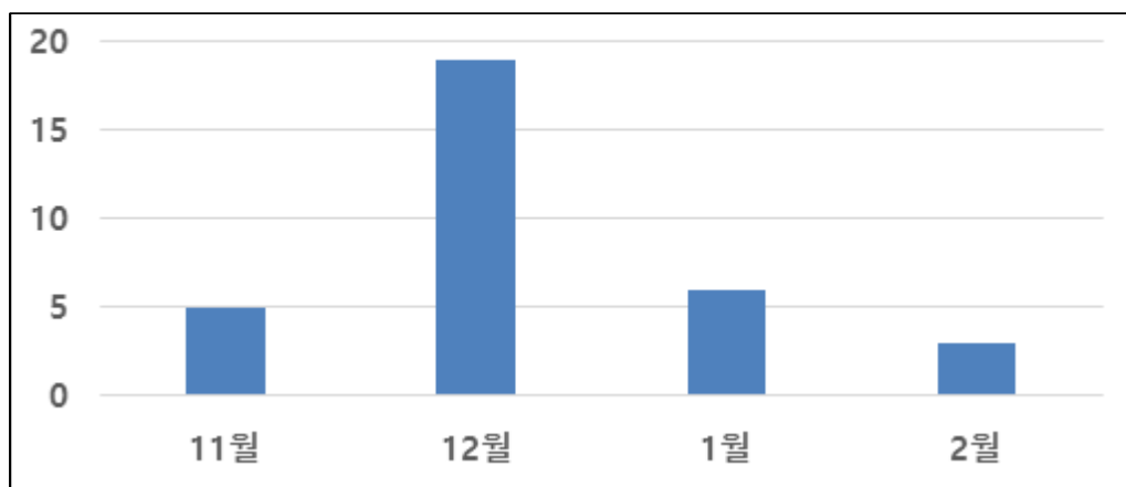
그림 1-4. 2017~2020년 월별 온난이류형 강수 발생 일수
