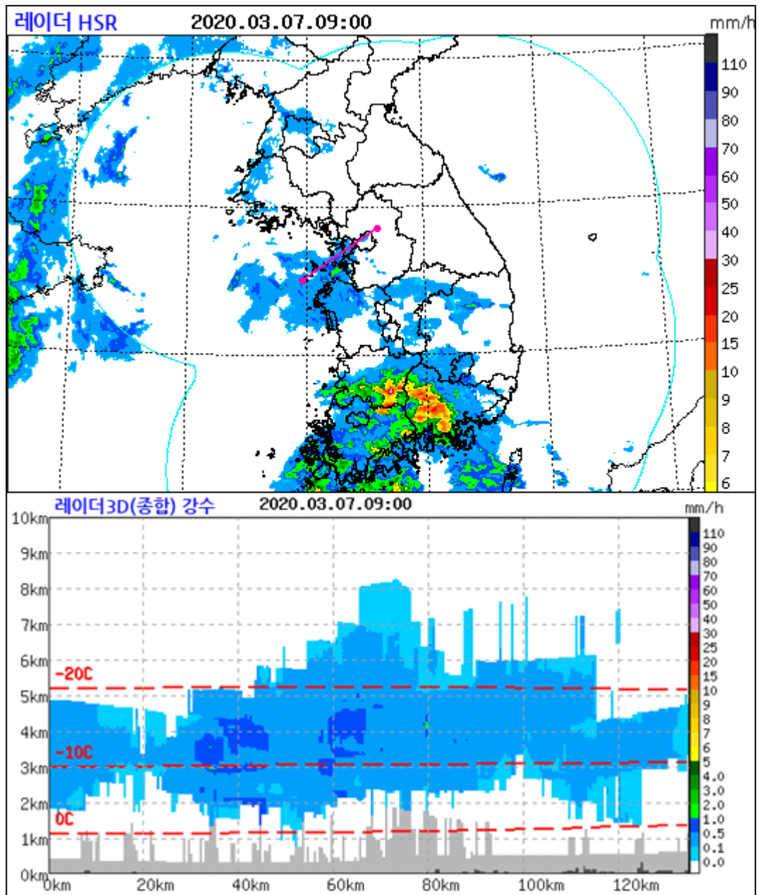
그림 5-22. 2020년 3월 7일 09시 레이더 합성영상(HSR) 수도권 단면도
