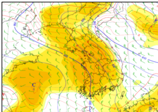
그림 1-12. 925hPa 상세바람장 (2017. 12. 29. 06시)
