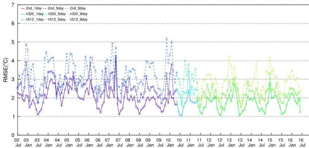
그림 3.5.4 GDLM 최저기온 월별 RMSE 성능 변화
