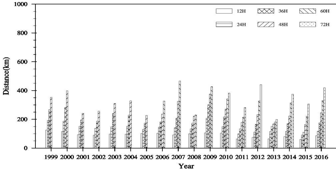
그림 3.7.2 지역예보모델의 태풍진로 모의성능 변화(2009년 이전(MM5 30km), 2010년(UM 12kmL38), 2011년 이후(UM 12kmL70)).
