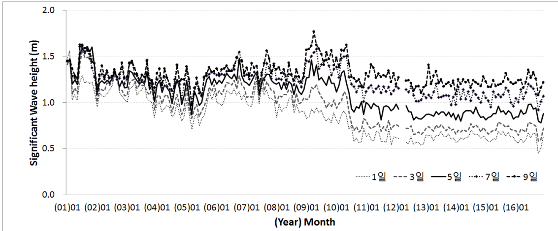
그림 3.6.1 전지구 파랑모델(GWW3) 유의파고 위성검증 RMSE
