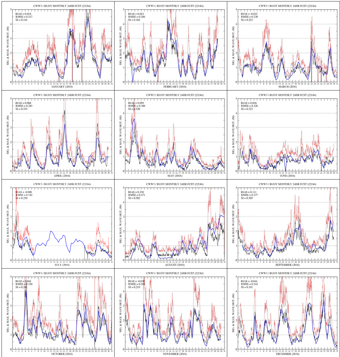
그림 3.6.35 추자도 부이 관측(검은색 실선)과 CWW3 +24H 예측 유의파고(파란색 실선) 시계열 (2016년 1월~12월). 붉은색 점선은 최대 파고.
