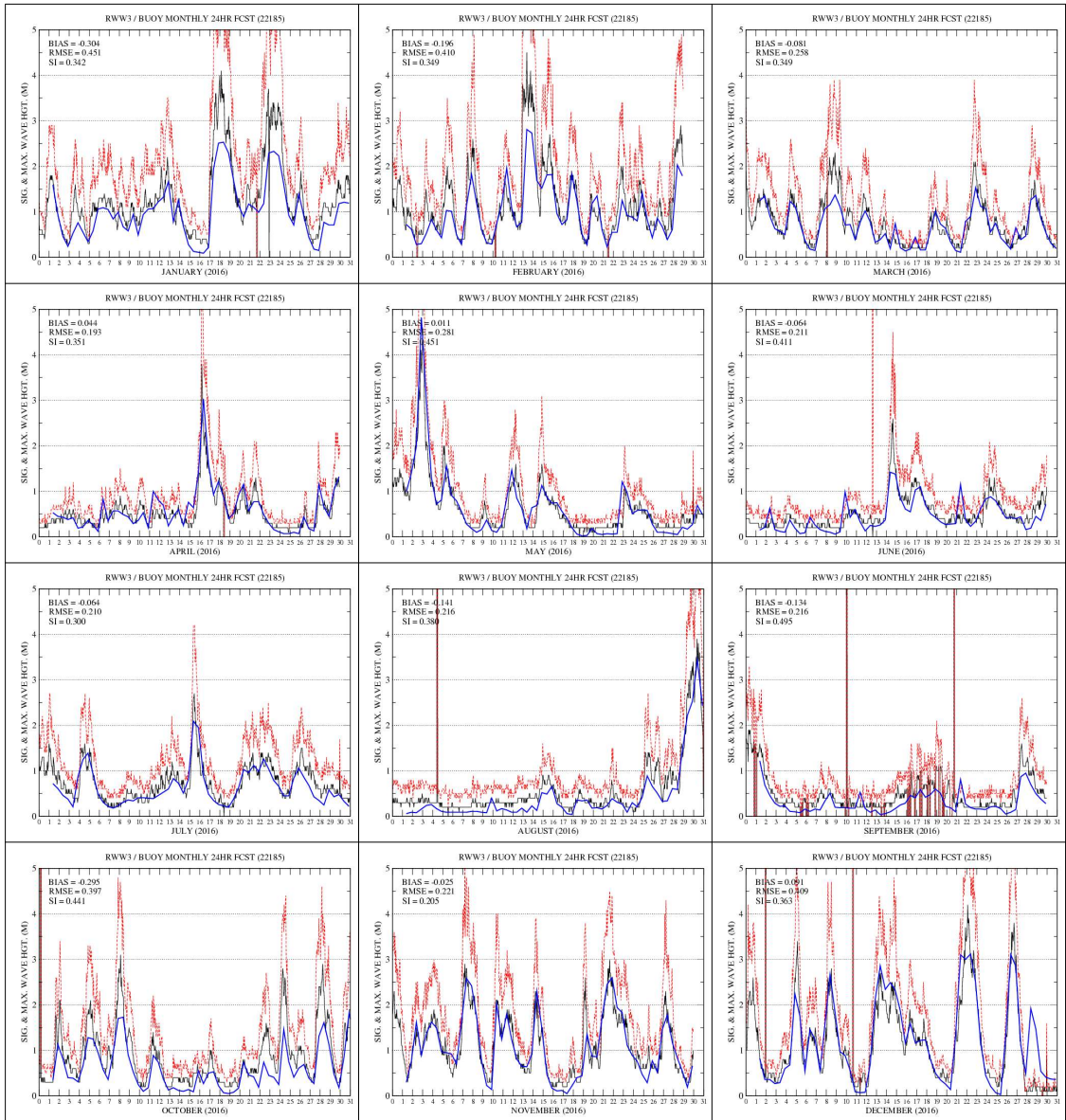
그림 3.6.20 인천 부이 관측(검은색 실선)과 RWW3 +24H 예측 유의파고(파란색 실선) 시계열 (2016년 1월~12월). 붉은색 점선은 최대 파고.
