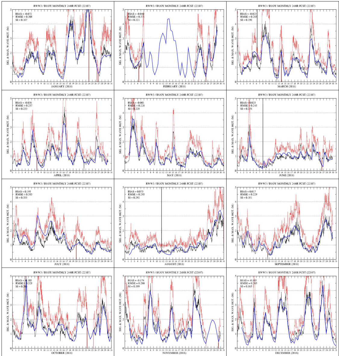
그림 3.6.16 마라도 부이 관측(검은색 실선)과 RWW3 +24H 예측 유의파고(파란색 실선) 시계열 (2016년 1월~12월). 붉은색 점선은 최대 파고.
