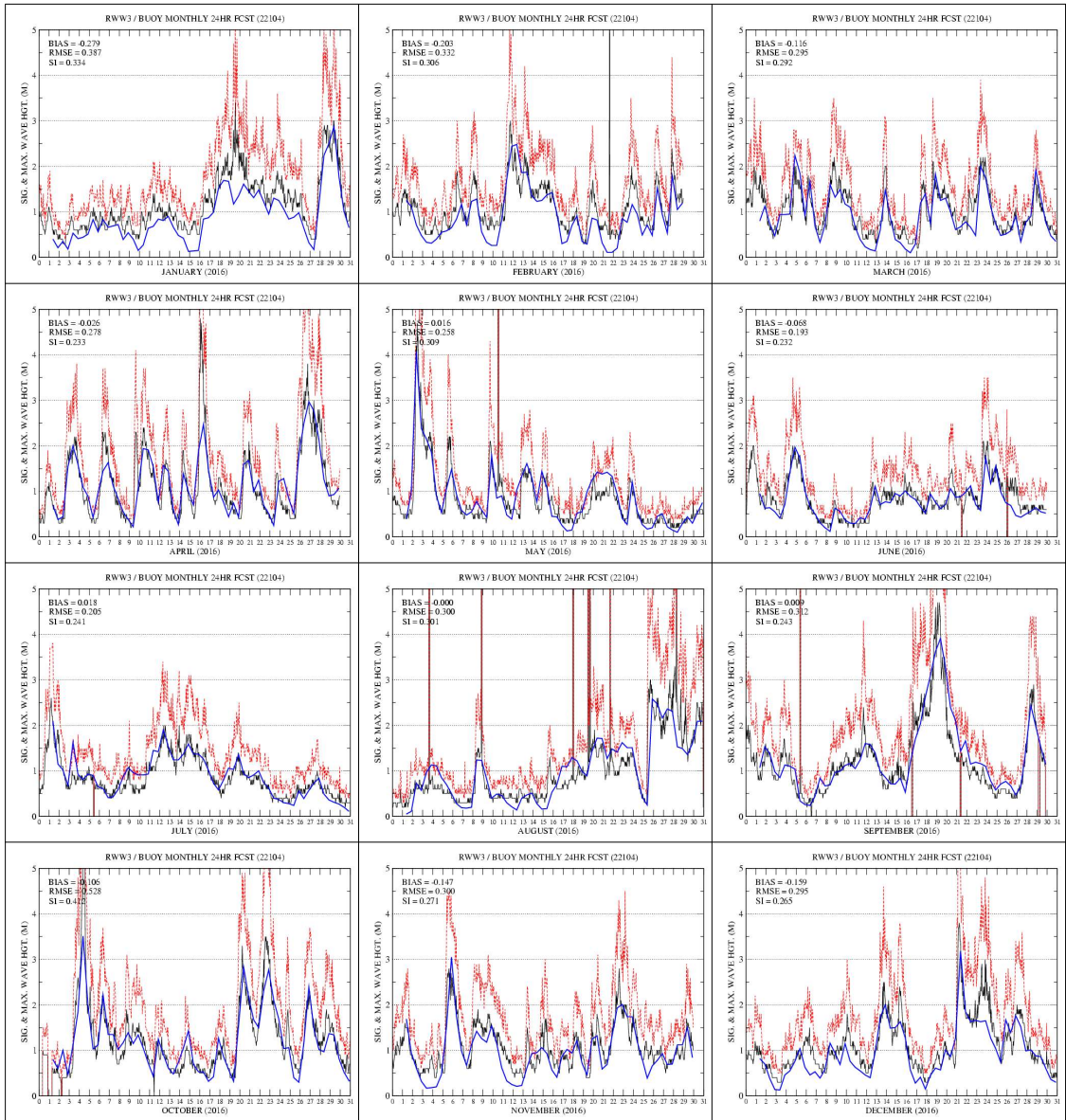
그림 3.6.13 거제도 부이 관측(검은색 실선)과 RWW3 +24H 예측 유의파고(파란색 실선) 시계열 (2016년 1월~12월). 붉은색 점선은 최대 파고.
