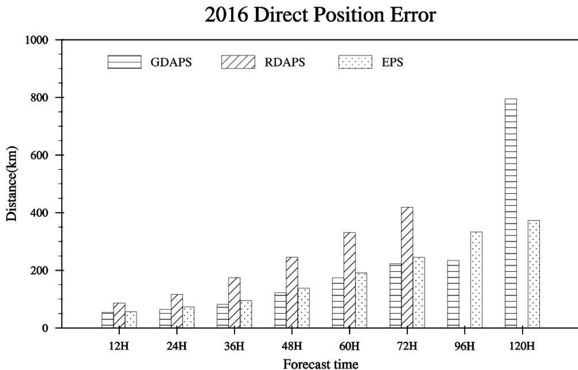
그림 3.7.4 2016년 수치예보모델별 평균단순거리오차(Direct Position Error).
