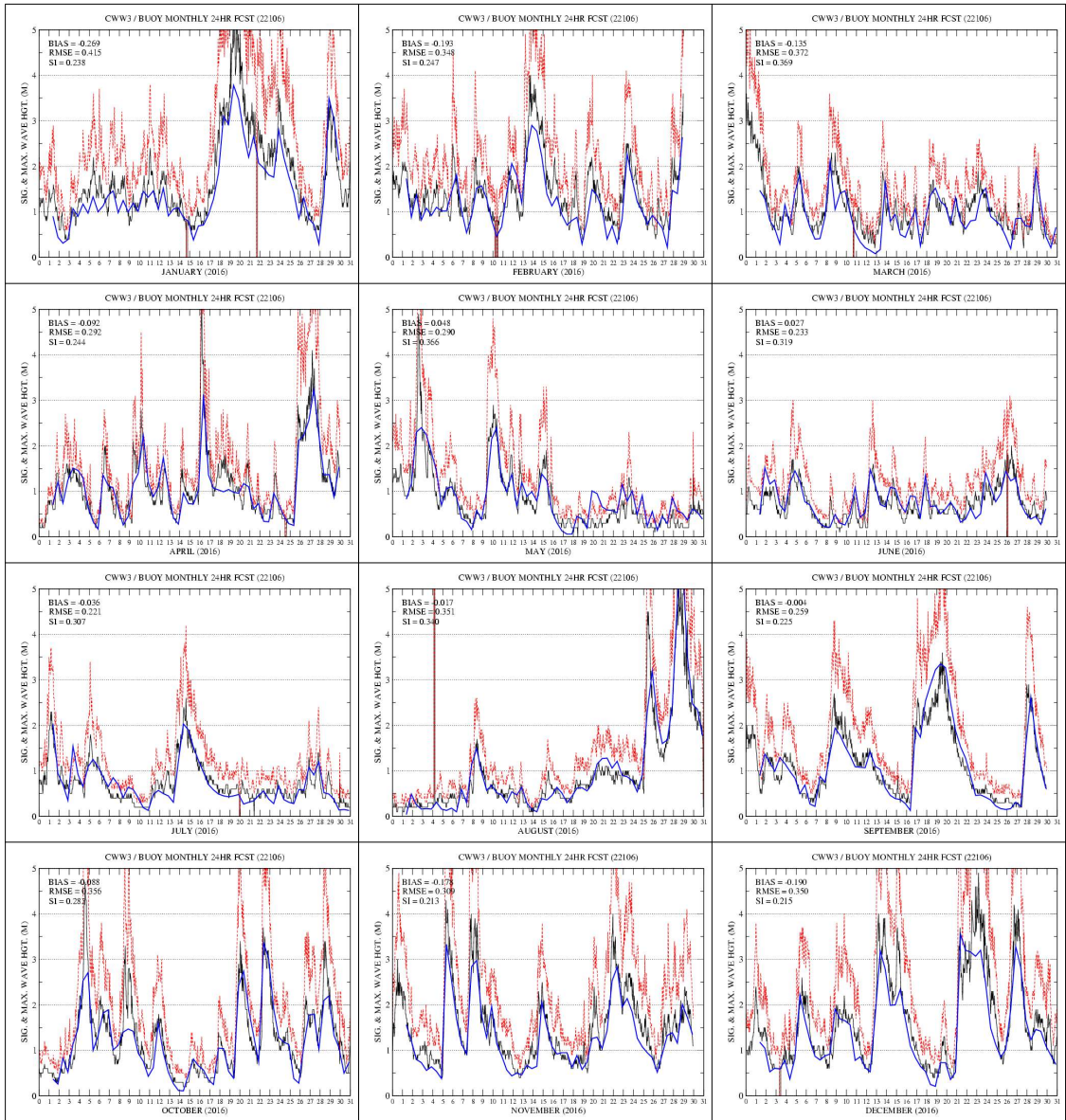
그림 3.6.31 포항 부이 관측(검은색 실선)과 CWW3 +24H 예측 유의파고(파란색 실선) 시계열 (2016년 1월~12월). 붉은색 점선은 최대 파고.
