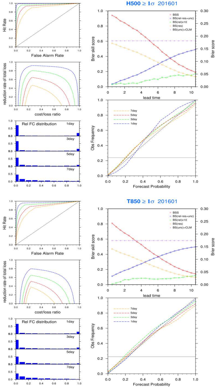
그림 3.4.7 2016년 1월 EPSG 북반구 500hPa 지위고도(상)와 850hPa 기온(하)의 +1 표준편차에 대한 확률예측 성능 (왼쪽 상단부터 ROC curve, Economic Value, Rank histogram, 오른쪽 상단부터 Brier Score, Reliability Table)
