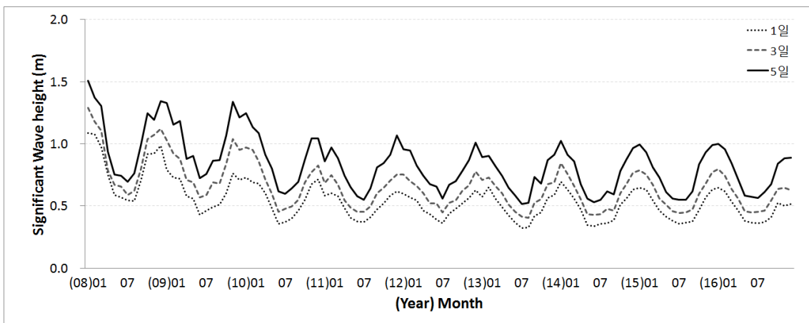
그림 3.6.2 전지구 파랑모델(GWW3) 유의파고 부이검증 RMSE
