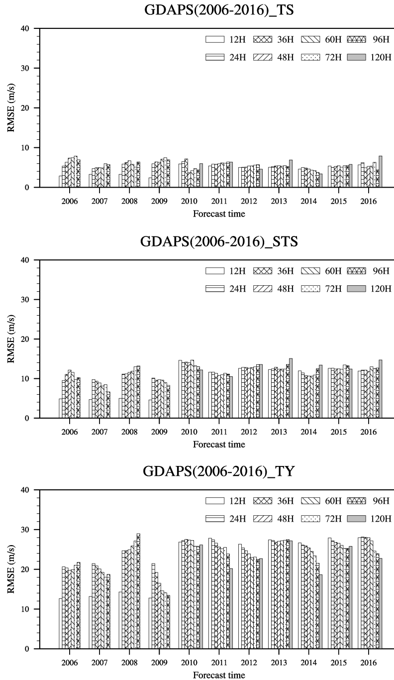
그림 3.7.11 전지구예보모델의 태풍 강도별 최대풍속 모의성능 변화(2006~2009년(T426L40), 2010년(UM N320L50), 2011년 이후(UM N512L70), 2016년 이후(UM N768L70)).
