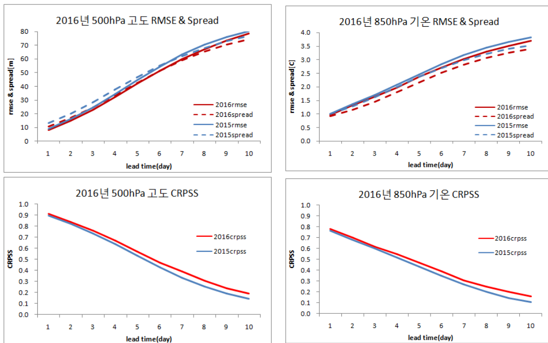
그림 2.11 2015년 및 2016년 EPSG 북반구 평균 RMSE/Spread와 CRPSS
