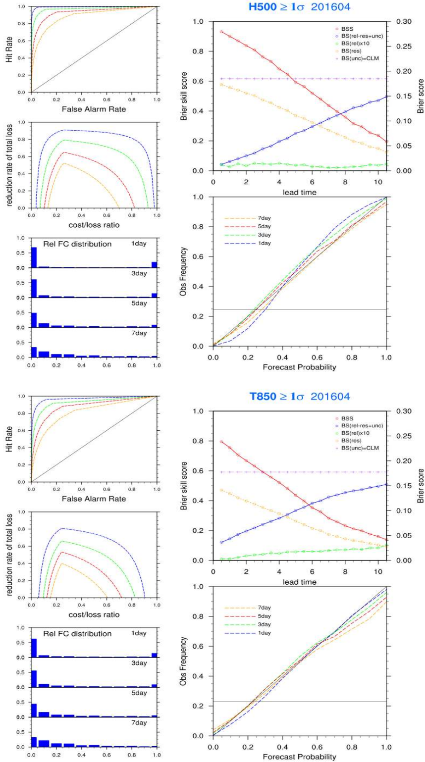
그림 3.4.10 2016년 4월 EPSG 북반구 500hPa 지위고도(상)와 850hPa 기온(하)의 +1 표준편차에 대한 확률예측 성능 (왼쪽 상단부터 ROC curve, Economic Value, Rank histogram, 오른쪽 상단부터 Brier Score, Reliability Table)
