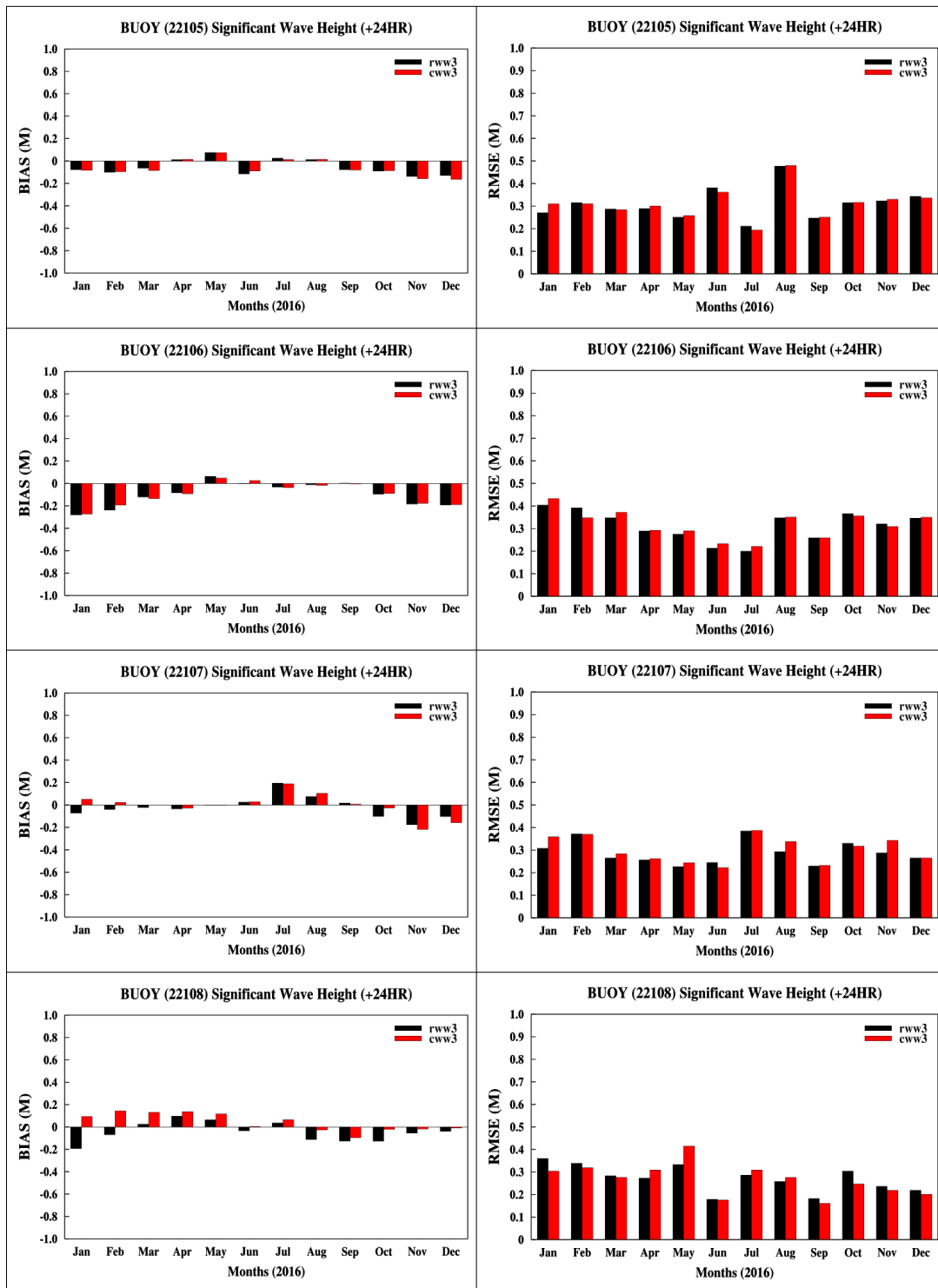
그림 3.6.43 4개 부이관측지점(22105~22108)에 대한 CWW3(붉은색)과 RWW3(검정색)의 +24H 예측 유의파고의 BIAS(왼쪽)와 RMSE(오른쪽)
