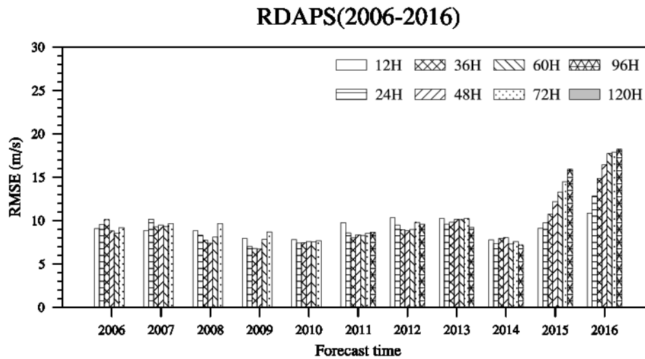
그림 3.7.9 지역예보모델의 태풍 최대풍속 모의성능 변화(2009년 이전(MM5 30km), 2010년(UM 12kmL38), 2011년 이후(UM 12kmL70)).
