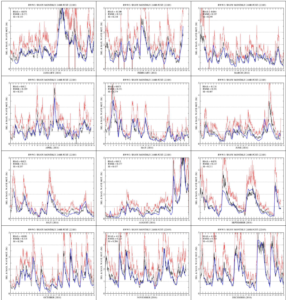
그림 3.6.14 동해 부이 관측(검은색 실선)과 RWW3 +24H 예측 유의파고(파란색 실선) 시계열 (2016년 1월~12월). 붉은색 점선은 최대 파고.
