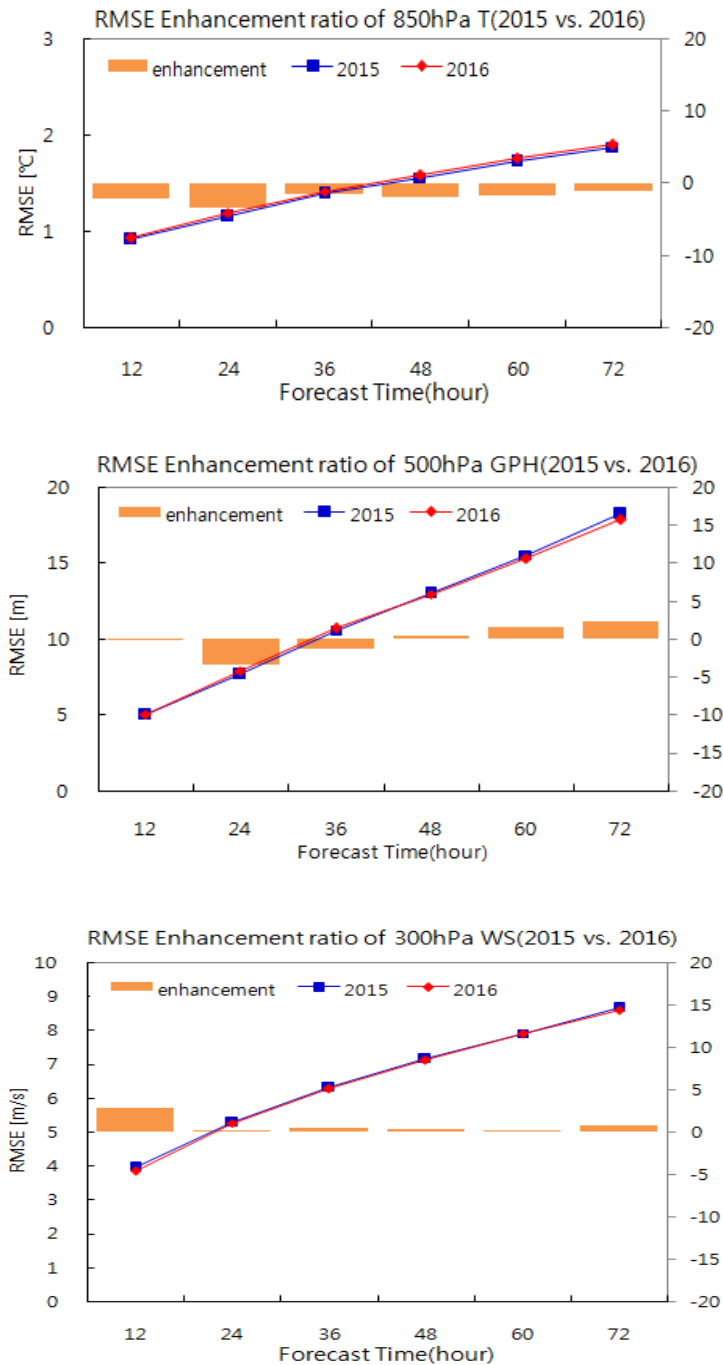
그림 2.7 지역예측시스템(UM 12km L70) 분석검증 RMSE 2015년 대비 2016년 개선 정도
