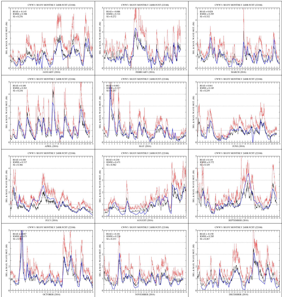
그림 3.6.39 통영 부이 관측(검은색 실선)과 CWW3 +24H 예측 유의파고(파란색 실선) 시계열 (2016년 1월~12월). 붉은색 점선은 최대 파고.
