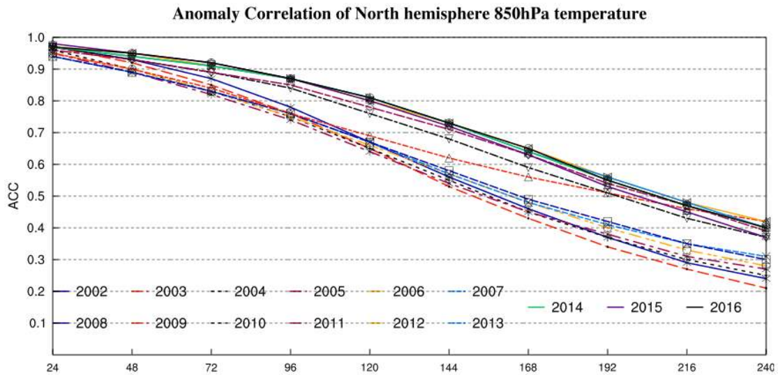
그림 2.3 전지구예측시스템(GDAPS) 북반구 850hPa 기온 분석검증 이상상관 계수 예보시간별, 연별 변화
