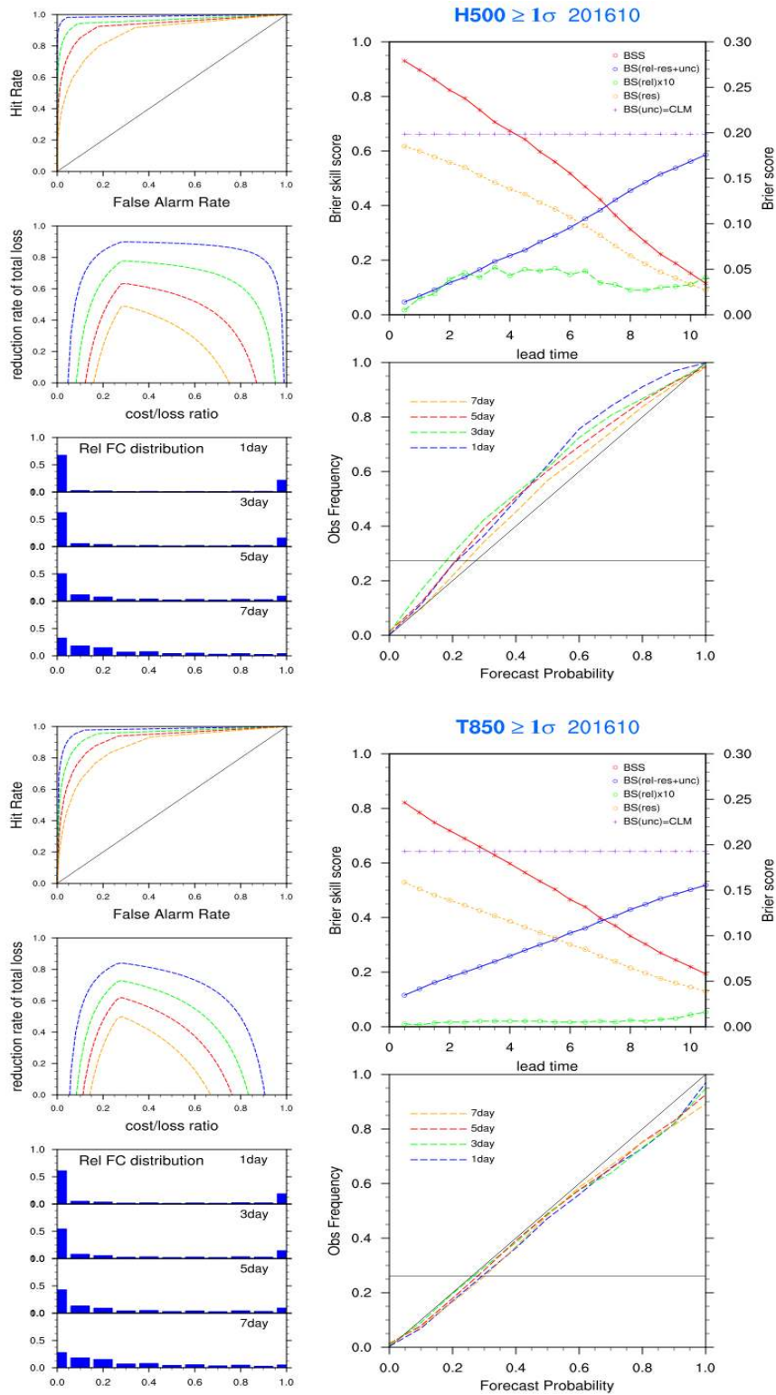
그림 3.4.16 2016년 10월 EPSG 북반구 500hPa 지위고도(상)와 850hPa 기온(하)의 +1 표준편차에 대한 확률예측 성능 (왼쪽 상단부터 ROC curve, Economic Value, Rank histogram, 오른쪽 상단부터 Brier Score, Reliability Table)
