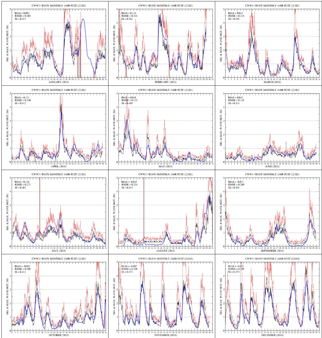
그림 3.6.27 칠발도 부이 관측(검은색 실선)과 CWW3 +24H 예측 유의파고(파란색 실선) 시계열 (2016년 1월~12월). 붉은색 점선은 최대 파고.
