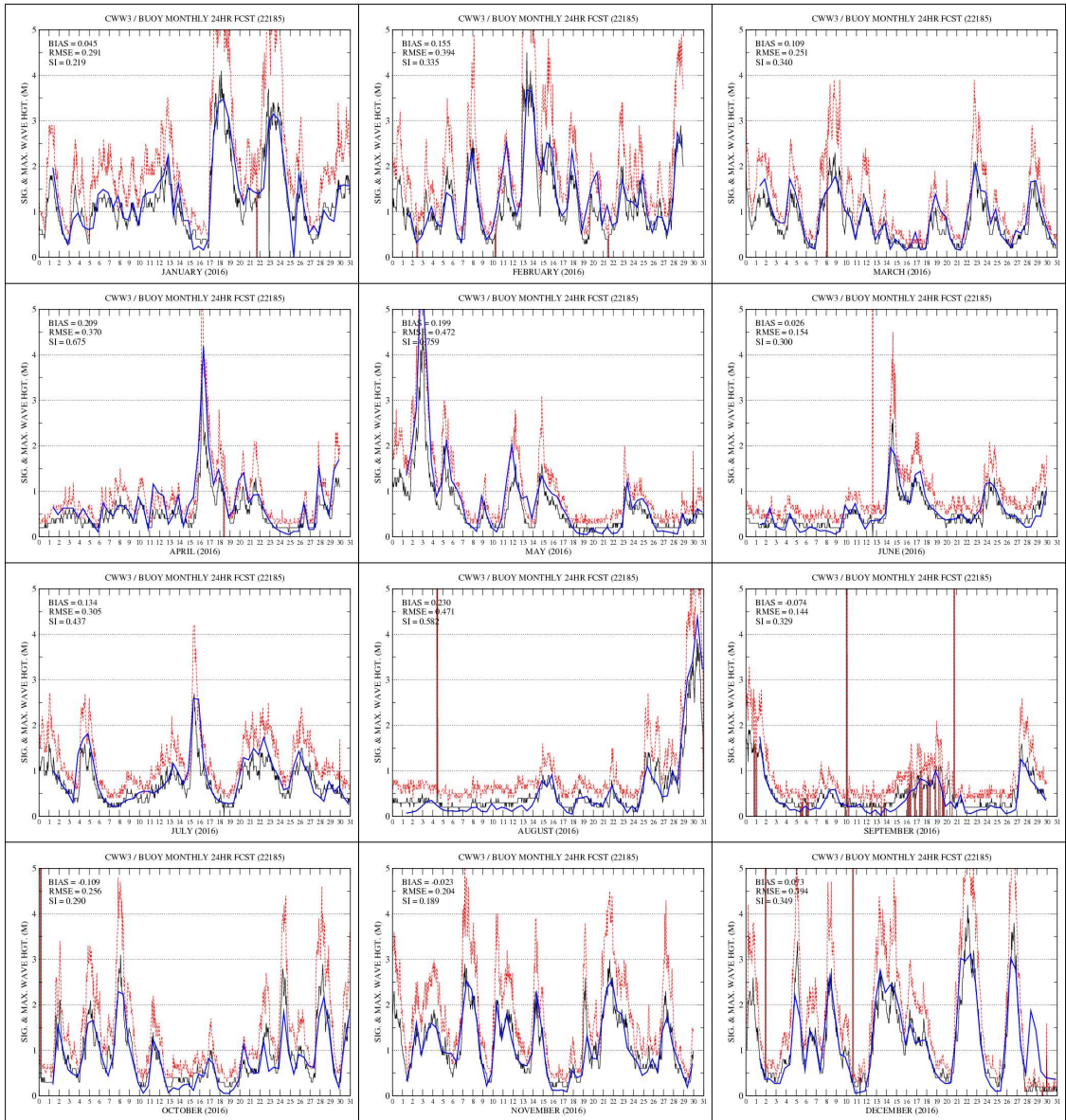
그림 3.6.36 인천 부이 관측(검은색 실선)과 CWW3 +24H 예측 유의파고(파란색 실선) 시계열 (2016년 1월~12월). 붉은색 점선은 최대 파고.
