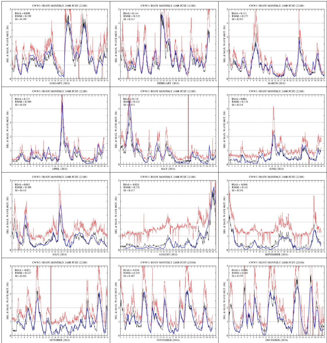
그림 3.6.33 외연도 부이 관측(검은색 실선)과 CWW3 +24H 예측 유의파고(파란색 실선) 시계열 (2016년 1월~12월). 붉은색 점선은 최대 파고.
