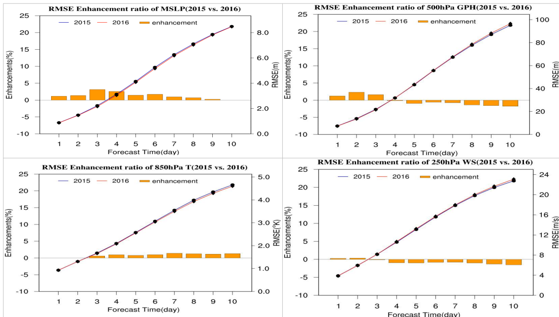
그림 2.1 전지구예측시스템(GDAPS) 북반구 분석검증 RMSE 2015년 대비 2016년 개선 정도
