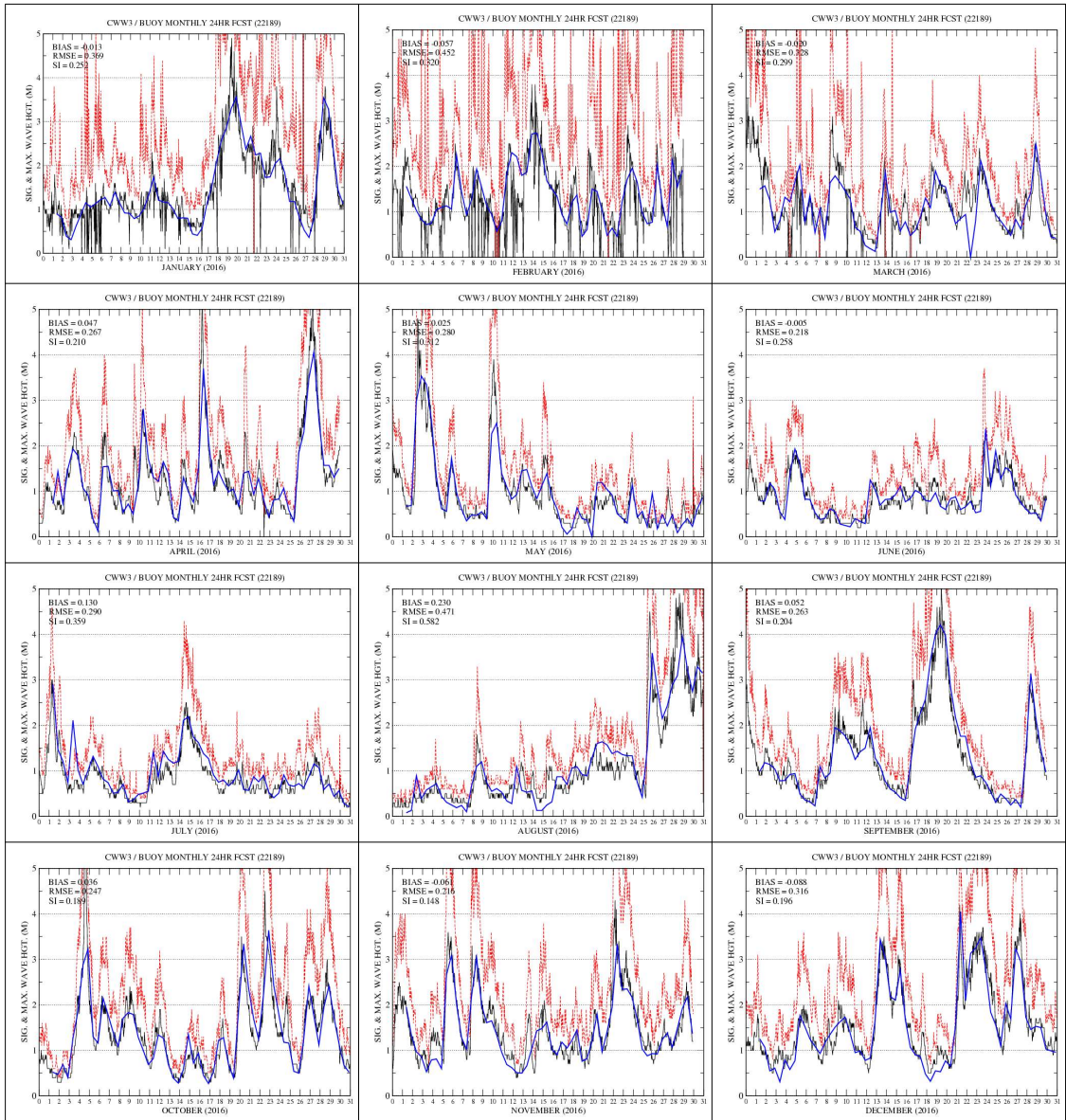
그림 3.6.40 울산 부이 관측(검은색 실선)과 CWW3 +24H 예측 유의파고(파란색 실선) 시계열 (2016년 1월~12월). 붉은색 점선은 최대 파고.
