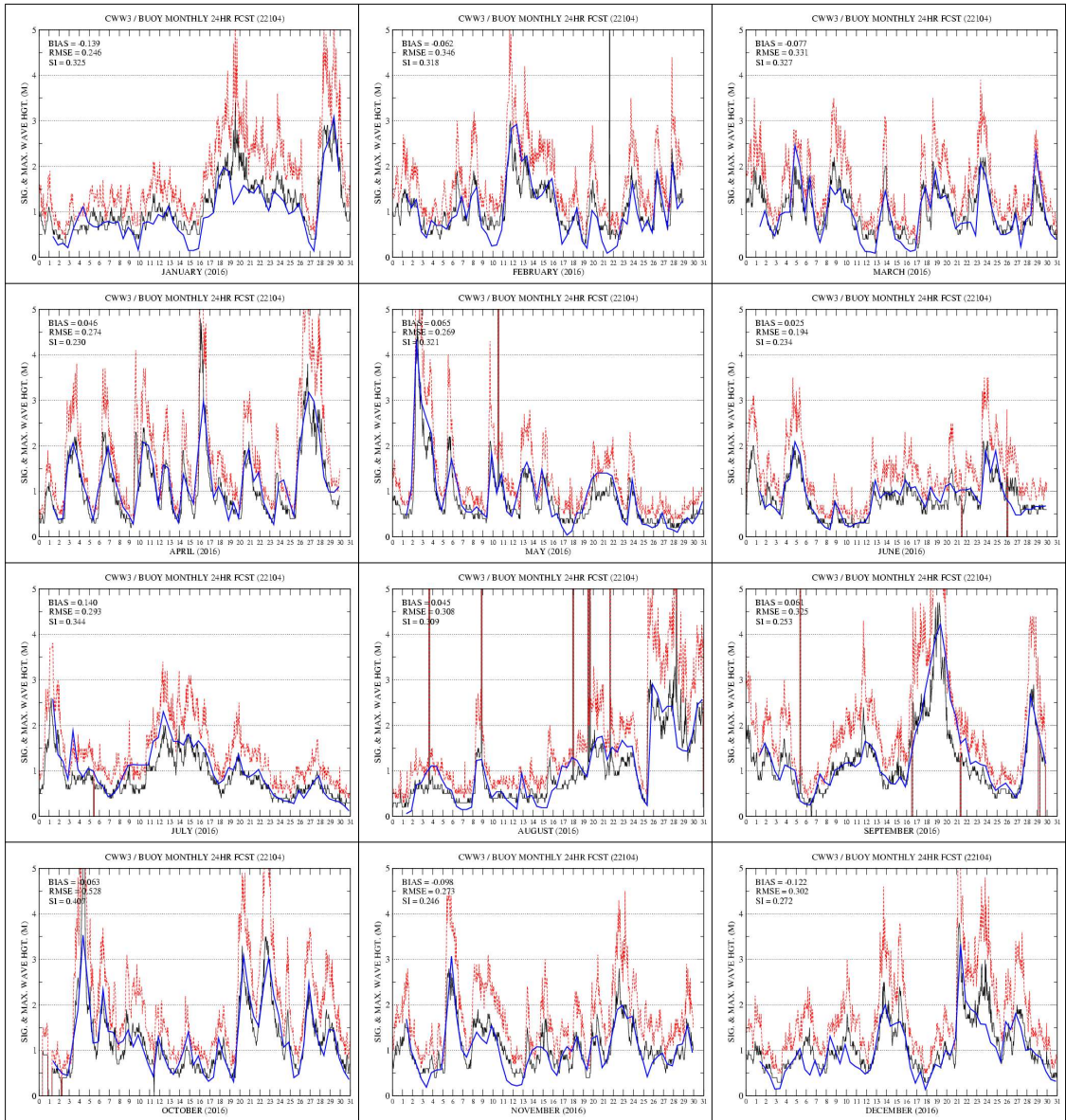
그림 3.6.29 거제도 부이 관측(검은색 실선)과 CWW3 +24H 예측 유의파고(파란색 실선) 시계열 (2016년 1월~12월). 붉은색 점선은 최대 파고.
