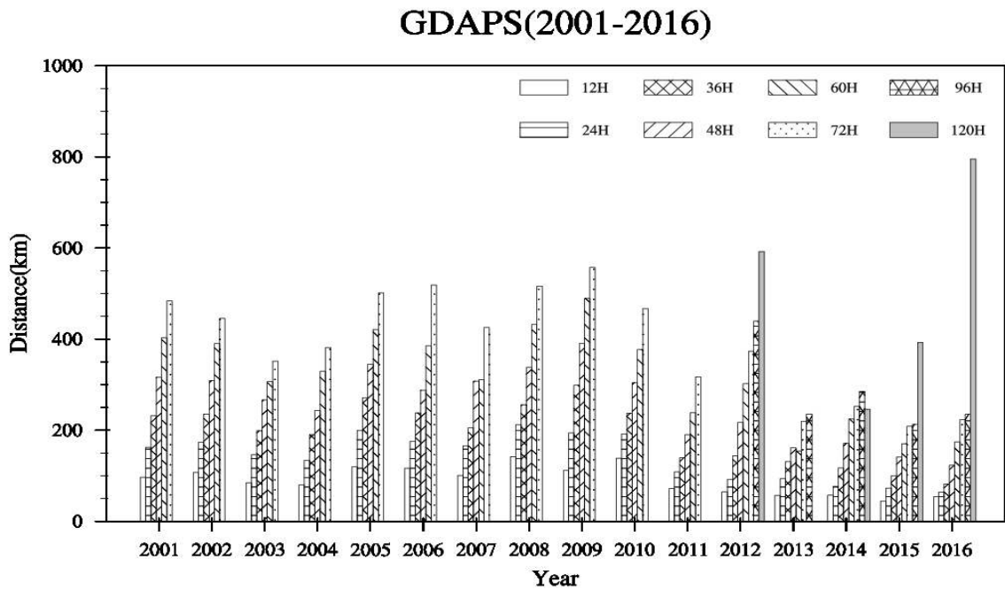
그림 3.7.1 전지구예측시스템의 태풍진로 모의성능 변화(2006년 이전(T213L30), 2006~2009년(T426L40), 2010년(UM N320L50), 2011년 이후(UM N512L70), 2016년 이후(UM N768L70)).
