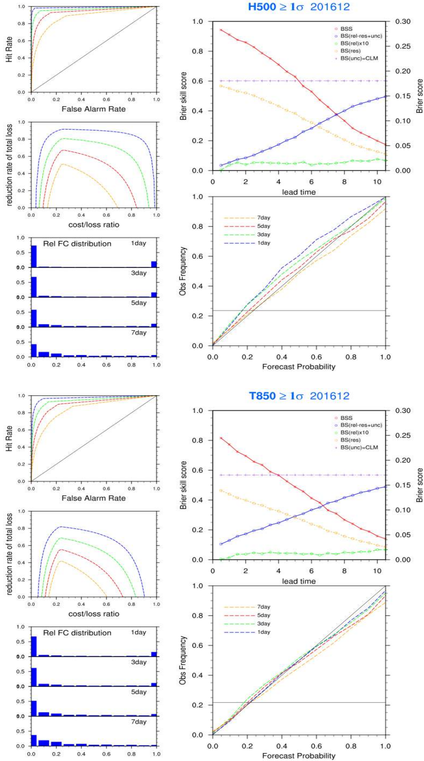
그림 3.4.18 2016년 12월 EPSG 북반구 500hPa 지위고도(상)와 850hPa 기온(하)의 +1 표준편차에 대한 확률예측 성능 (왼쪽 상단부터 ROC curve, Economic Value, Rank histogram, 오른쪽 상단부터 Brier Score, Reliability Table)
