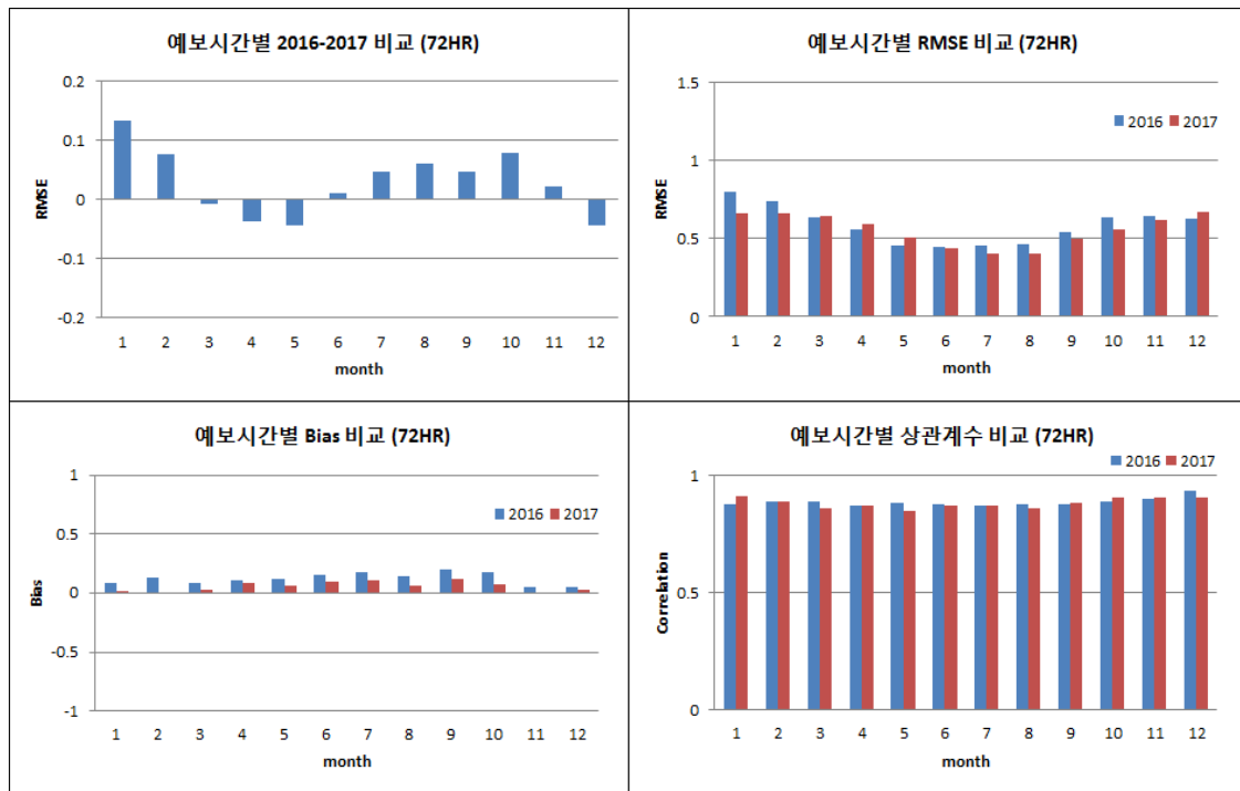
그림 3.5.7 GWW3 +72H예보장에 대한 전년 대비 성능 비교. BIAS, RMSE, Correlation
