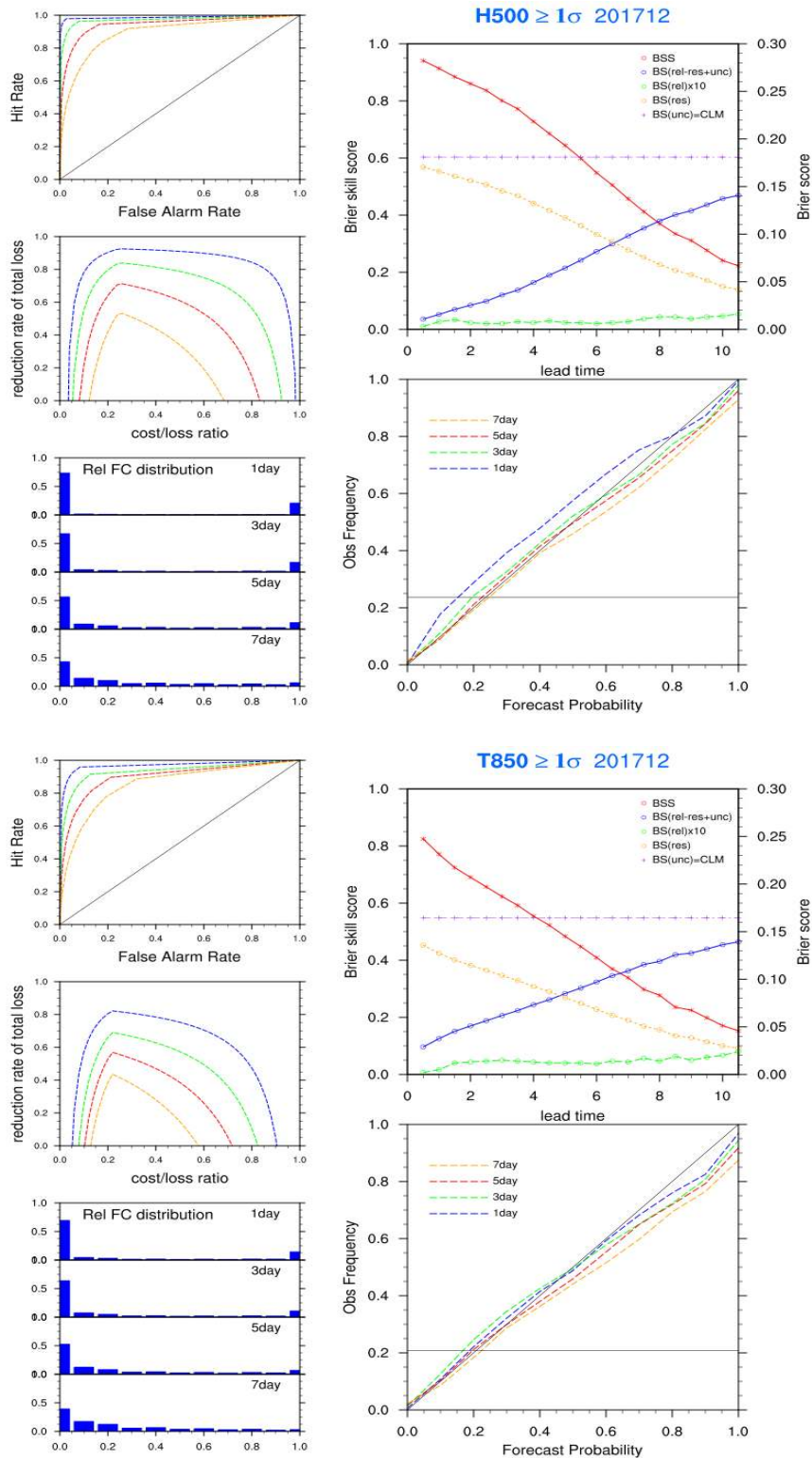
그림 3.4.18 2017년 12월 EPSG 북반구 500hPa 지위고도(상)와 850hPa 기온(하)의 +1 표준편차에 대한 확률예측 성능 (왼쪽 상단부터 ROC curve, Economic Value, Rank histogram, 오른쪽 상단부터 Brier Score, Reliability Table)
