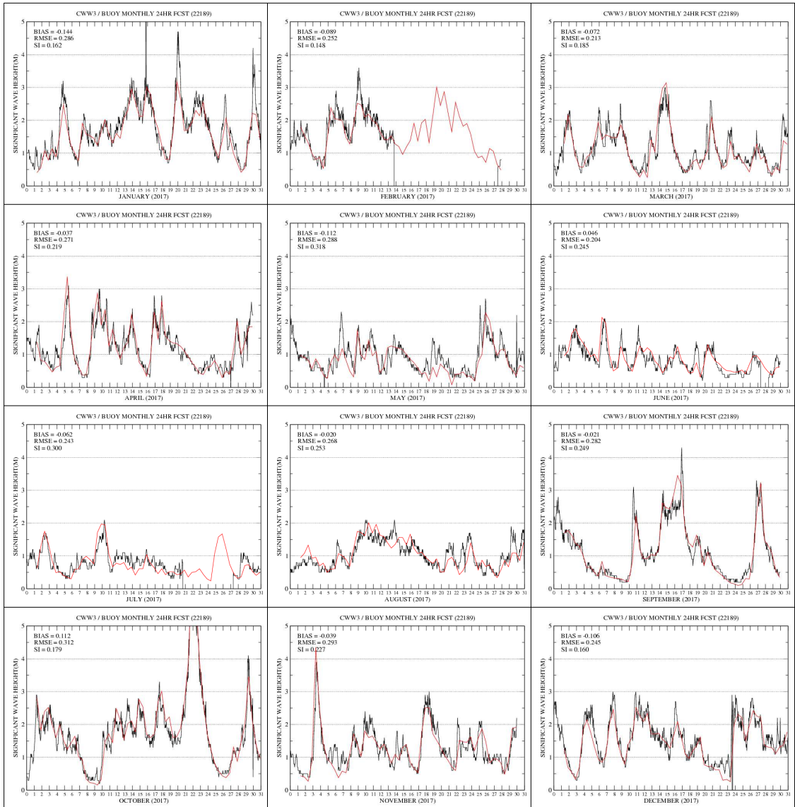
그림 3.5.40 울산 부이 관측(검은색 실선)과 CWW3 +24H 예측 유의파고(붉은색 실선) 시계열(2017년 1월~12월).
