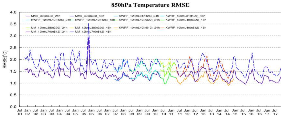
그림 3.2.2 RDAPS 850hPa 기온 예측 시간별 월평균 RMSE
