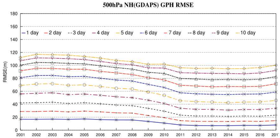
그림 2.2 전지구예측시스템(GDAPS) 북반구 분석검증 RMSE 연 평균 변화
