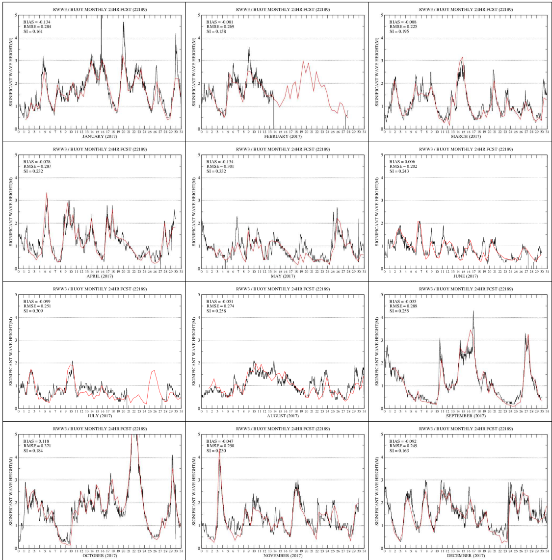
그림 3.5.24 울산 부이 관측(검은색 실선)과 RWW3 +24H 예측 유의파고(붉은색 실선) 시계열(2017년 1월~12월).
