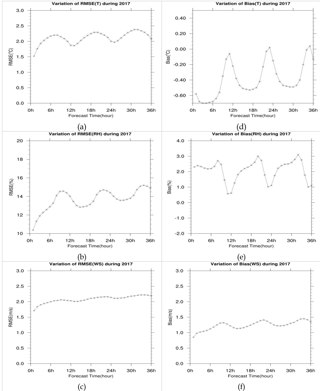
그림 3.3.1 LDAPS의 2017년 지상변수의 예보시간별 RMSE((a): 기온, (b): 상대습도, (c): 풍속) 및 Bias((d): 기온, (e): 상대습도, (f): 풍속)의 변화
