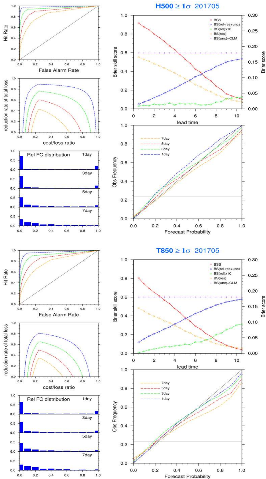
그림 3.4.11 2017년 5월 EPSG 북반구 500hPa 지위고도(상)와 850hPa 기온(하)의 +1 표준편차에 대한 확률예측 성능 (왼쪽 상단부터 ROC curve, Economic Value, Rank histogram, 오른쪽 상단부터 Brier Score, Reliability Table)
