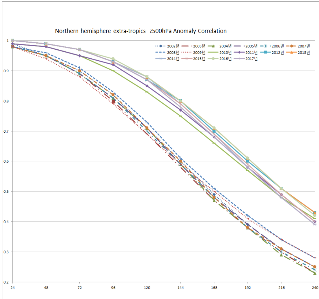
그림 2.4 전지구예측시스템(GDAPS) 북반구 500hPa 고도 분석검증 이상상관 계수 예보시간별, 연별 변화
