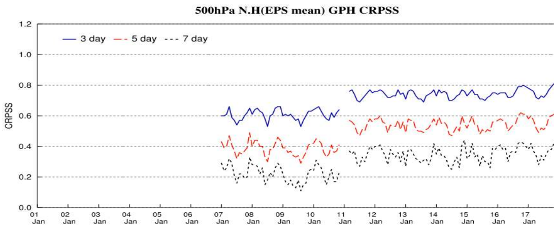
그림 3.4.3 EPSG 북반구 500hPa 지위고도 예측 시간별 월평균 CRPSS
