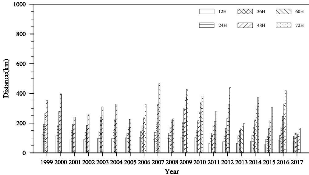
그림 3.6.2 지역예보모델의 태풍진로 모의성능 변화(2009년 이전(MM5 30km), 2010년(UM 12kmL38), 2011년 이후(UM 12kmL70)).
