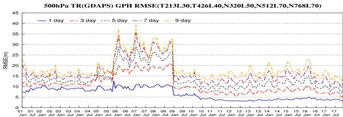
그림 3.1.3 GDAPS 적도지역 500hPa 지위고도 예측 시간별 월평균 RMSE
