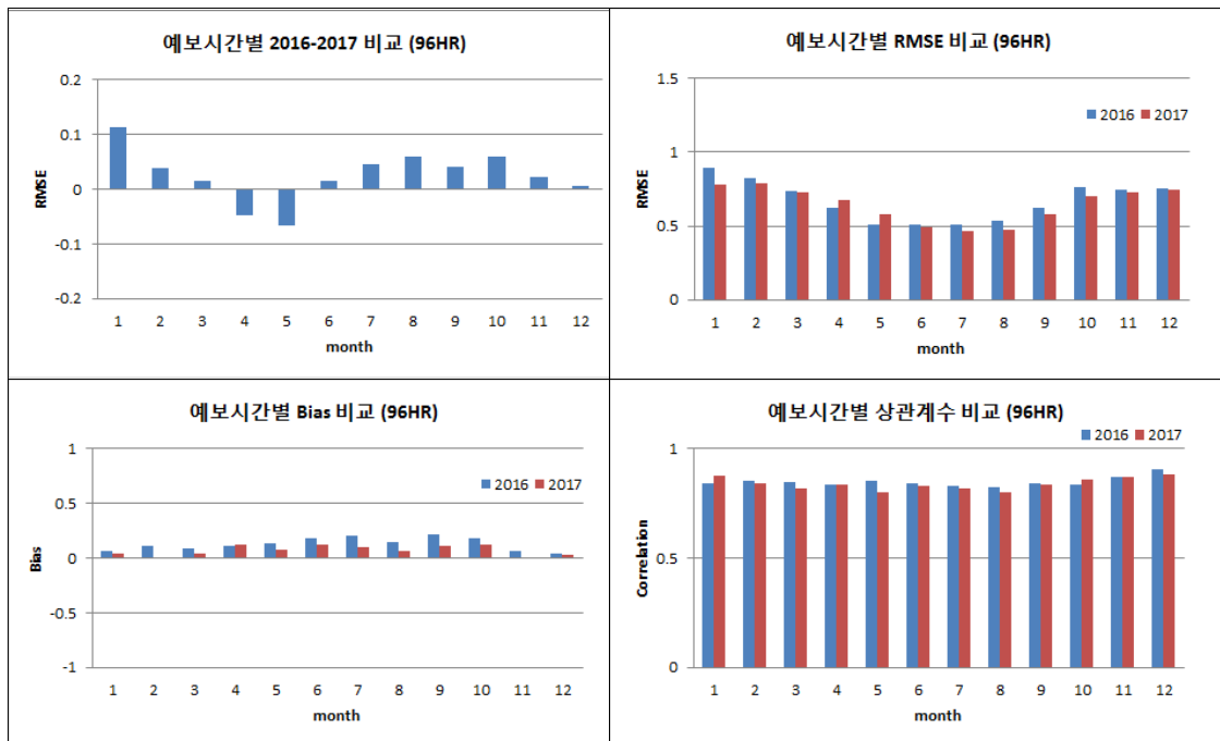
그림 3.5.8 GWW3 +96H예보장에 대한 전년 대비 성능 비교. BIAS, RMSE, Correlation
