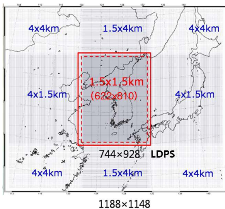
그림 1.2 가변격자 영역확장 국지모델 격자계 (내부 고정격자계는 이전과 동일)
