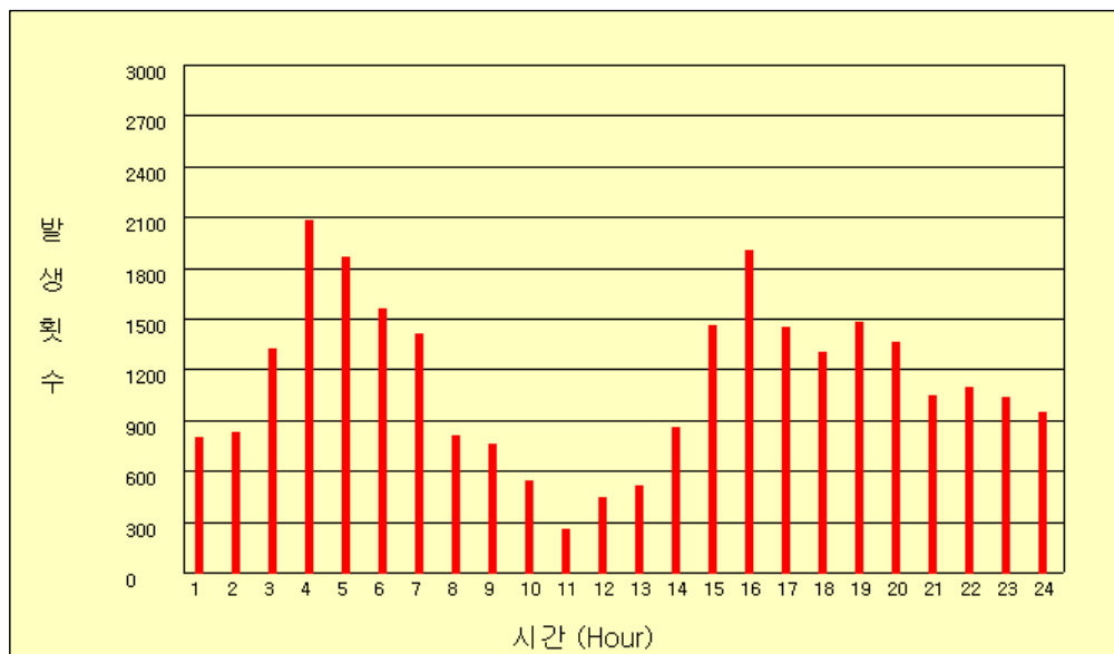
그림 34(b). 2008년 5월 시간별 낙뢰발생 횟수
