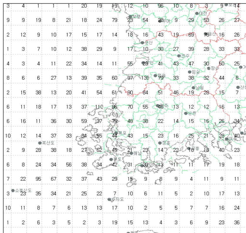
그림 28(b). 2008년 5월 전라도지역 낙뢰발생 횟수
