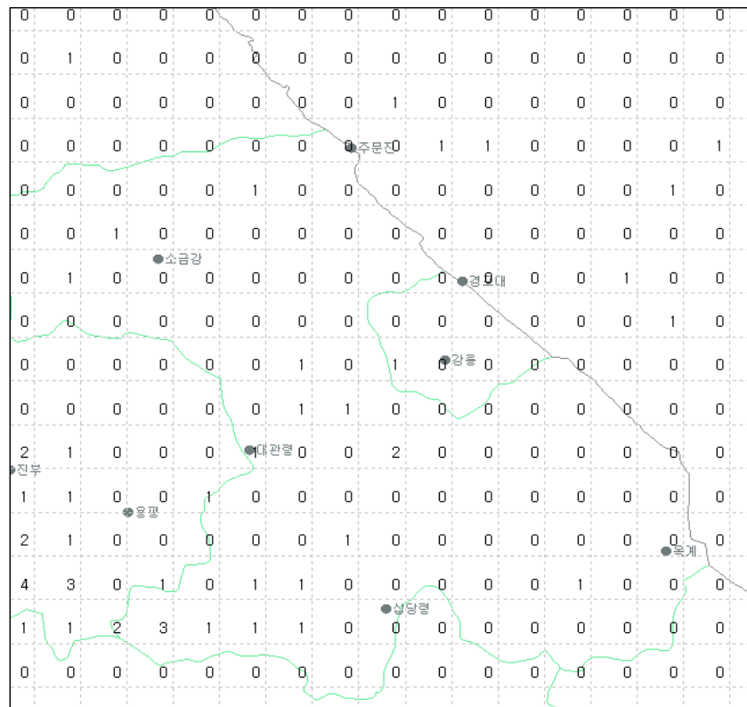
그림 23(c). 2008년 6월 강릉지역 낙뢰발생 횟수
