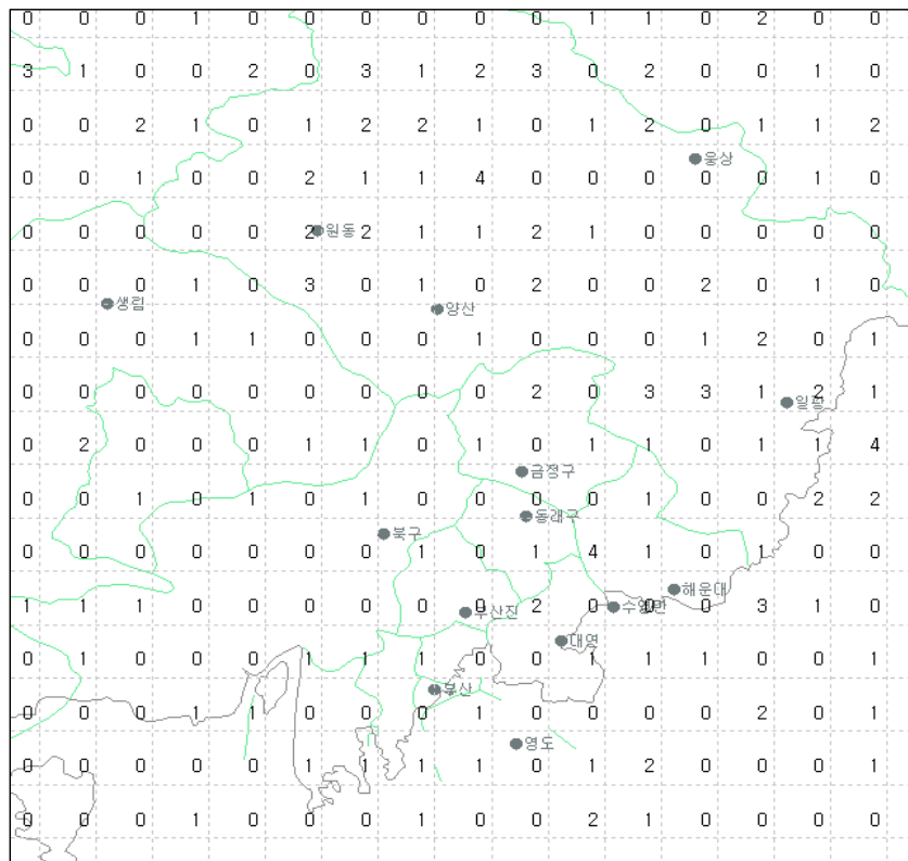
그림 19(b). 2008년 5월 부산지역 낙뢰발생 횟수
