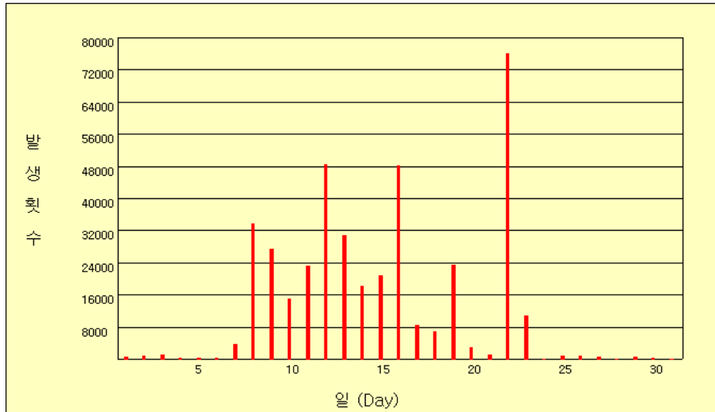
그림 37(a). 2008년 8월 일별 낙뢰발생 횟수
