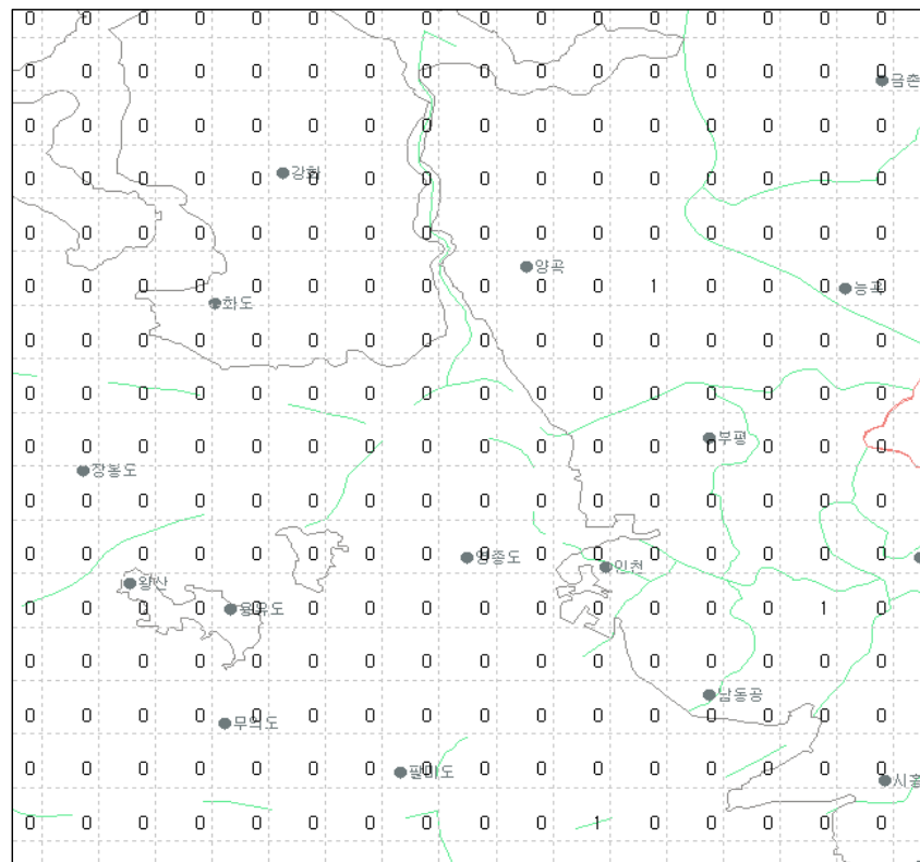
그림 22(f). 2008년 9월 인천지역 낙뢰발생 횟수
