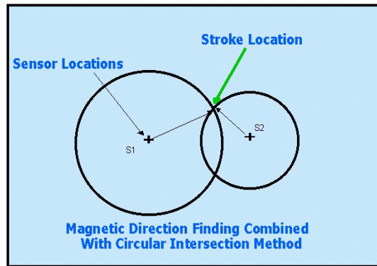
그림 8. TOA방식과 MDF방식의 합성에 의한 낙뢰위치 결정.
