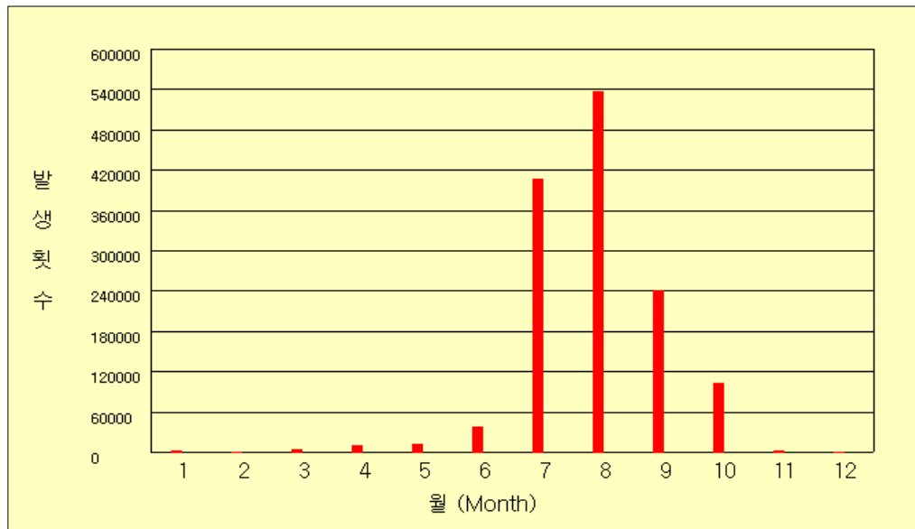
그림 47(a). 2003년 월별 낙뢰발생 횟수
