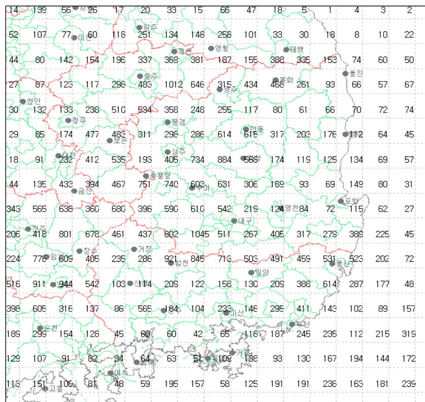
그림 27(d). 2008년 7월 경상도지역 낙뢰발생 횟수
