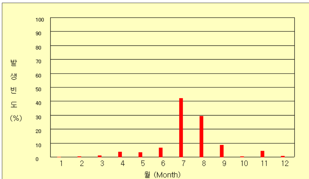
그림 47(d). 2004년 월별 낙뢰발생 횟수
