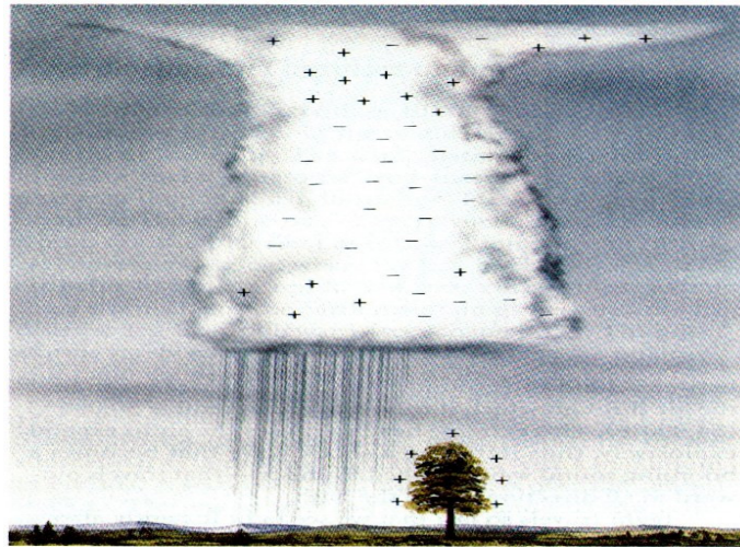
그림 2. 뇌우의 전형적인 전하 분포
