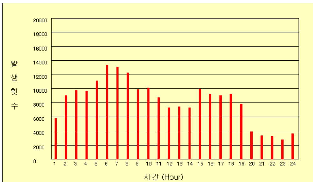
그림 36(b). 2008년 7월 시간별 낙뢰발생 횟수
