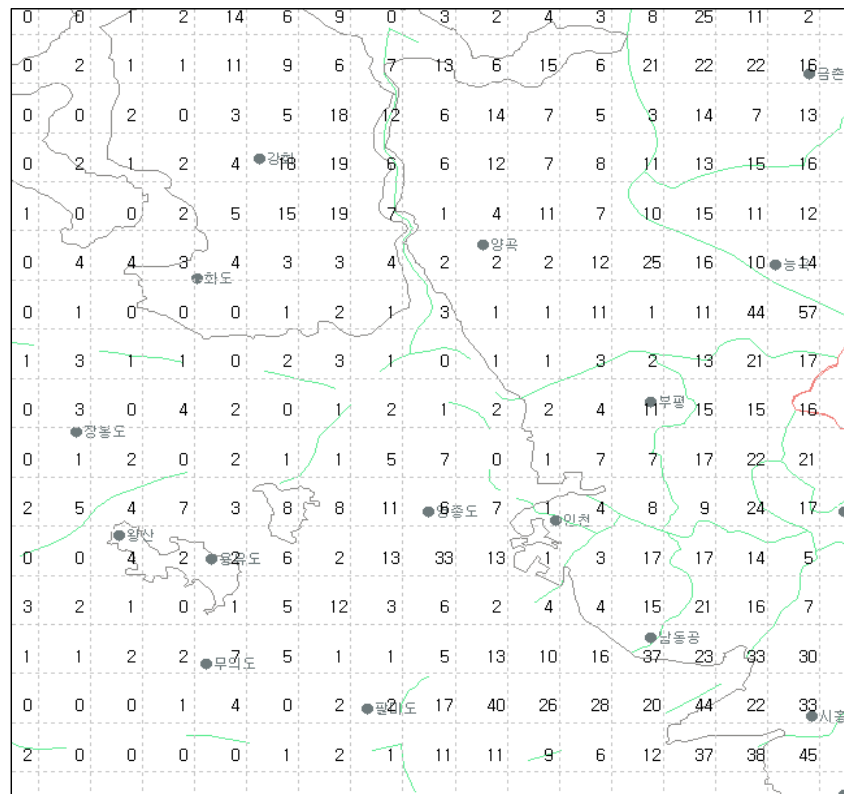
그림 22(e). 2008년 8월 인천지역 낙뢰발생 횟수
