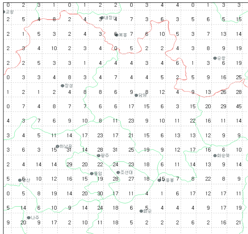
그림 21(e). 2008년 8월 광주지역 낙뢰발생 횟수
