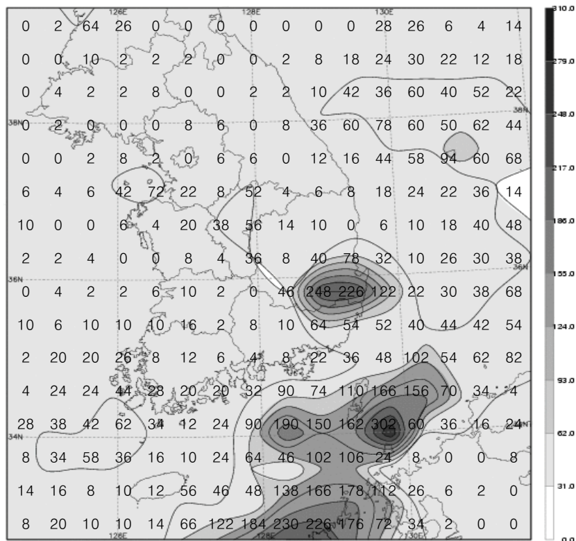
그림 16(b). 2008년 겨울철(12-2월) 낙뢰발생 횟수 분포
