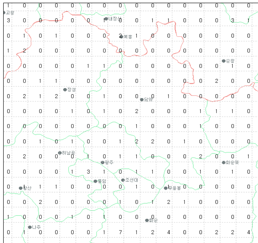
그림 21(f). 2008년 9월 광주지역 낙뢰발생 횟수
