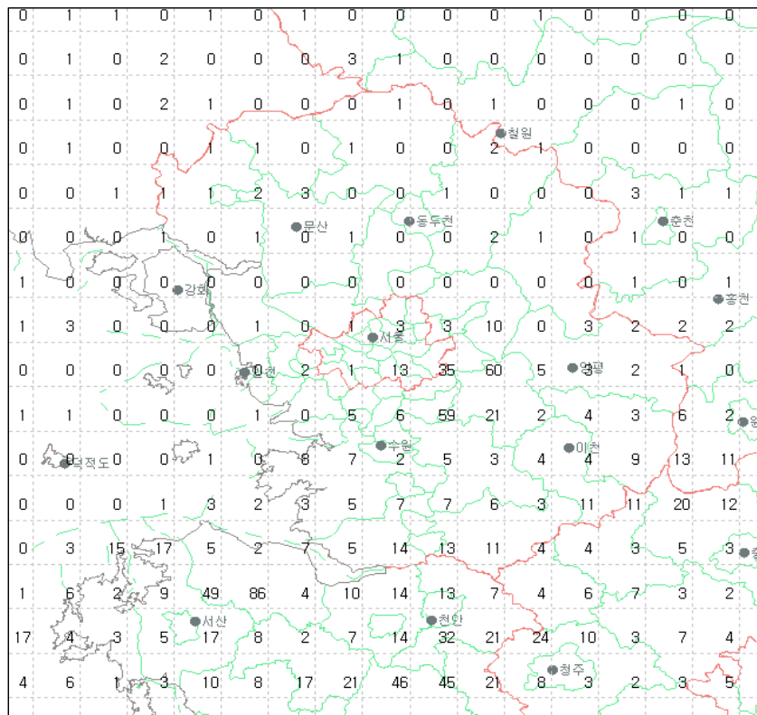
그림 24(f). 2008년 9월 경기도지역 낙뢰발생 횟수
