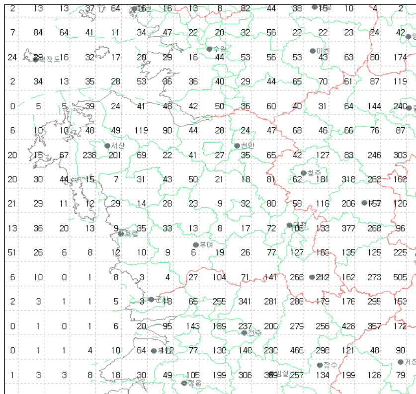
그림 26(d). 2008년 7월 충청도지역 낙뢰발생 횟수
