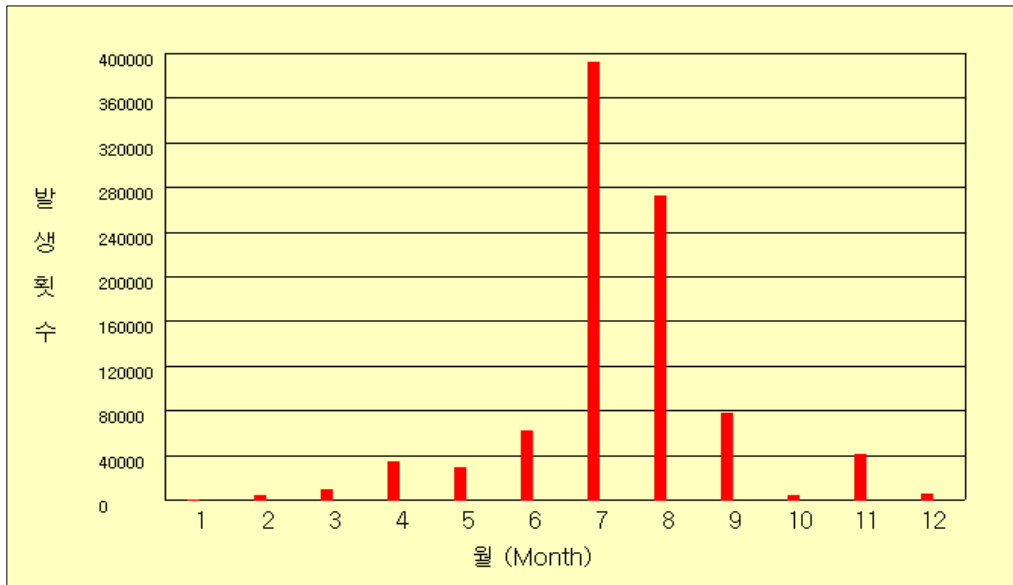
그림 47(c). 2004년 월별 낙뢰발생 횟수
