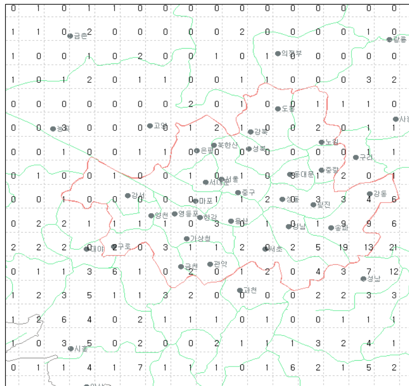
그림 18(d). 2008년 7월 서울지역 낙뢰발생 횟수
