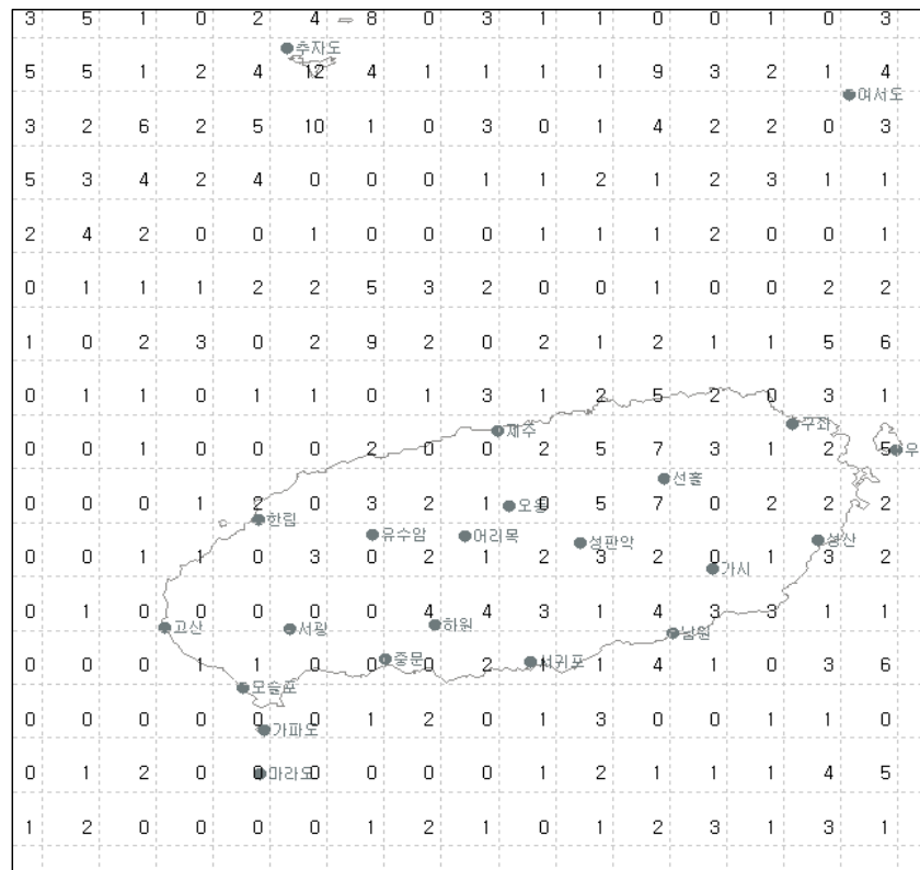
그림 29(c). 2008년 6월 제주도지역 낙뢰발생 횟수
