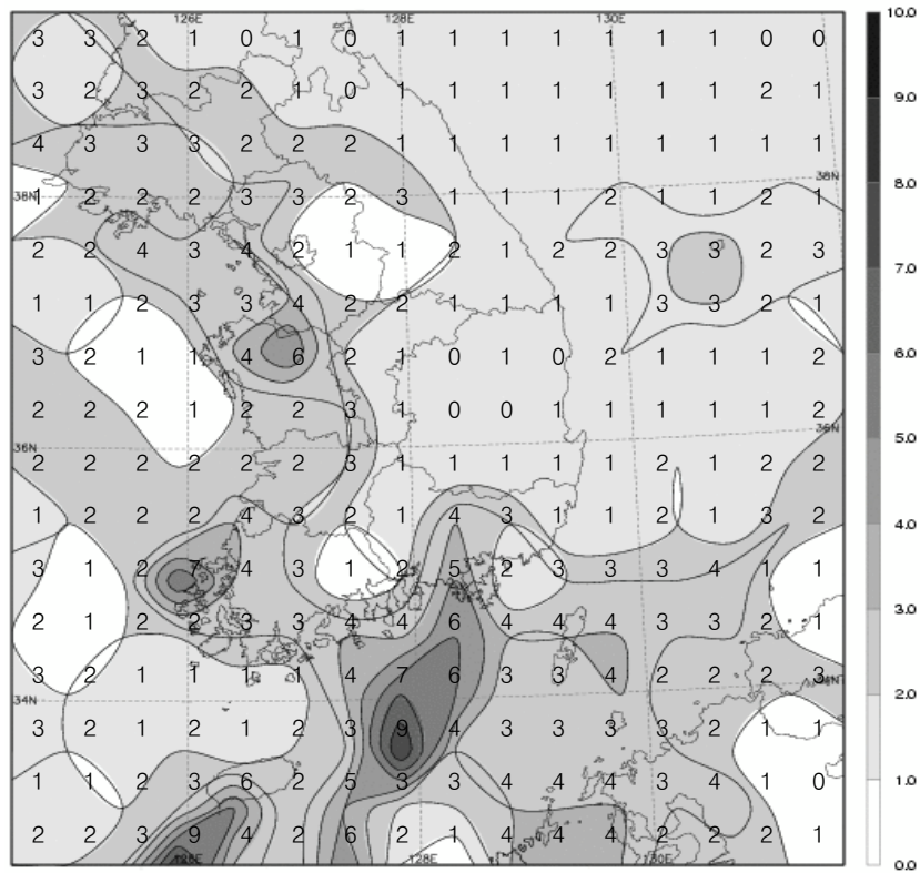
그림 4(a). 2008년 4월 낙뢰발생 일수 분포
