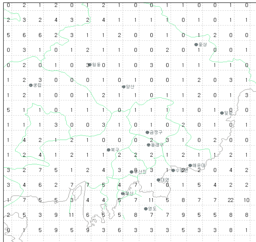
그림 19(c). 2008년 6월 부산지역 낙뢰발생 횟수
