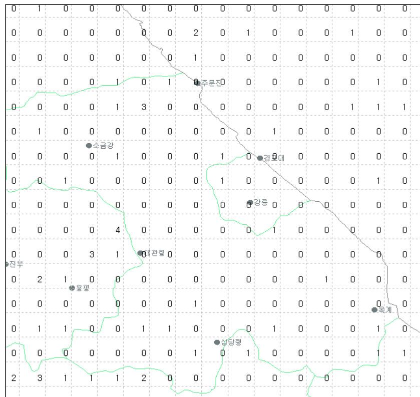
그림 23(d). 2008년 7월 강릉지역 낙뢰발생 횟수
