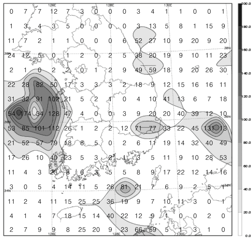
그림 11(b). 2008년 11월 낙뢰발생 횟수 분포
