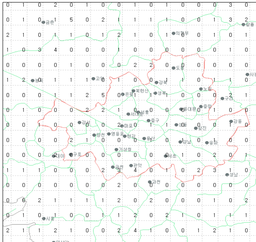
그림 18(b). 2008년 5월 서울지역 낙뢰발생 횟수
