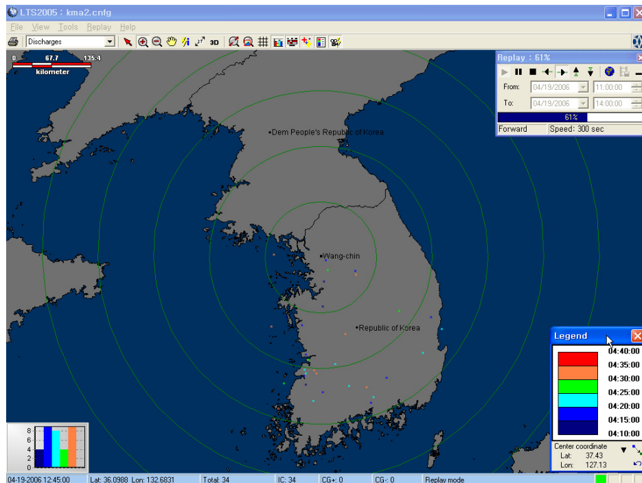
그림 14. LTS(Lightning Tracking System)의 표출 화면
