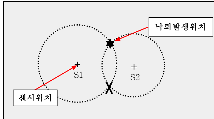
그림 5. 2개 센서를 이용한 낙뢰위치 결정(TOA)
