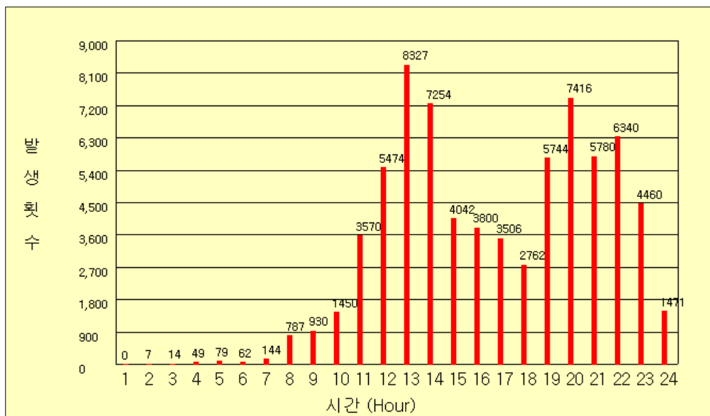
그림 54. 2008년 6월 8일 시간별 낙뢰발생 횟수 분포
