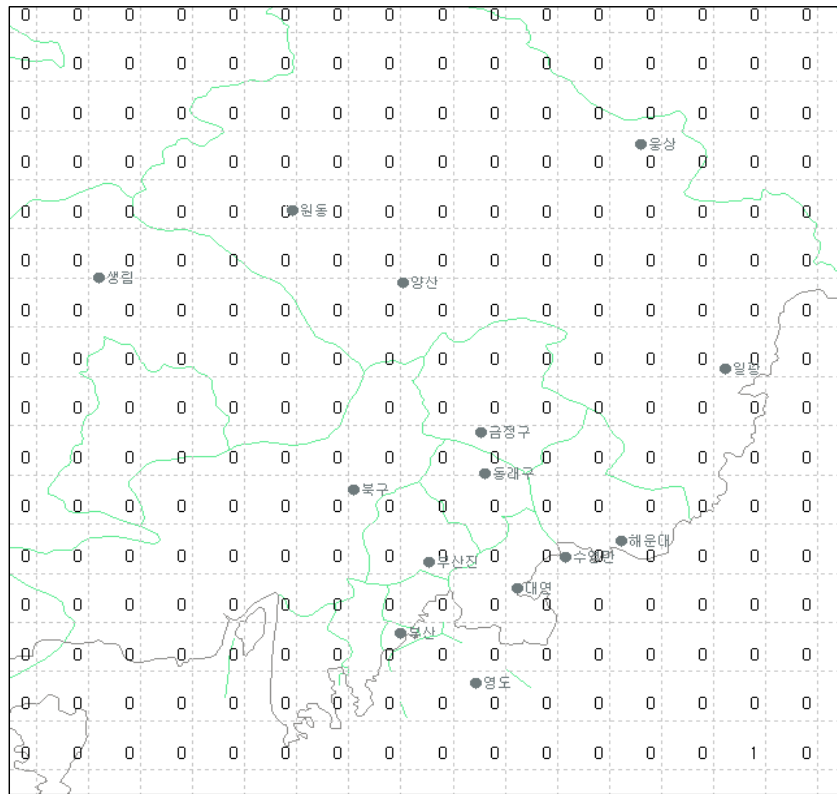
그림 19(a). 2008년 4월 부산지역 낙뢰발생 횟수
