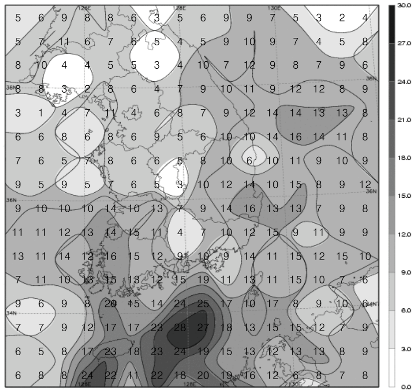
그림 15(a). 2008년 가을철(9-11월) 낙뢰발생 일수 분포
