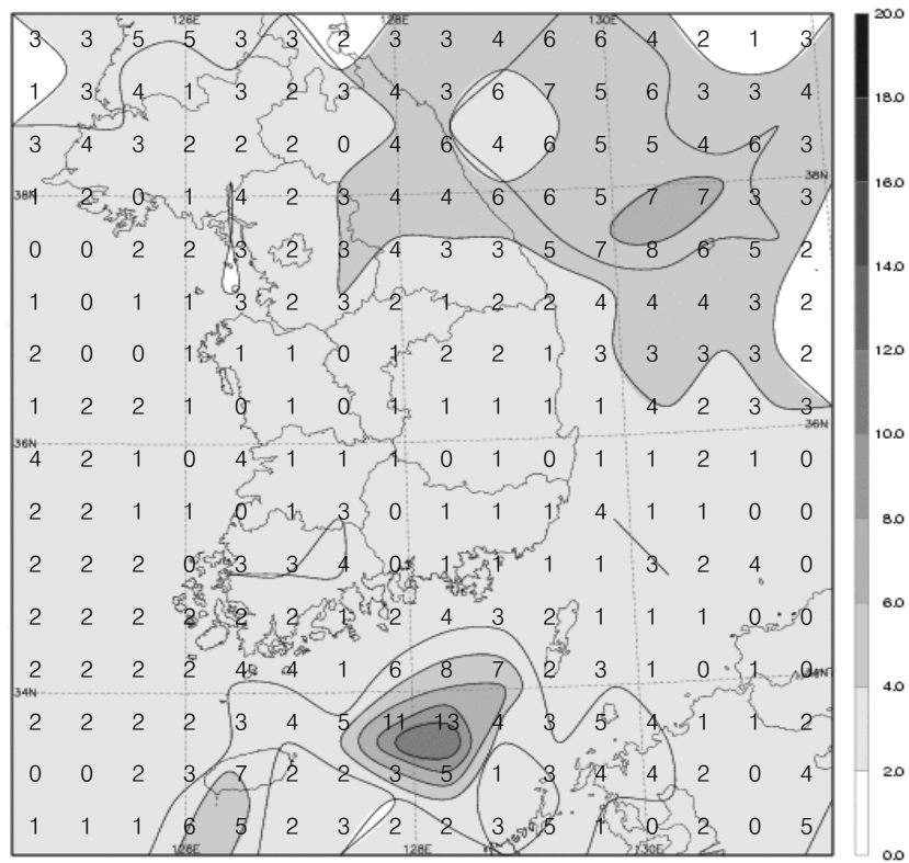
그림 10(a). 2008년 10월 낙뢰발생 일수 분포
