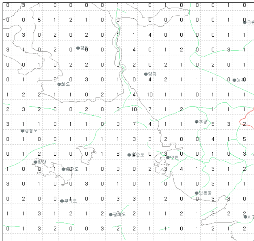
그림 22(c). 2008년 6월 인천지역 낙뢰발생 횟수
