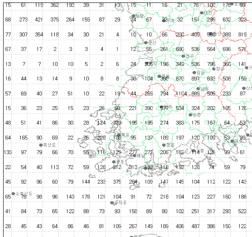
그림 28(d). 2008년 7월 전라도지역 낙뢰발생 횟수
