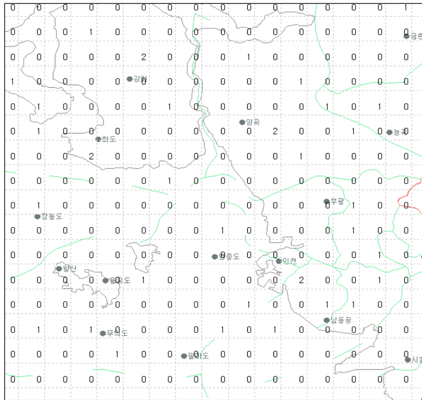
그림 22(a). 2008년 4월 인천지역 낙뢰발생 횟수
