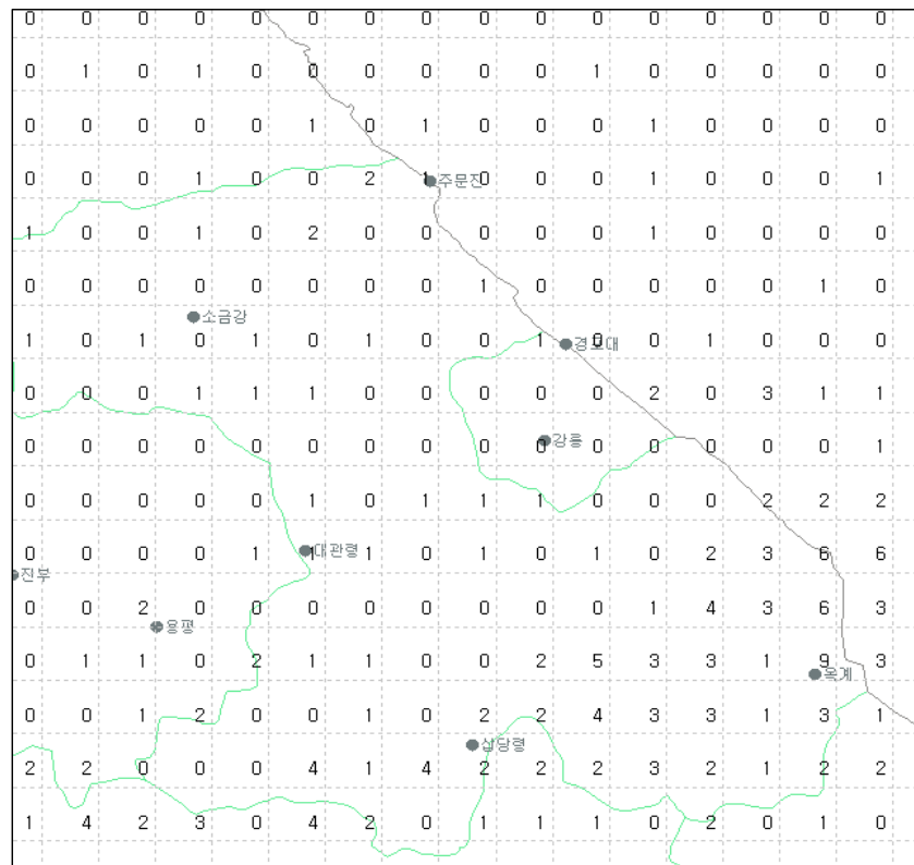
그림 23(e). 2008년 8월 강릉지역 낙뢰발생 횟수
