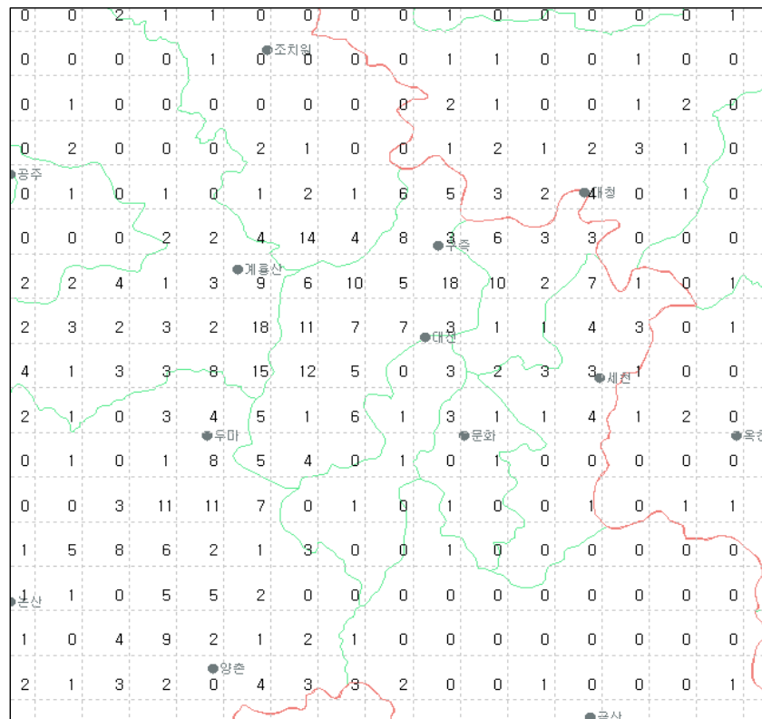
그림 20(f). 2008년 9월 대전지역 낙뢰발생 횟수
