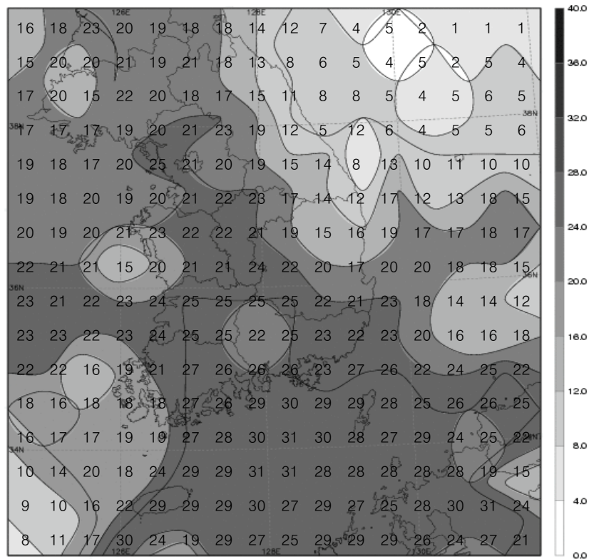
그림 14(a). 2008년 여름철(6-8월) 낙뢰발생 일수 분포
