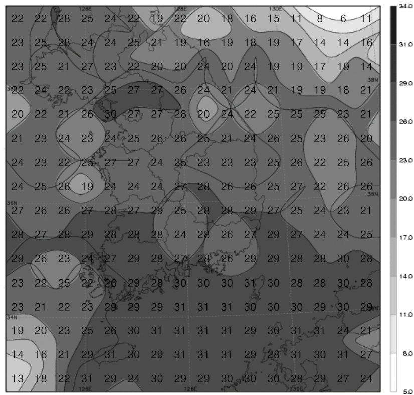
그림 17(a). 2008년 낙뢰발생 일수 분포
