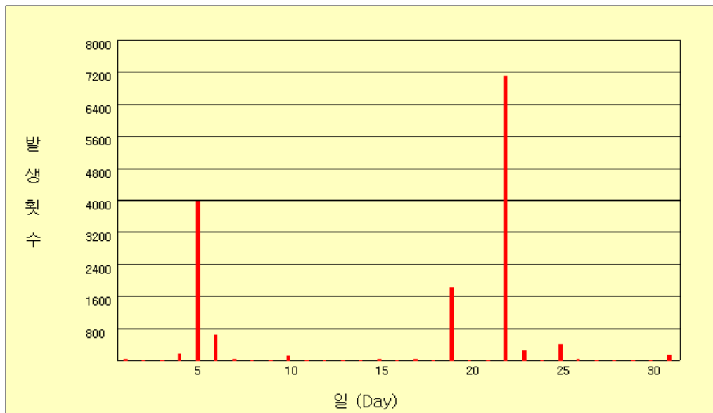
그림 39(a). 2008년 10월 일별 낙뢰발생 횟수
