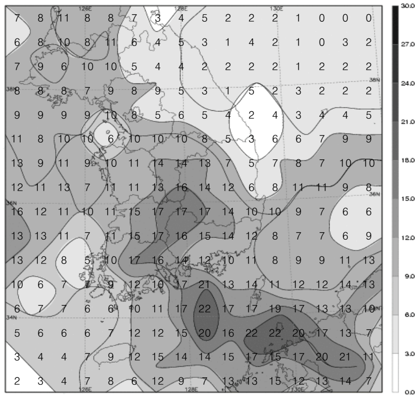
그림 7(a). 2008년 7월 낙뢰발생 일수 분포
