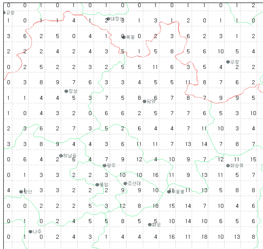
그림 21(c). 2008년 6월 광주지역 낙뢰발생 횟수
