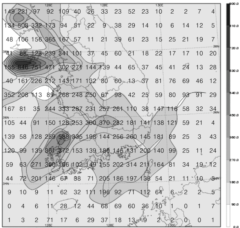
그림 5(b). 2008년 5월 낙뢰발생 횟수 분포
