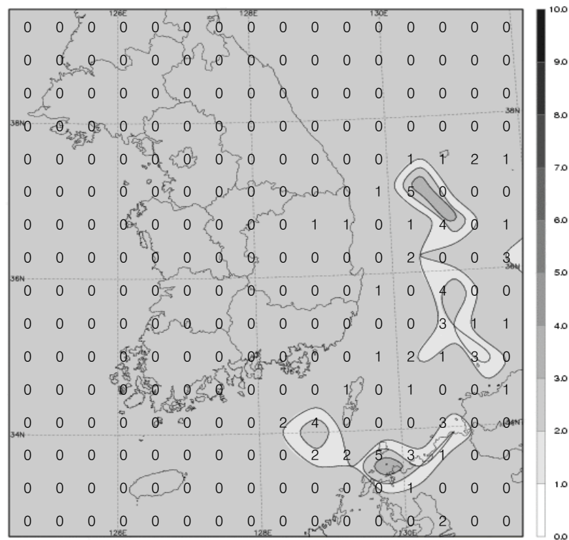
그림 2(b). 2008년 2월 낙뢰발생 횟수 분포
