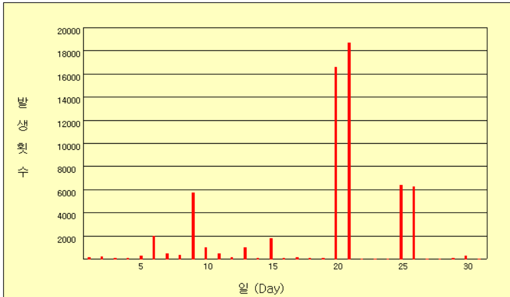
그림 38(a). 2008년 9월 일별 낙뢰발생 횟수
