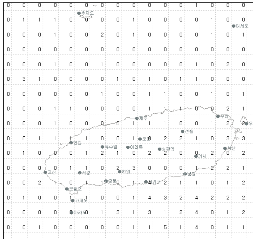
그림 29(a). 2008년 4월 제주도지역 낙뢰발생 횟수
