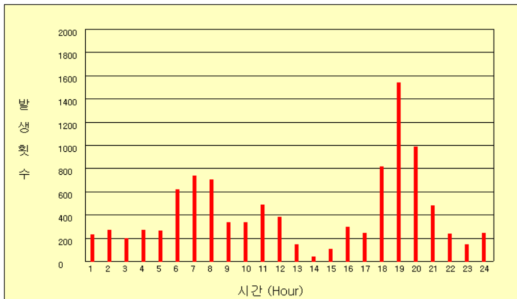
그림 33(b). 2008년 4월 시간별 낙뢰발생 횟수
