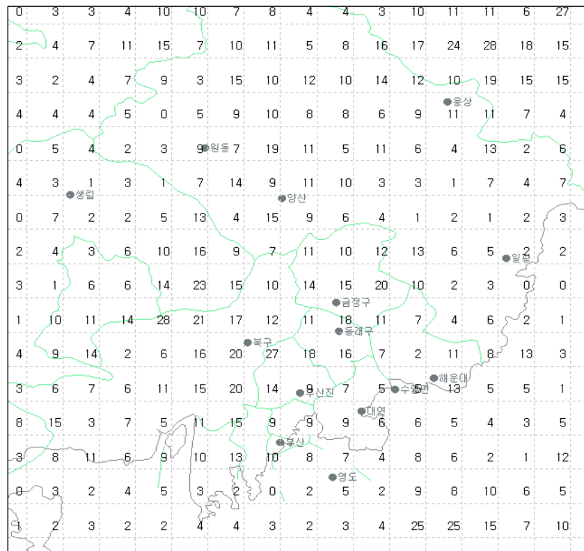
그림 19(d). 2008년 7월 부산지역 낙뢰발생 횟수
