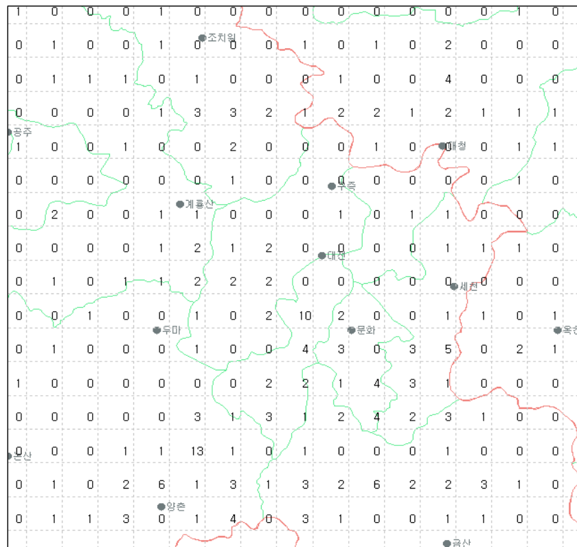
그림 20(b). 2008년 5월 대전지역 낙뢰발생 횟수
