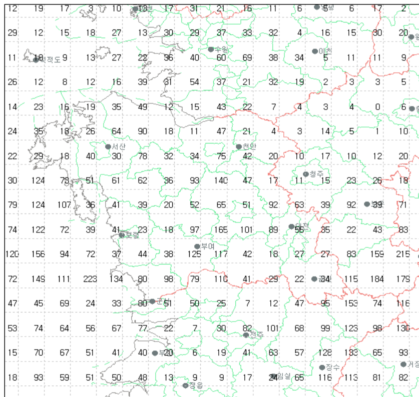
그림 26(c). 2008년 6월 충청도지역 낙뢰발생 횟수
