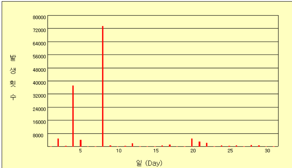
그림 35(a). 2008년 6월 일별 낙뢰발생 횟수
