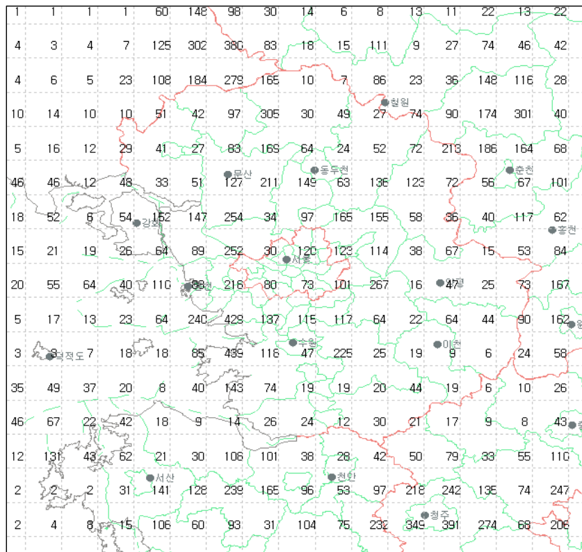
그림 24(e). 2008년 8월 경기도지역 낙뢰발생 횟수
