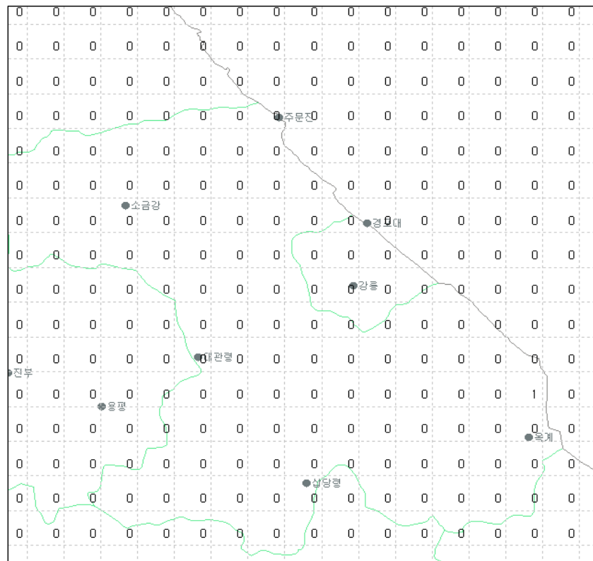
그림 23(a). 2008년 4월 강릉지역 낙뢰발생 횟수
