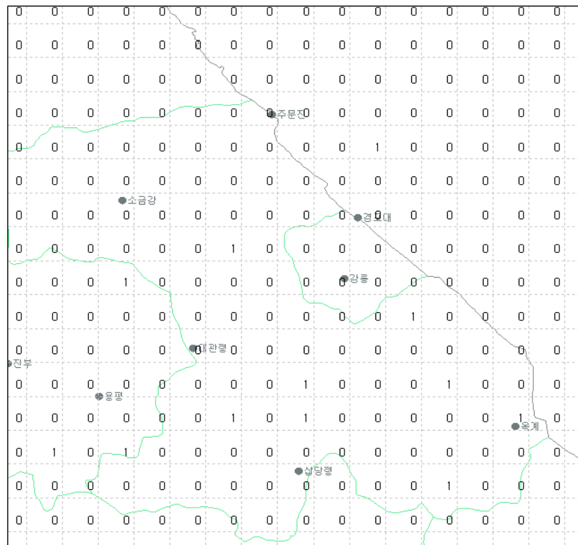
그림 23(f). 2008년 9월 강릉지역 낙뢰발생 횟수
