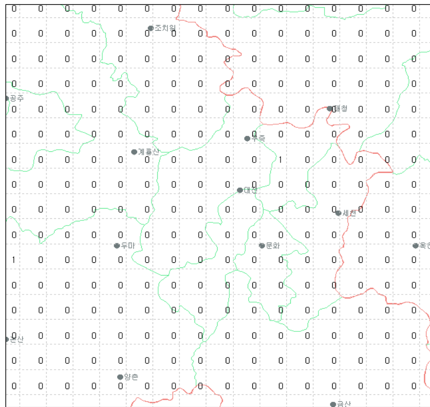
그림 20(a). 2008년 4월 대전지역 낙뢰발생 횟수
