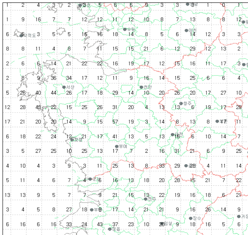
그림 26(b). 2008년 5월 충청도지역 낙뢰발생 횟수
