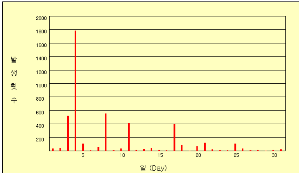
그림 41(a). 2008년 12월 일별 낙뢰발생 횟수
