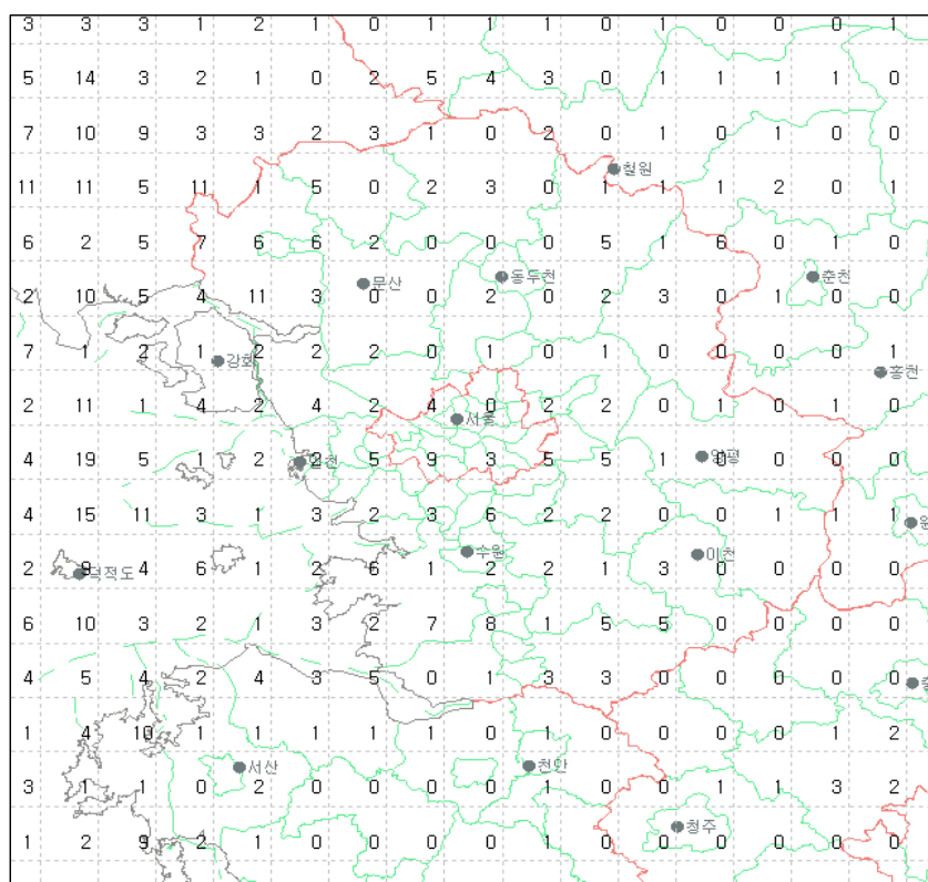
그림 24(a). 2008년 4월 경기도지역 낙뢰발생 횟수
