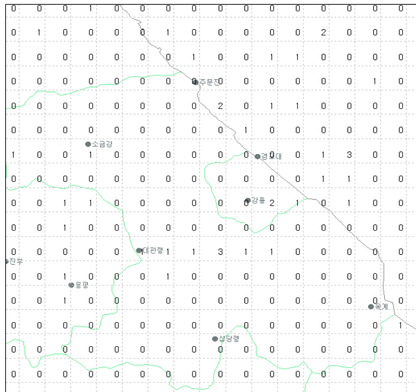
그림 23(b). 2008년 5월 강릉지역 낙뢰발생 횟수
