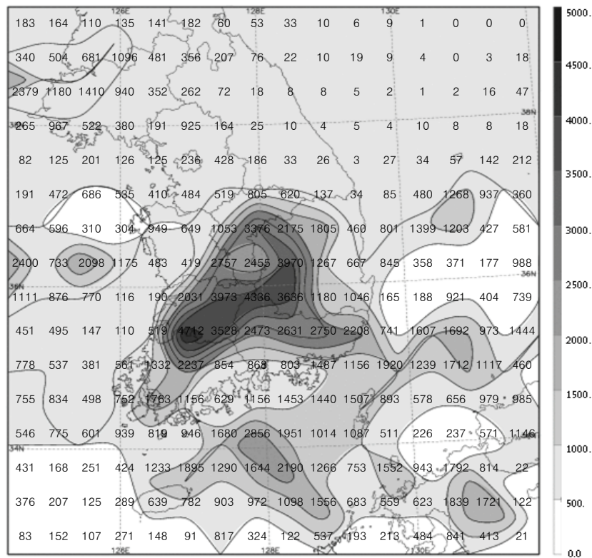
그림 7(b). 2008년 7월 낙뢰발생 횟수 분포
