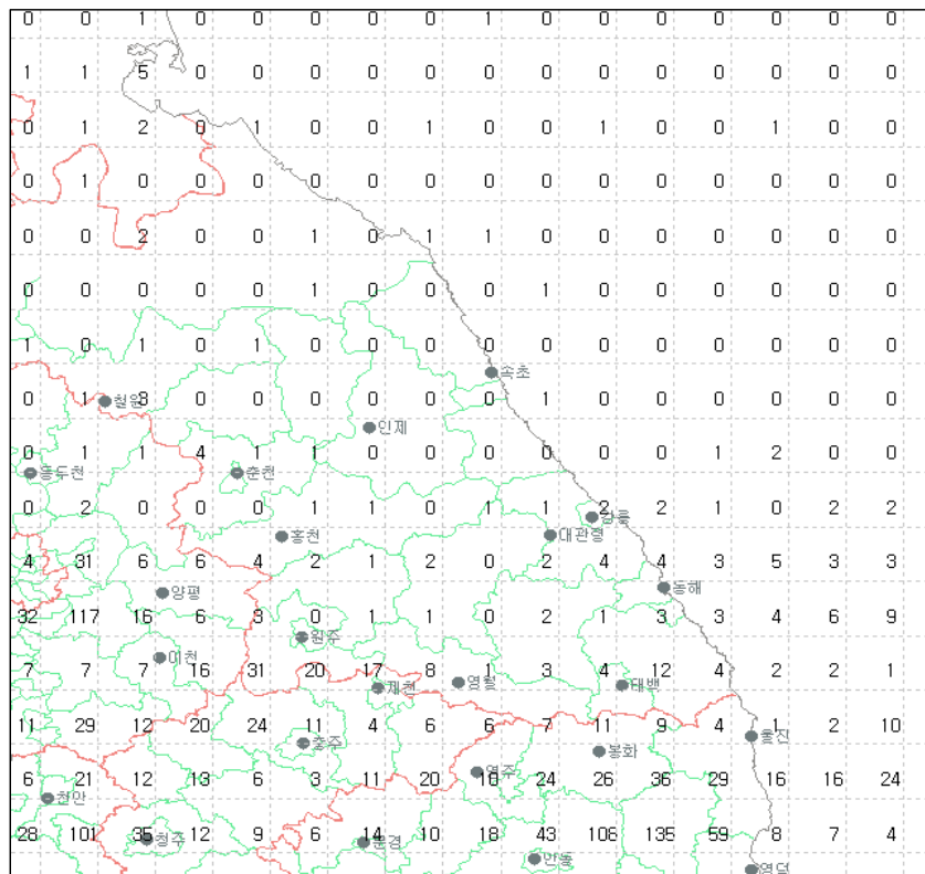
그림 25(f). 2008년 9월 강원도지역 낙뢰발생 횟수
