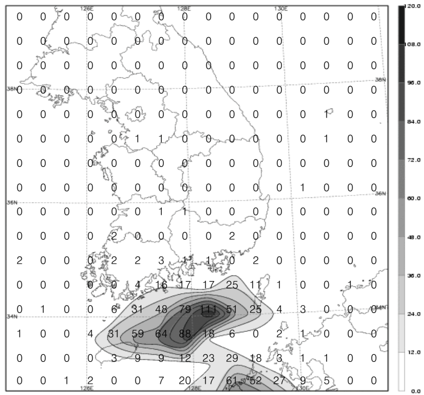
그림 1(b). 2008년 1월 낙뢰발생 횟수 분포
