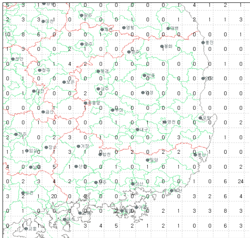
그림 27(a). 2008년 4월 경상도지역 낙뢰발생 횟수
