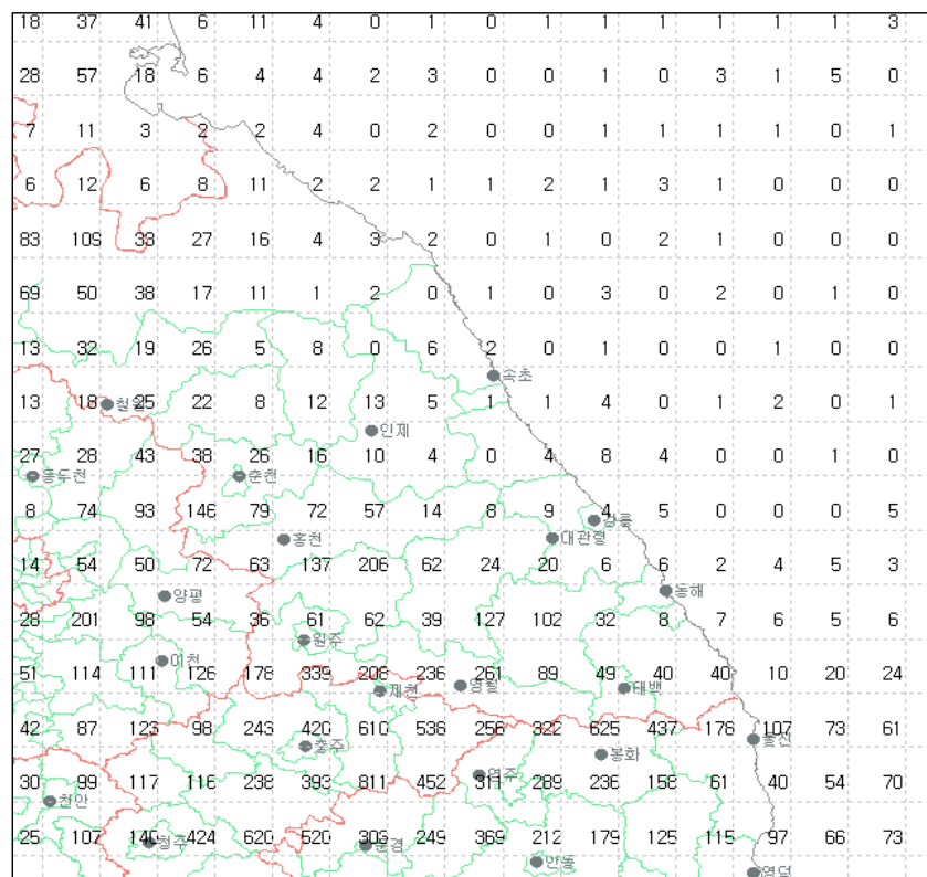
그림 25(d). 2008년 7월 강원도지역 낙뢰발생 횟수
