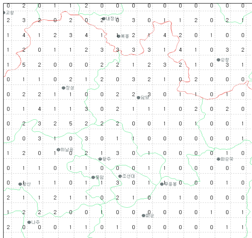
그림 21(b). 2008년 5월 광주지역 낙뢰발생 횟수
