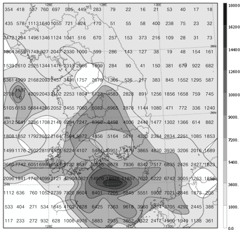
그림 14(b). 2008년 여름철(6-8월) 낙뢰발생 횟수 분포
