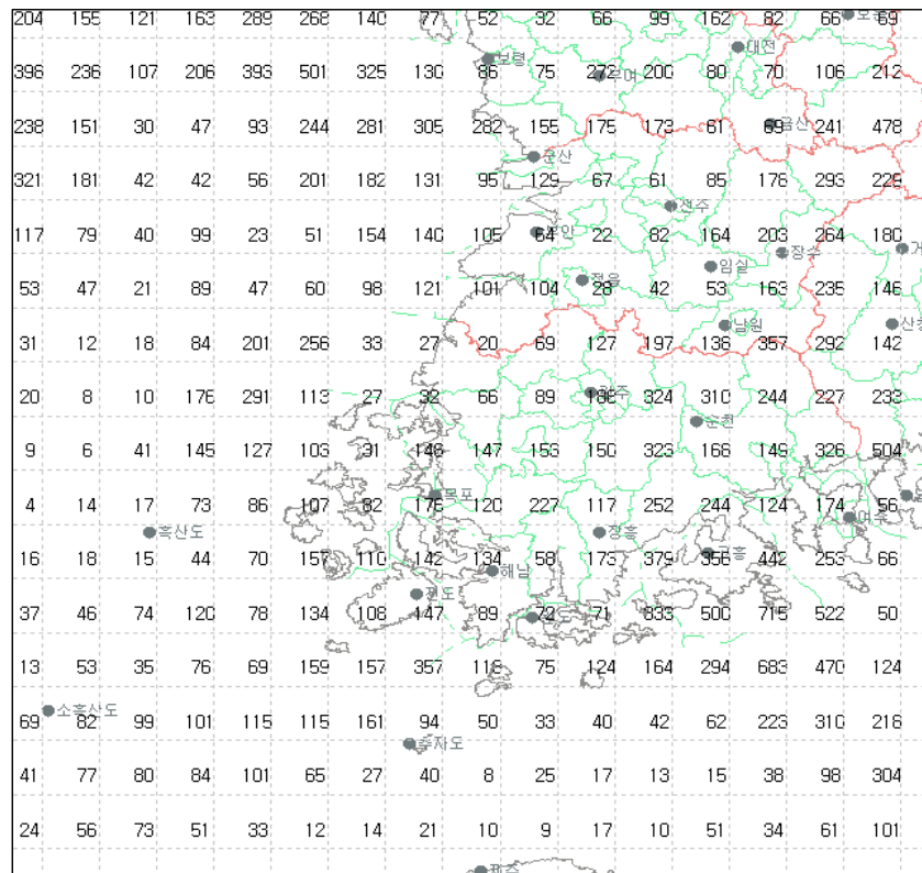
그림 28(c). 2008년 6월 전라도지역 낙뢰발생 횟수
