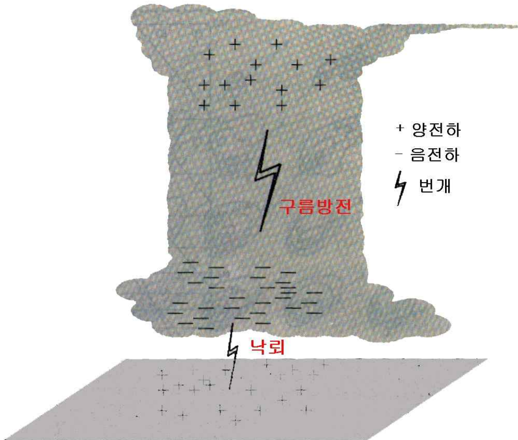
<그림 1.1> 적란운에서의 구름방전과 낙뢰(대지방전) 개념도
