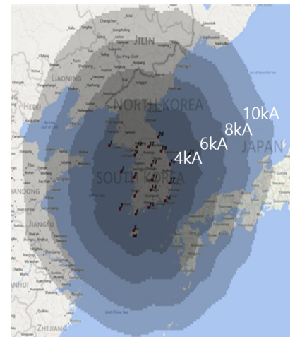
〈낙뢰관측범위〉
