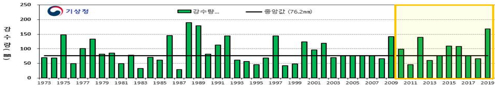
[그림 9] 연도별(1973년~2019년) 전국 강수량(12월~2월)
