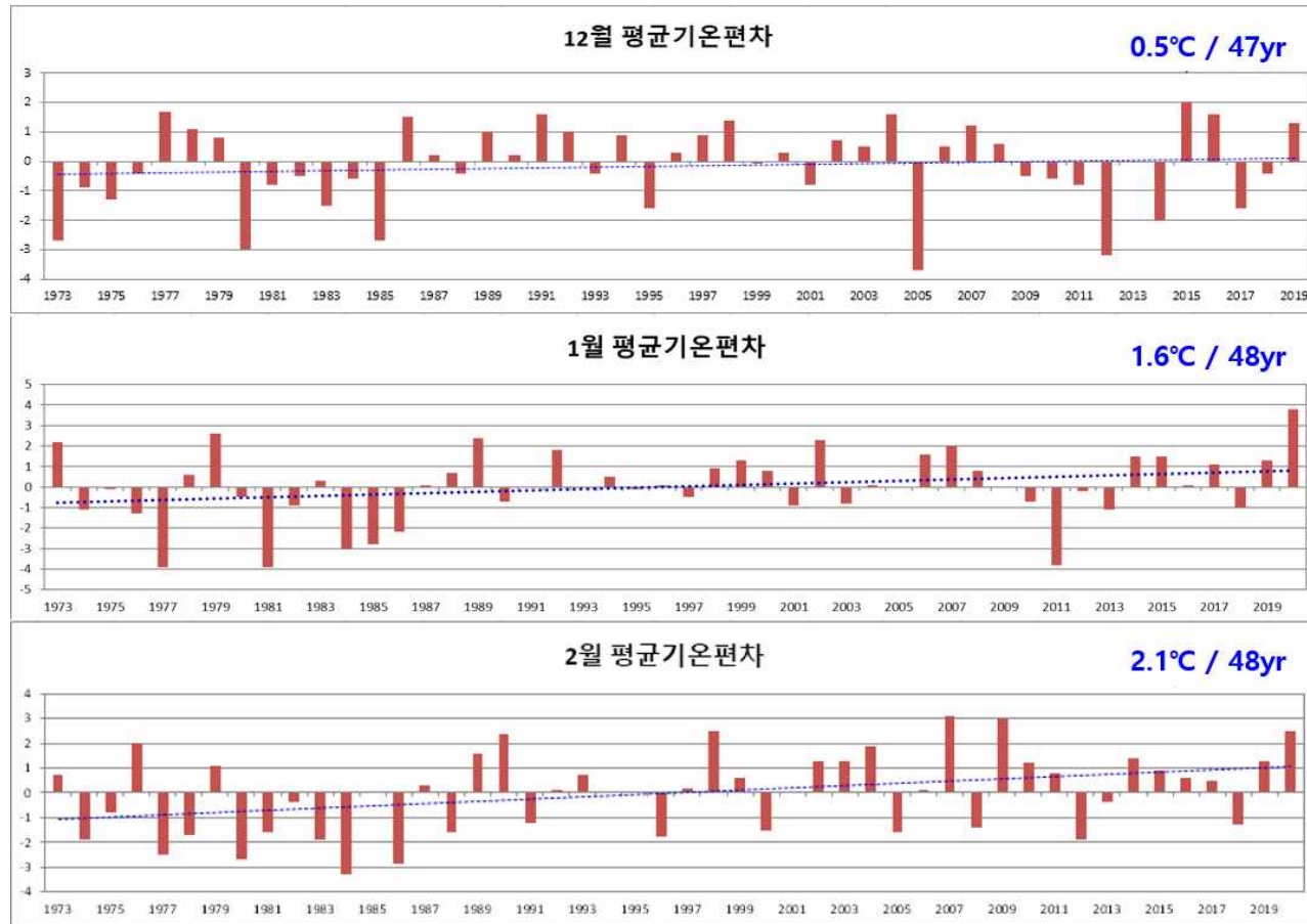
[그림 7] 월 평균기온 경향성(Trend) 분석
