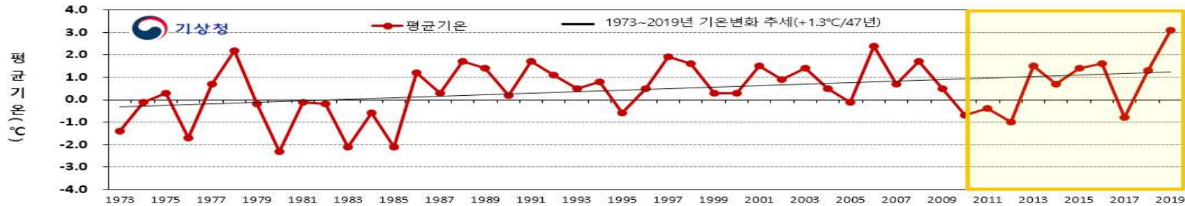
[그림 8] 연도별(1973년~2019년) 전국 평균 기온(12월~2월)
