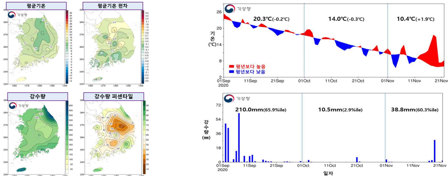
[그림 1] 가을철 전국 (위) 평균기온과 편차(°C) 분포도 및 일변화 시계열, (아래) 강수량(mm)과 강수량 퍼센타일) 분포도 및 일변화 시계열
