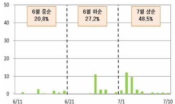
그림 4. 대구·경북 강수량의 일변화(6.11~7.10)
