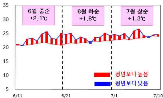
그림 3. 대구·경북 평균기온의 일변화(6.11~7.10)
