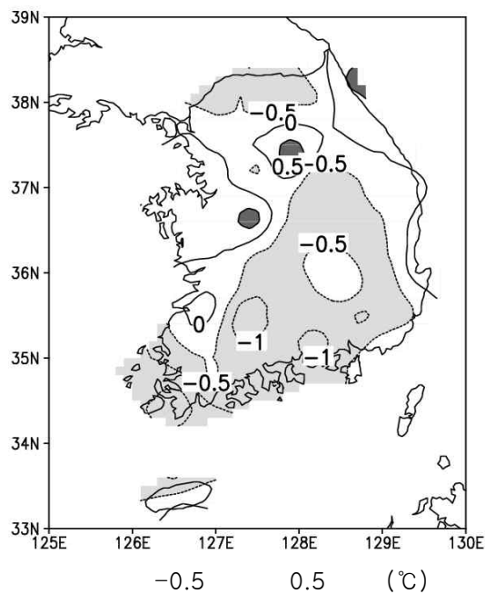
기온 편차(°C)
