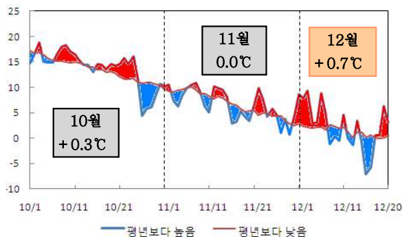
최근 평균기온의 일변화(10.1~12.20)
