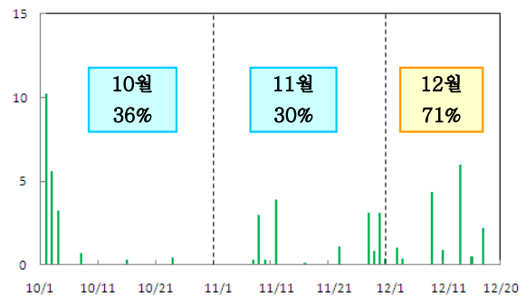
최근 강수량의 일변화(10.1~12.20)
