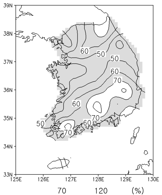
강수량 평년비(%)
