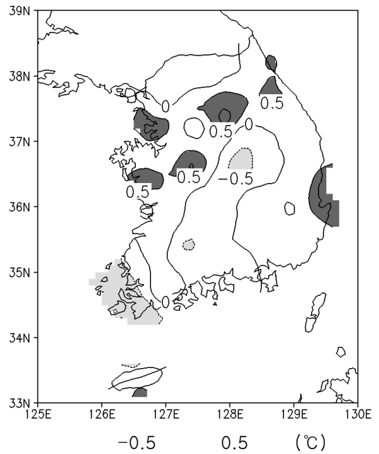
기온 편차(°C)
