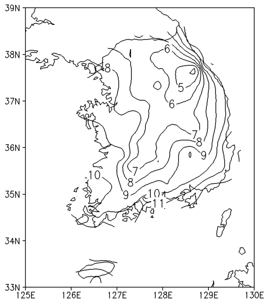
기온(°C)
