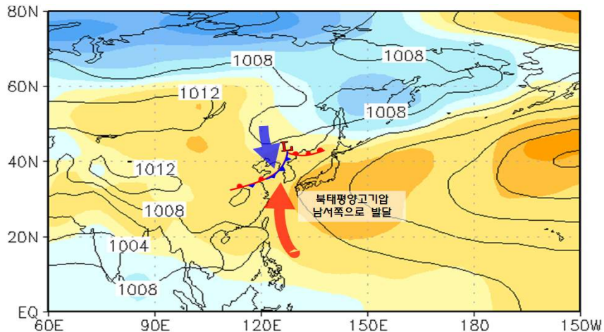
그림 6. 8월 평균 해면기압(실선) 및 해면기압편차(음영)와 기압계 모식도
