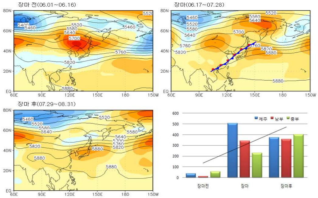
그림 5. 장마기간 전후의 500hPa 평균 고도장(실선) 및 편차장(음영)과 강수량 비교
