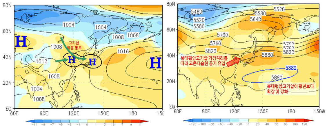
그림 4. (좌) 6월 평균 해면기압(실선) 및 해면기압편차(음영)과 (우) 7-8월 500hPa 평균 고도장(실선, 검정:2010년, 파랑:평년) 및 편차장(음영, 붉은색:고기압 발달, 파랑색:저기압 발달)
