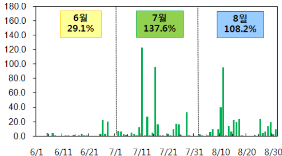
그림 2. (좌)부산·울산·경남 강수량 일변화(mm) (우)금년 여름 강수량 평년비 분포도(%)
