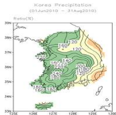
그림 2. (좌)부산·울산·경남 강수량 일변화(mm) (우)금년 여름 강수량 평년비 분포도(%)
