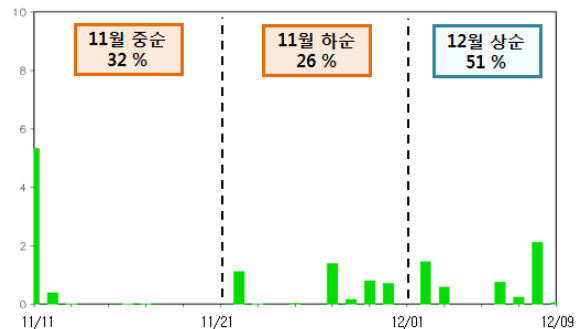
그림 2. 전국 강수량의 일변화(11.11~12.09)
