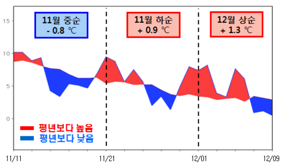
그림 1. 전국 평균기온의 일변화(11.11~12.09)
