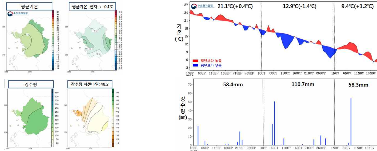
[그림 1] 가을철 수도권 (위) 평균기온과 편차(°C) 분포도 및 일변화 시계열, (아래) 강수량(mm)과 강수량 퍼센타일 1) 분포도 및 일변화 시계열
