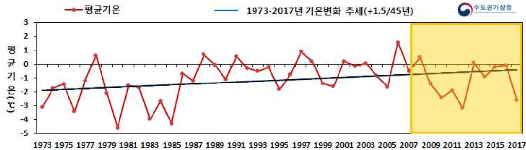
[그림 7] 연도별(1973~2017년) 겨울철 수도권 평균기온(12월~이듬해 2월)
