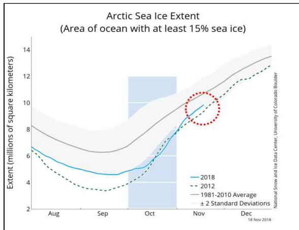
[그림 3] (왼쪽) 북극 해빙면적 시계열, (가운데) 10월 해빙 분포 및 편차, (오른쪽) 최근 현황
