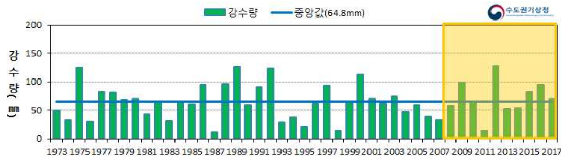
[그림 8] 연도별(1973~2017년) 겨울철 수도권 강수량(12월~이듬해 2월)
