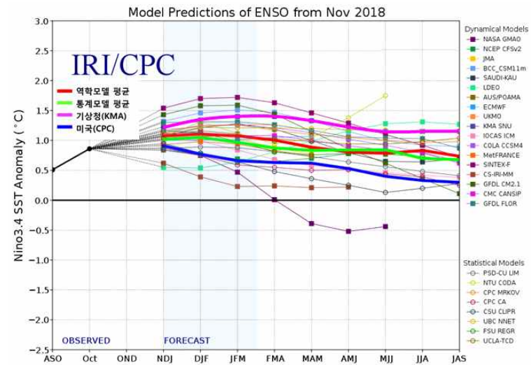
[그림 2] (왼쪽) 엘니뇨·라니냐 감시구역의 최근(11.11.~11.17.) 해수면온도 편차(OISSTv2), (오른쪽) 세계 각국의 엘니뇨·라니냐 예측 결과(출처 : IRI)
