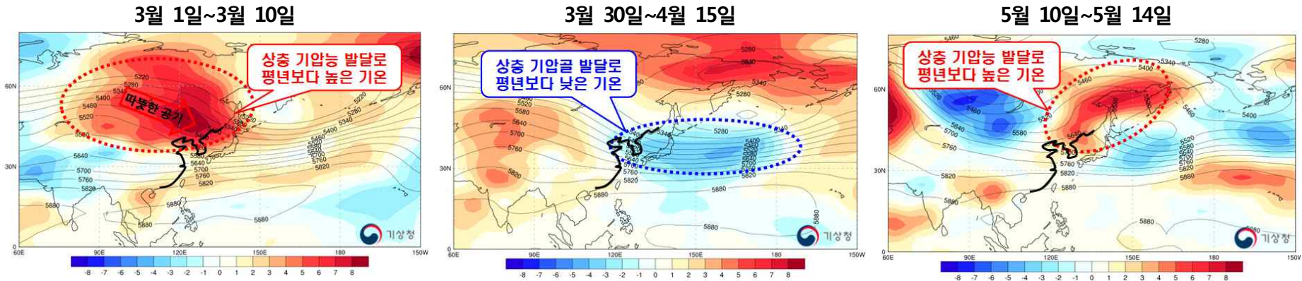
[그림 2] 500hPa(약 5.5km 상공) 지위고도(실선)와 850hPa(약 1.5km 상공) 기온 편차(채색)
