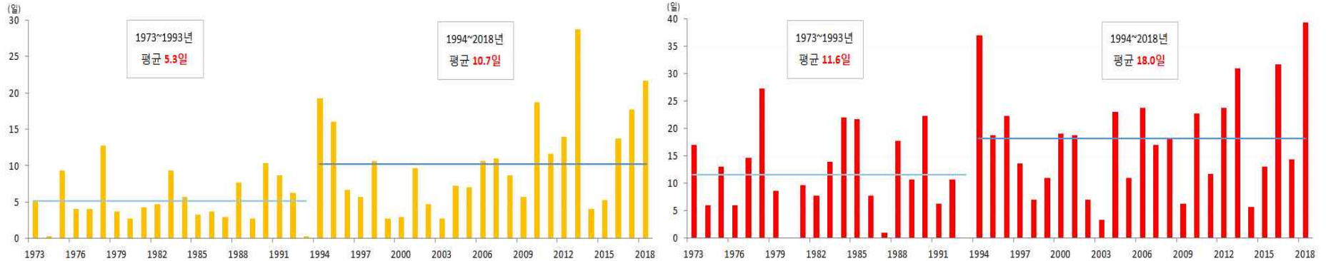
[그림 14] 전북 3개 지점 1973년 이후 (왼쪽) 연도별 열대야 일수, (오른쪽) 연도별 폭염 일수
