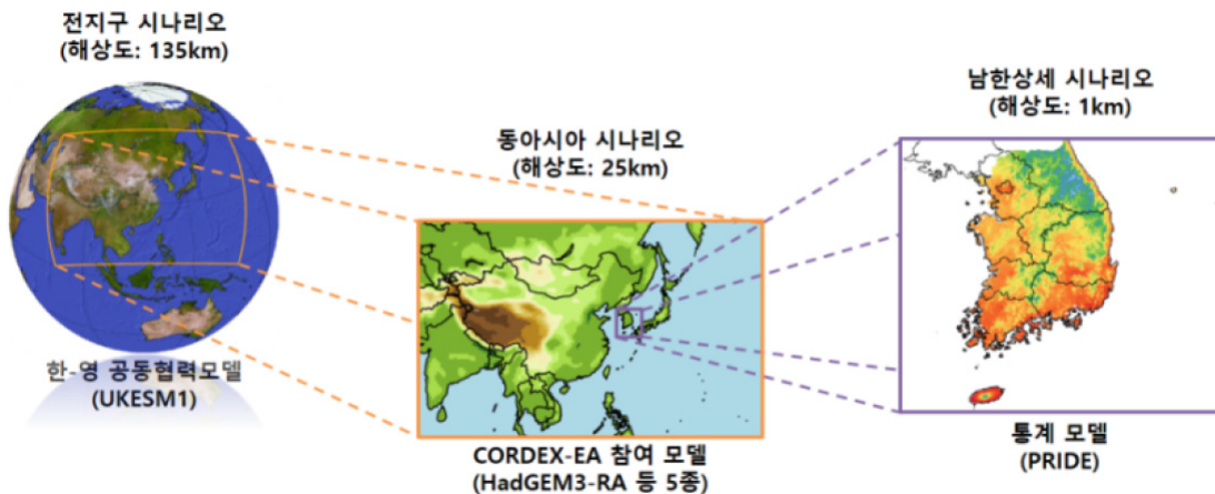
그림 1-2. SSP 기후변화 시나리오 생산체계(전지구→동아시아·한반도→남한상세)
