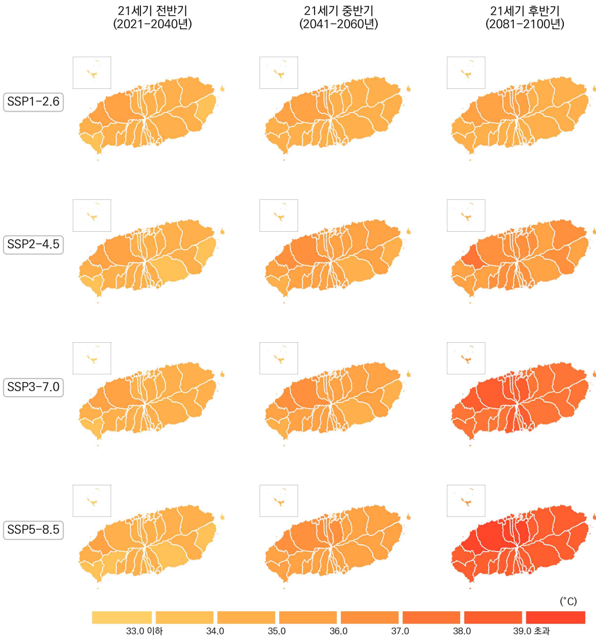
그림 4-23. 제주특별자치도의 일최고기온 연최대(°C) 전망 분포도
