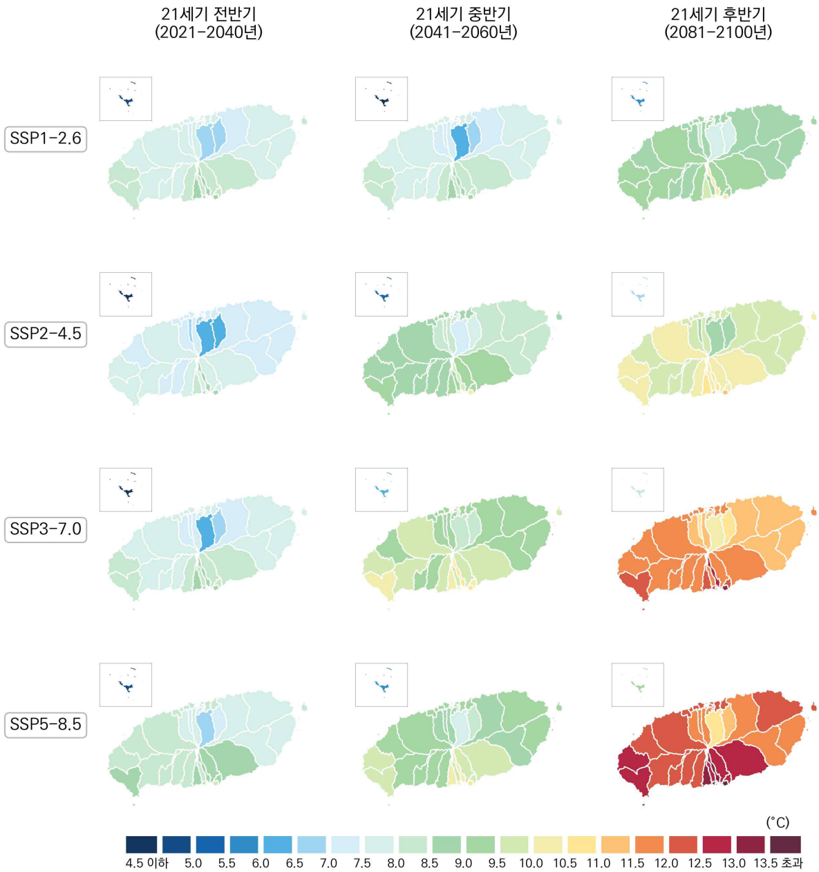
그림 4-5. 제주특별자치도의 겨울철 연평균기온(°C) 전망 분포도
