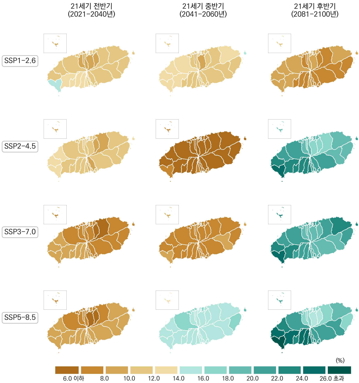
그림 4-17. 제주특별자치도의 연강수량 변화율(2000-2019년 대비) 전망 분포도
