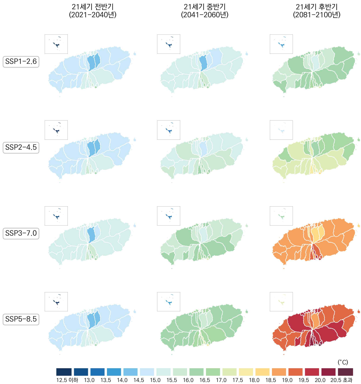
그림 4-2. 제주특별자치도의 봄철 연평균기온(°C) 전망 분포도
