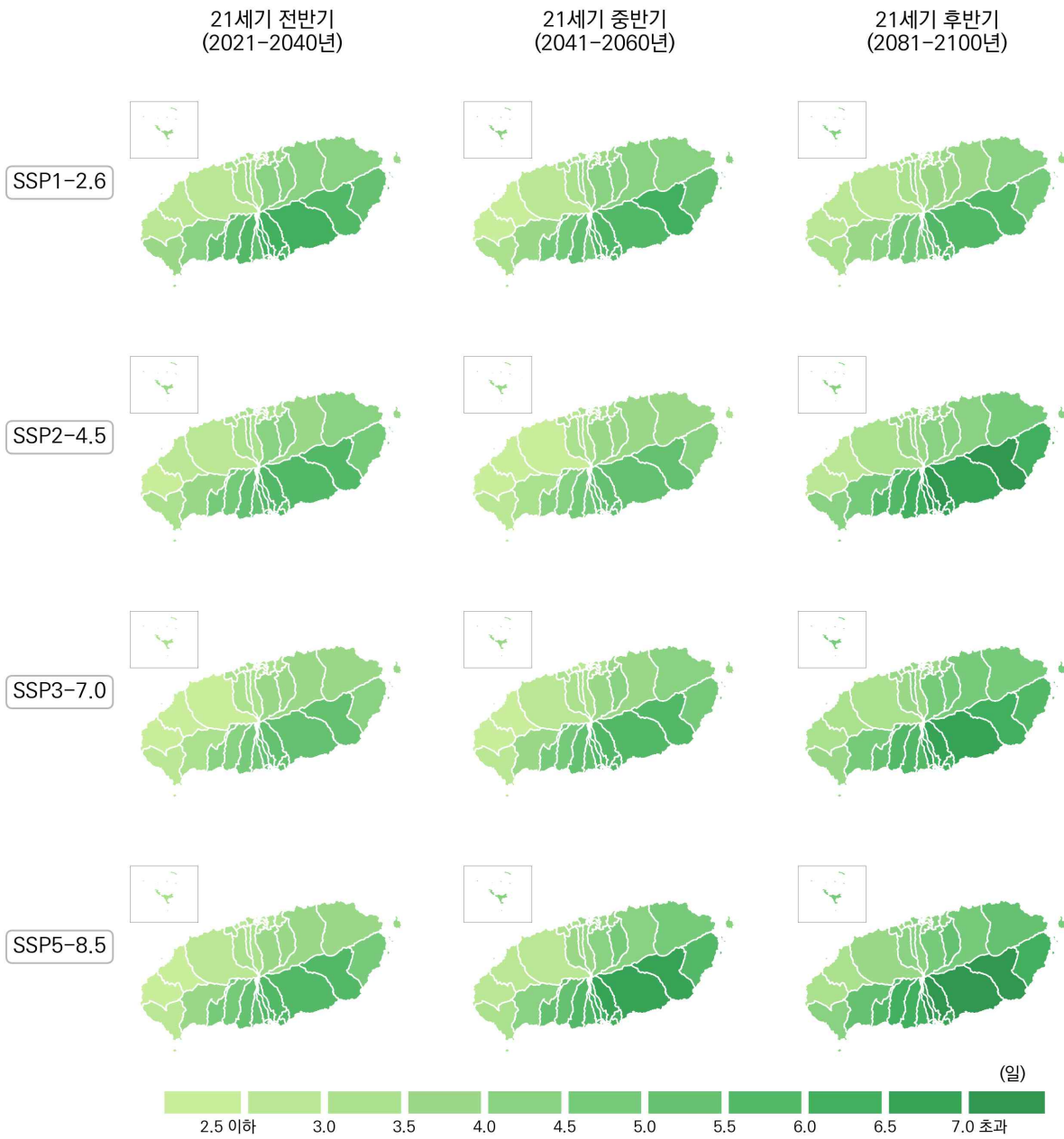
그림 4-34. 제주특별자치도의 호우일수(일) 전망 분포도
