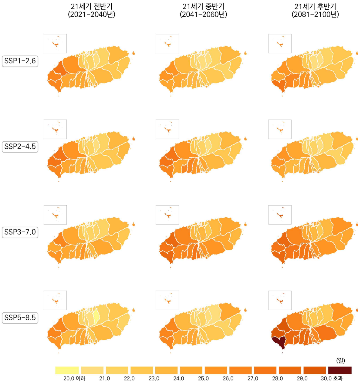
그림 4-40. 제주특별자치도의 최대무강수지속기간(일) 전망 분포도
