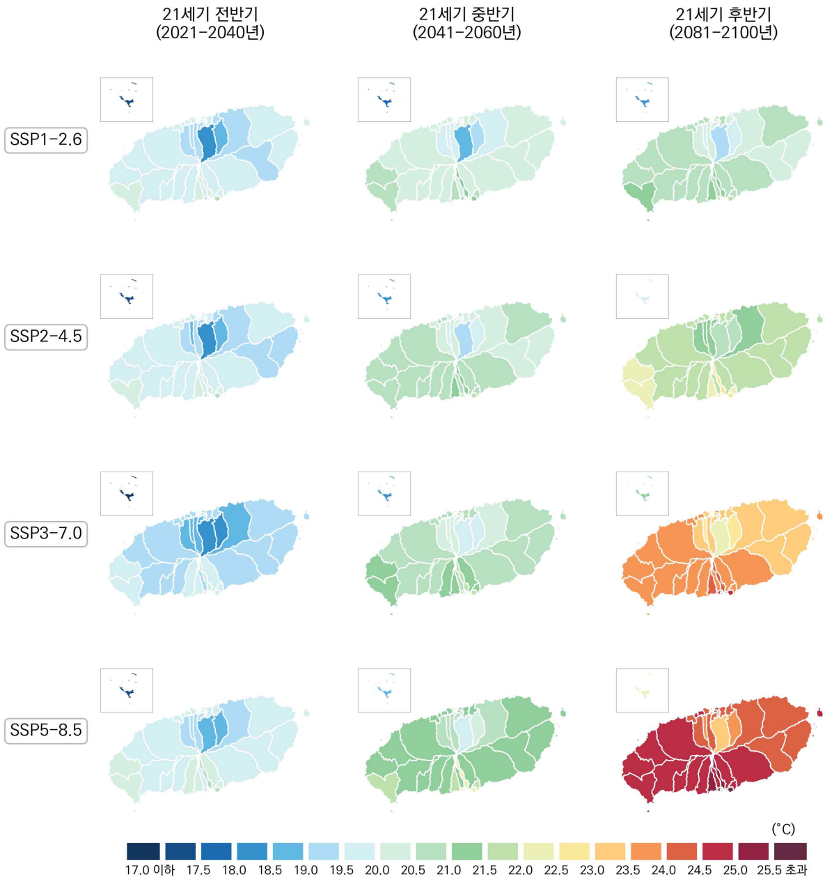
그림 4-4. 제주특별자치도의 가을철 연평균기온(°C) 전망 분포도
