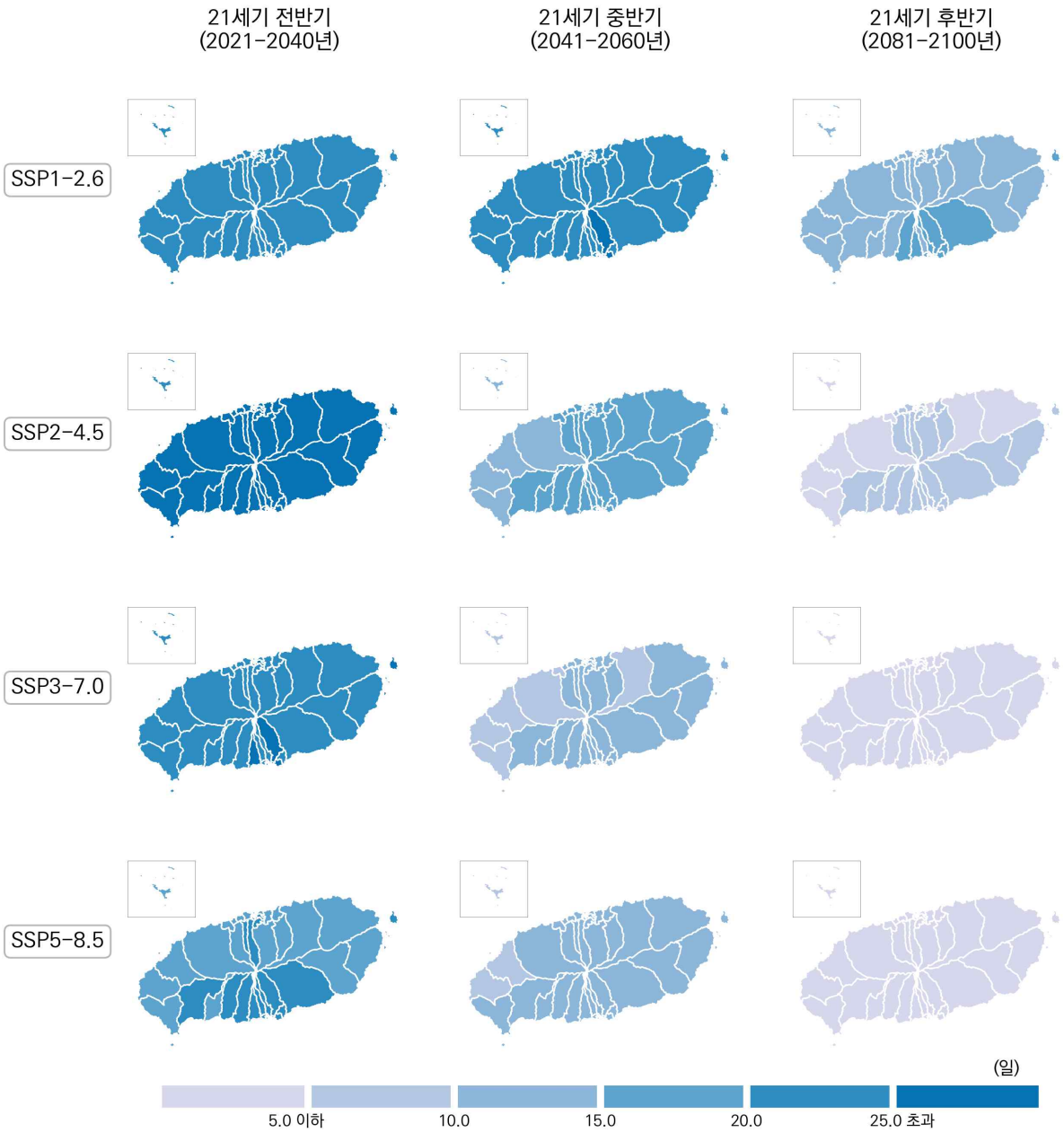
그림 4-31. 제주특별자치도의 한랭야(일) 전망 분포도
