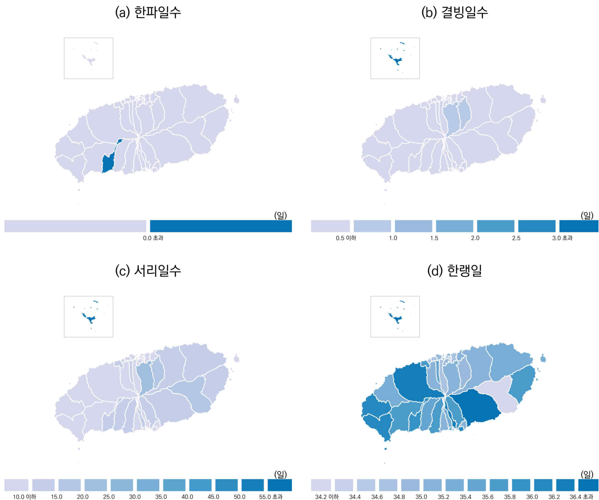
그림 3-3. 현재(2000-2019년) 제주특별자치도 저온 관련 극한기후지수 분포
