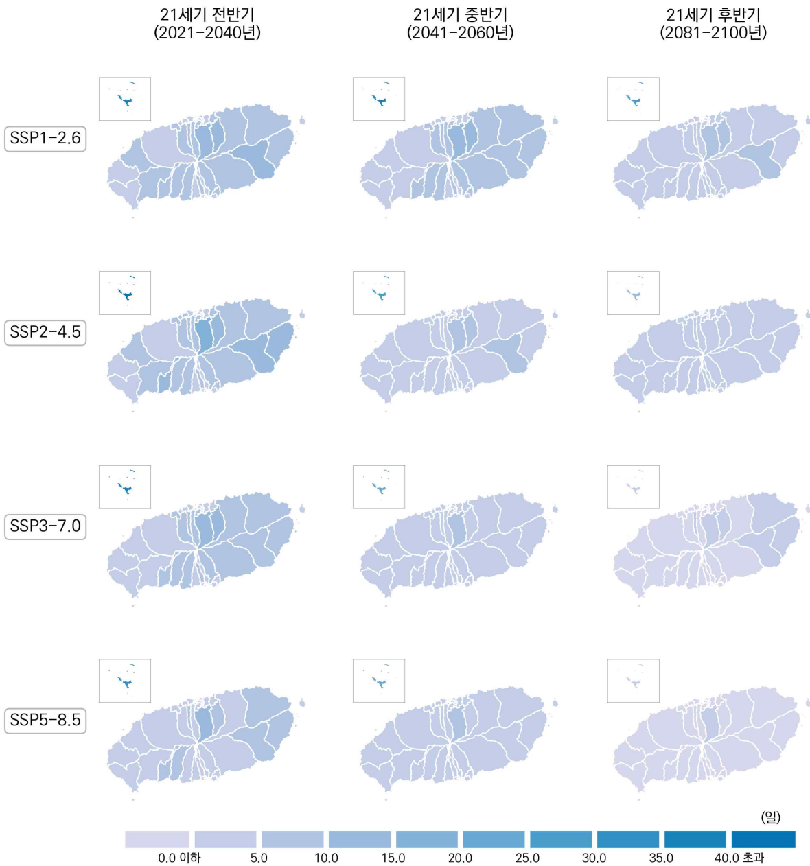
그림 4-29. 제주특별자치도의 서리일수(일) 전망 분포도
