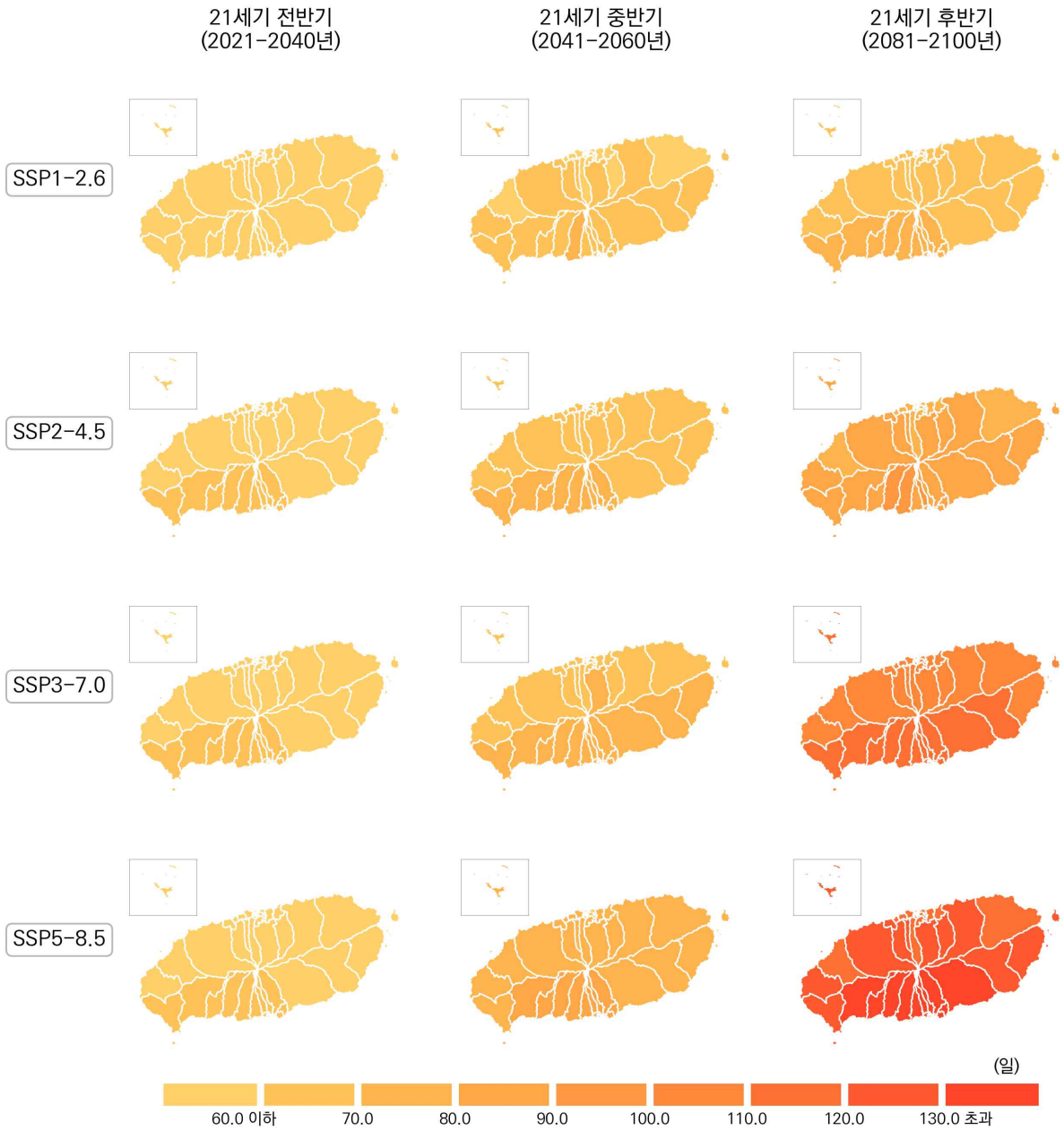
그림 4-21. 제주특별자치도의 온난일(일) 전망 분포도
