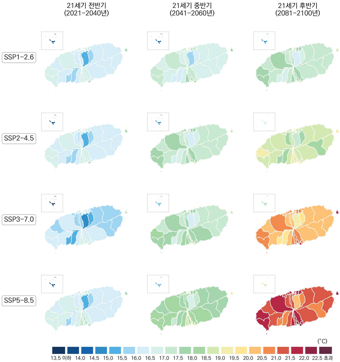
그림 4-14. 제주특별자치도의 가을철 연평균 최저기온(°C) 전망 분포도
