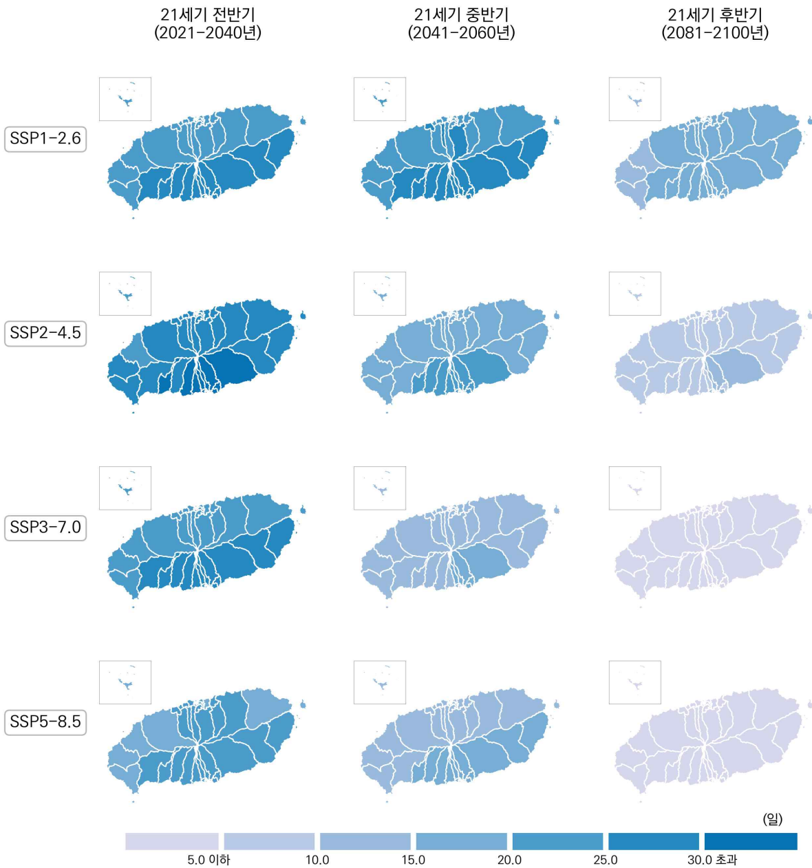
그림 4-30. 제주특별자치도의 한랭일(일) 전망 분포도
