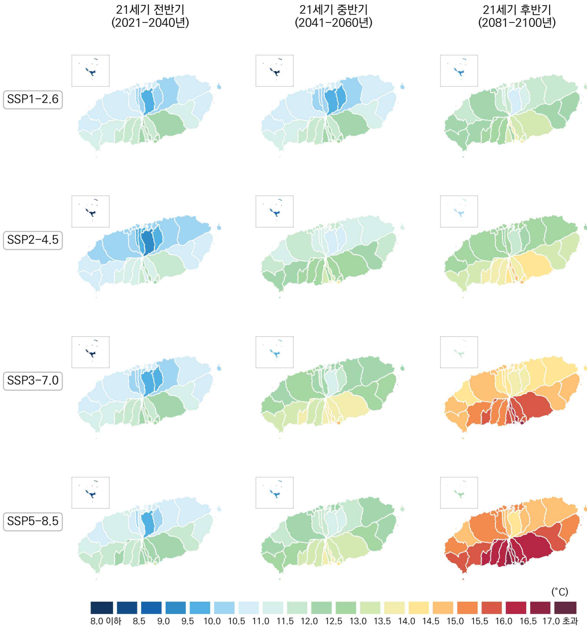
그림 4-10. 제주특별자치도의 겨울철 연평균 최고기온(°C) 전망 분포도
