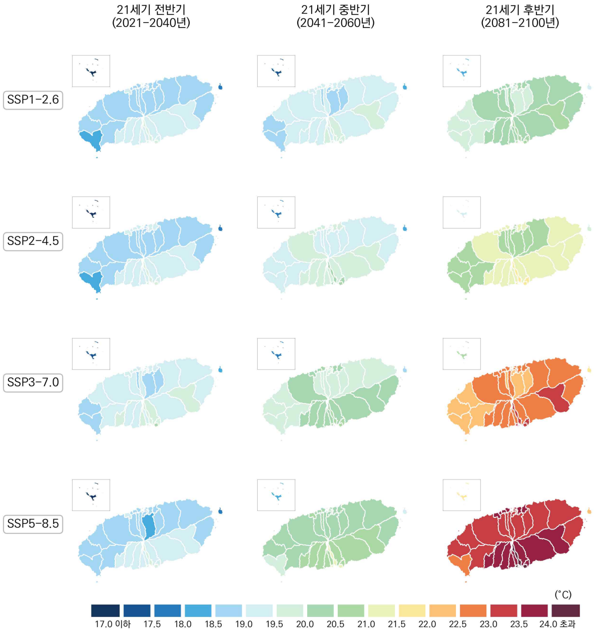
그림 4-7. 제주특별자치도의 봄철 연평균 최고기온(°C) 전망 분포도
