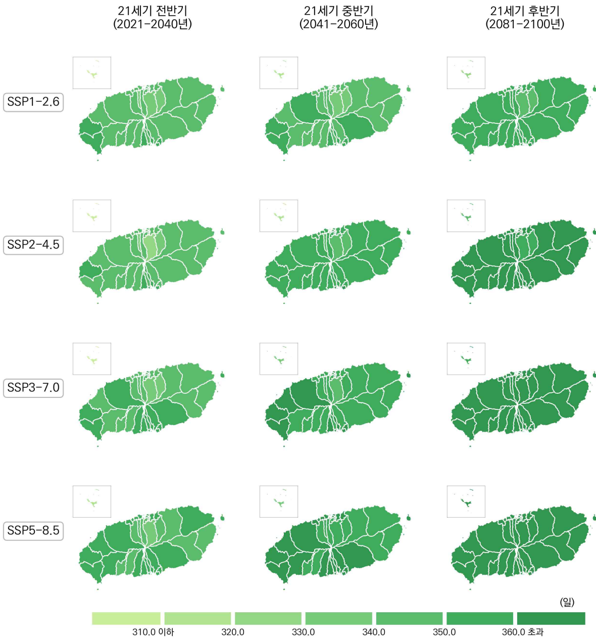
그림 4-26. 제주특별자치도의 식물성장가능기간(일) 전망 분포도
