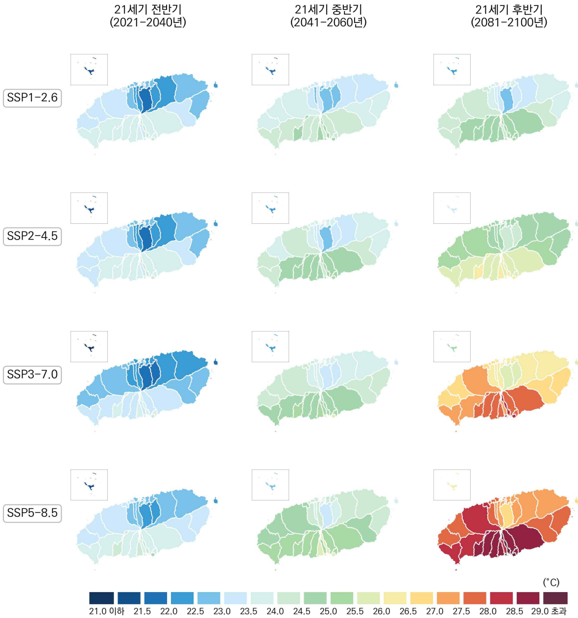
그림 4-9. 제주특별자치도의 가을철 연평균 최고기온(°C) 전망 분포도
