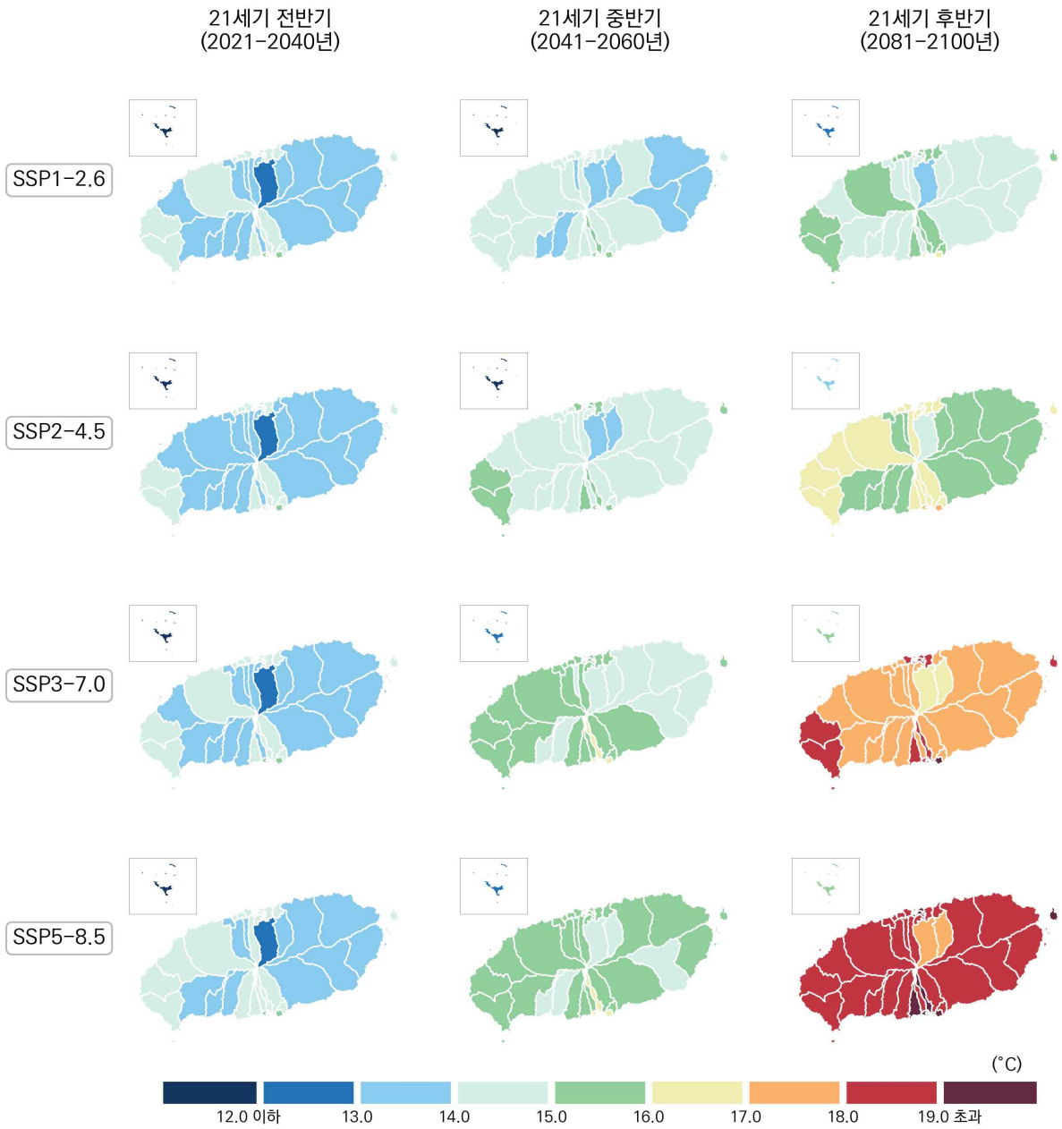
그림 4-11. 제주특별자치도의 연평균 최저기온(°C) 전망 분포도
