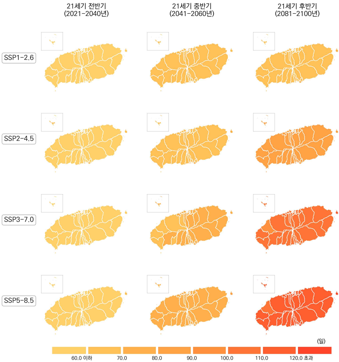
그림 4-22. 제주특별자치도의 온난야(일) 전망 분포도
