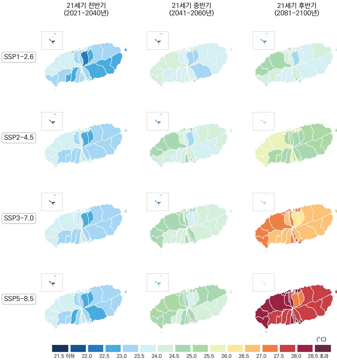
그림 4-13. 제주특별자치도의 여름철 연평균 최저기온(°C) 전망 분포도
