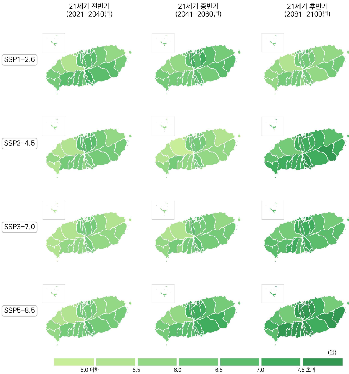
그림 4-38. 제주특별자치도의 95퍼센타일강수일수(일) 전망 분포도
