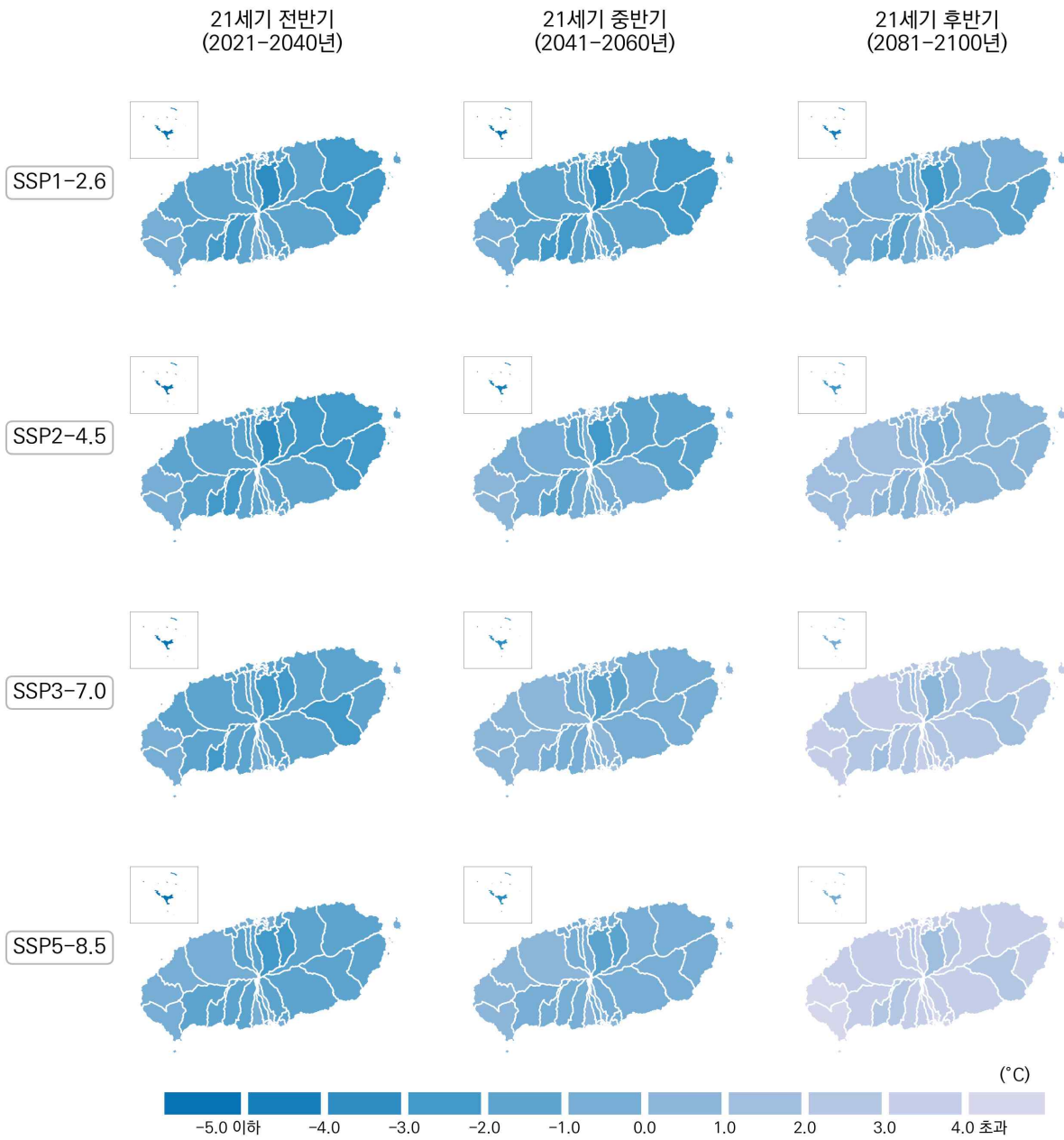
그림 4-33. 제주특별자치도의 일최저기온 연최소(°C) 전망 분포도
