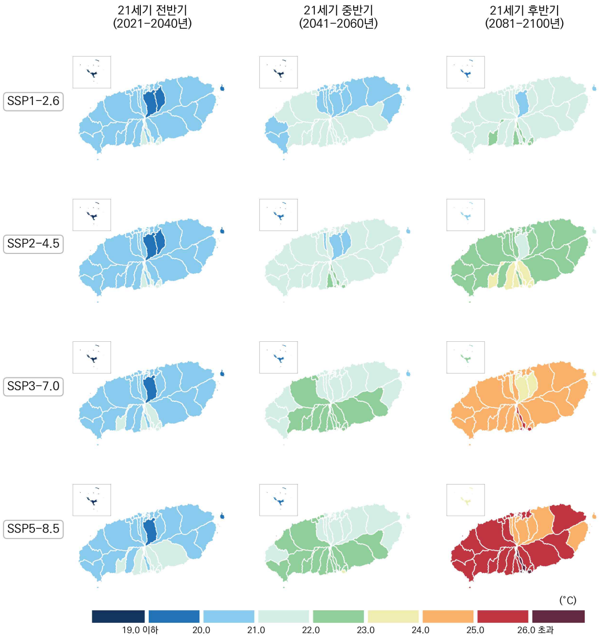
그림 4-6. 제주특별자치도의 연평균 최고기온(°C) 전망 분포도
