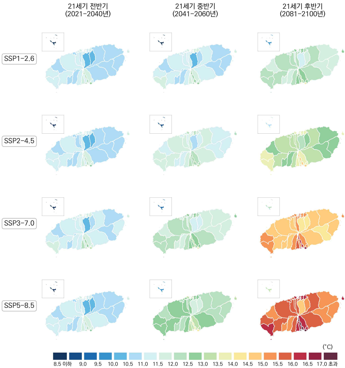
그림 4-12. 제주특별자치도의 봄철 연평균 최저기온(°C) 전망 분포도
