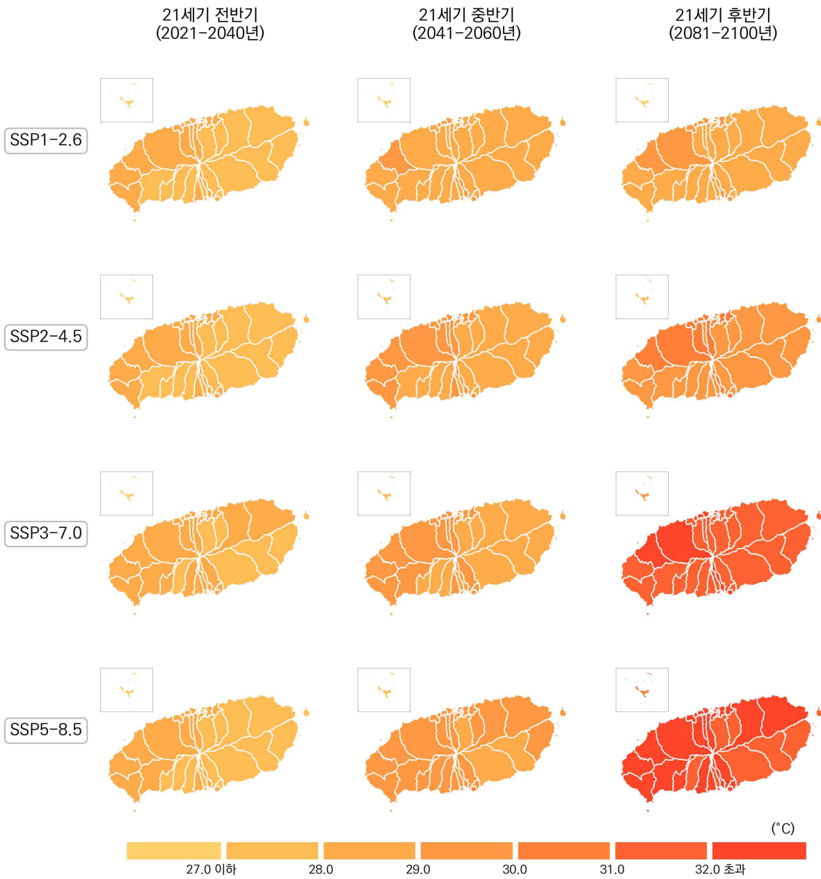
그림 4-24. 제주특별자치도의 일최저기온 연최대(°C) 전망 분포도
