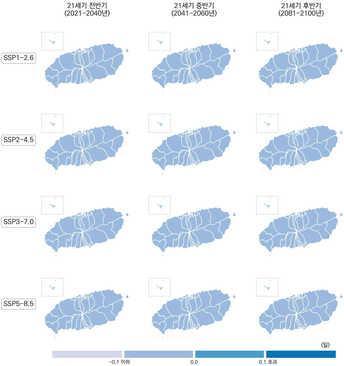
그림 4-27. 제주특별자치도의 한파일수(일) 전망 분포도
