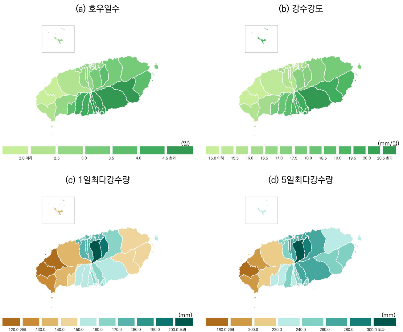
그림 3-4. 현재(2000-2019년) 제주특별자치도 강수 관련 극한기후지수 분포
