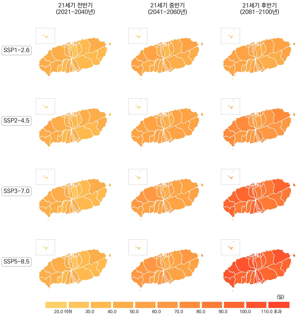
그림 4-19. 제주특별자치도의 열대야일수(일) 전망 분포도
