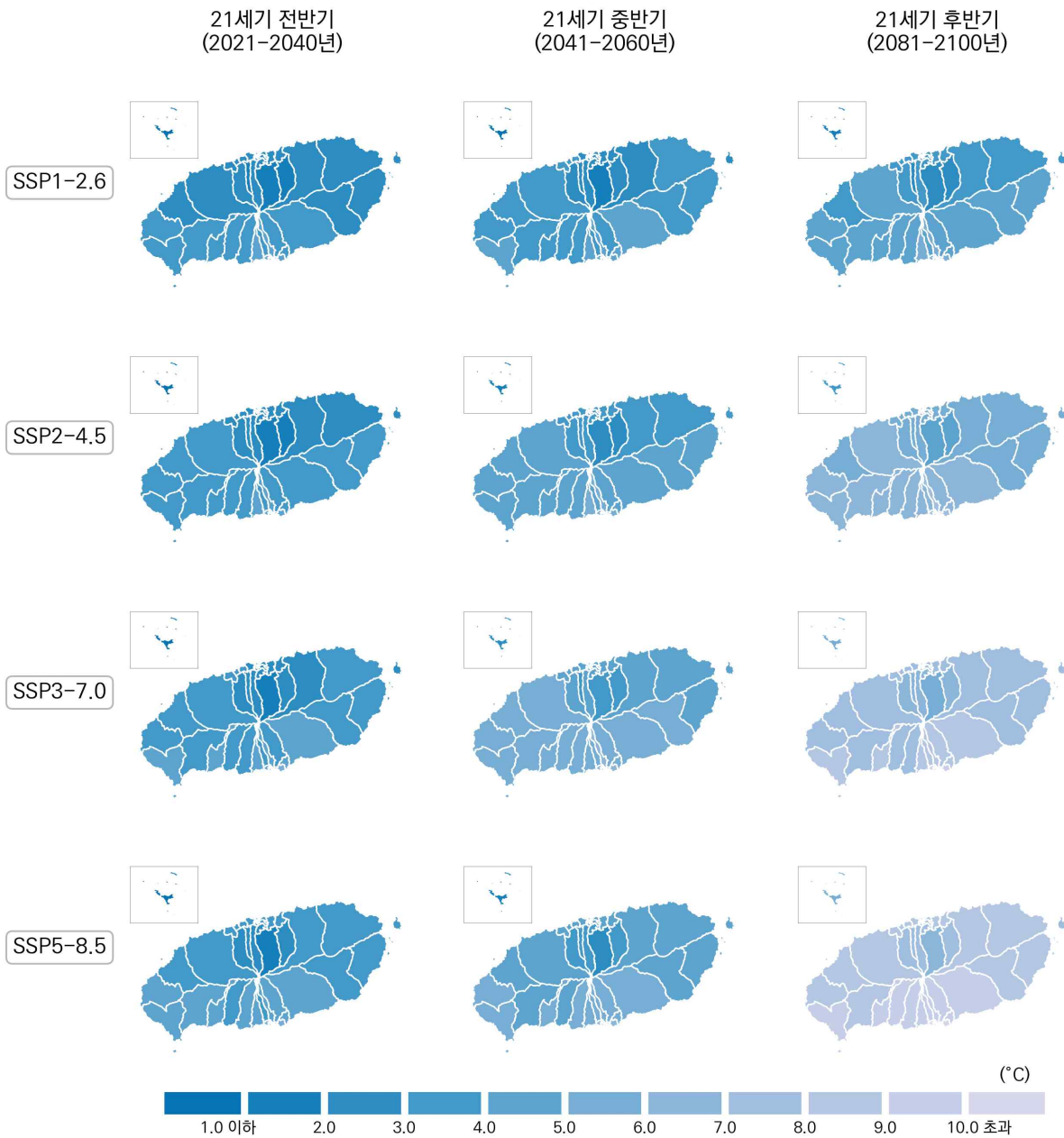
그림 4-32. 제주특별자치도의 일최고기온 연최소(°C) 전망 분포도
