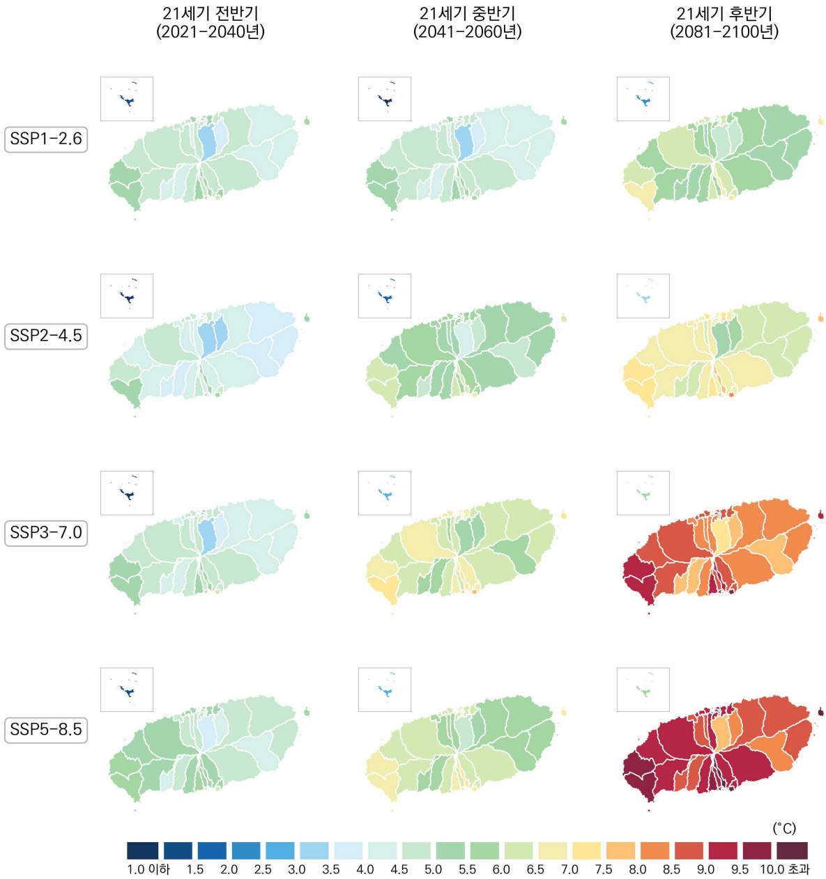
그림 4-15. 제주특별자치도의 겨울철 연평균 최저기온(°C) 전망 분포도
