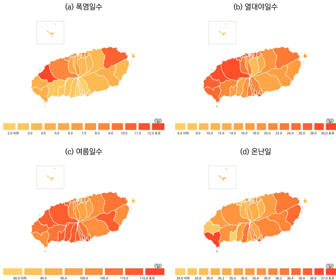
그림 3-2. 현재(2000-2019년) 제주특별자치도 고온 관련 극한기후지수 분포
