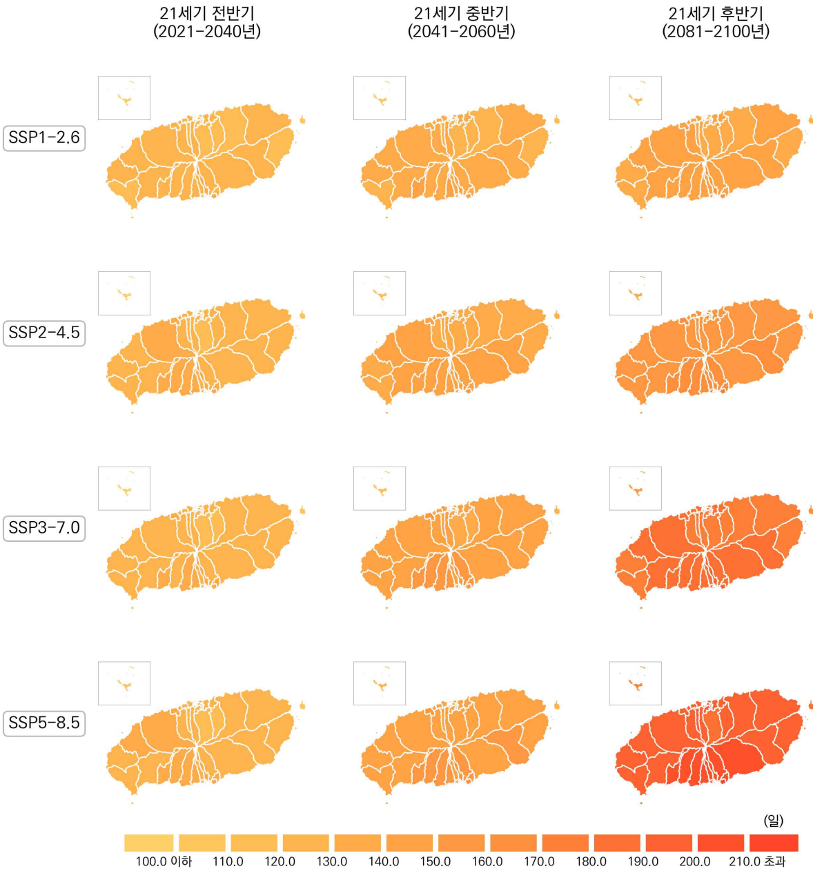
그림 4-20. 제주특별자치도의 여름일수(일) 전망 분포도
