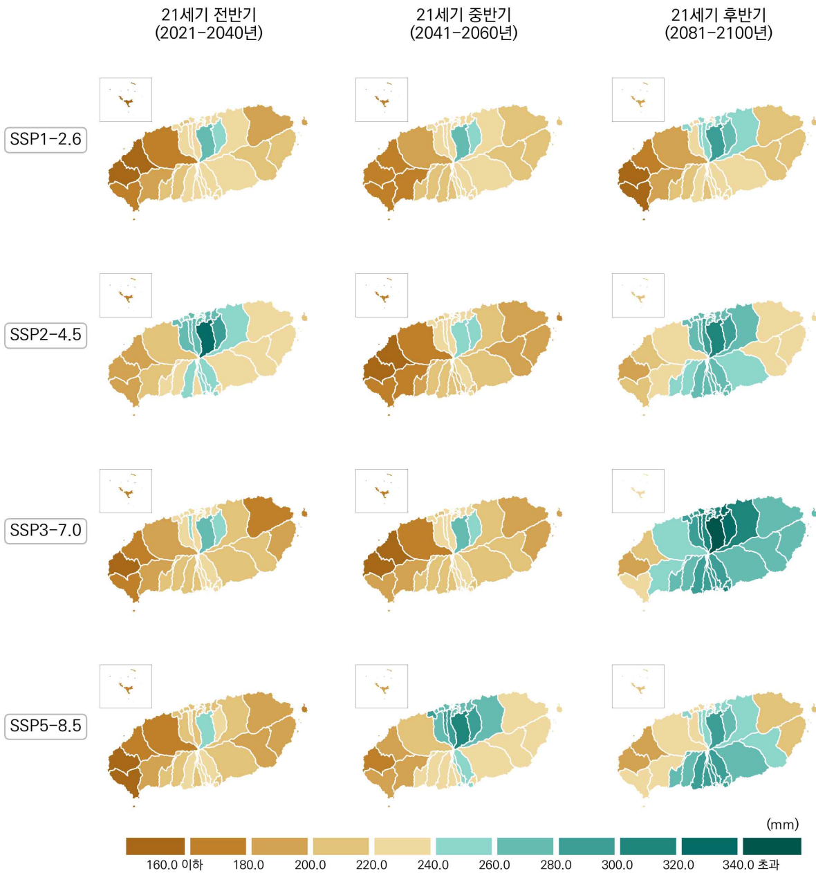
그림 4-36. 제주특별자치도의 1일최다강수량(mm) 전망 분포도
