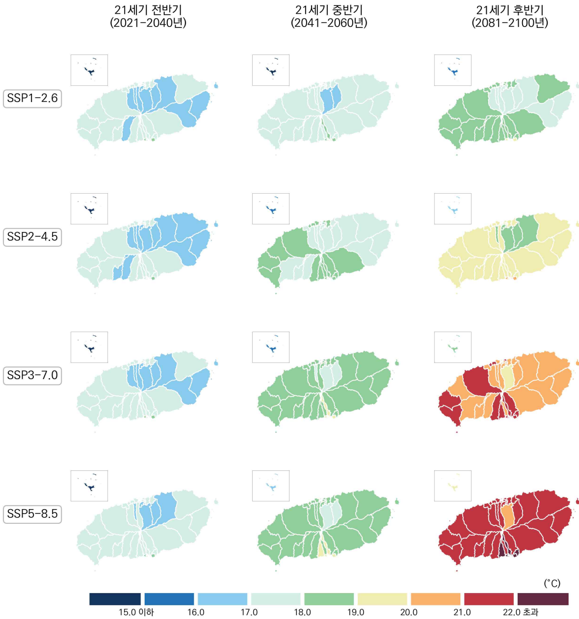
그림 4-1. 제주특별자치도의 연평균기온(°C) 전망 분포도
