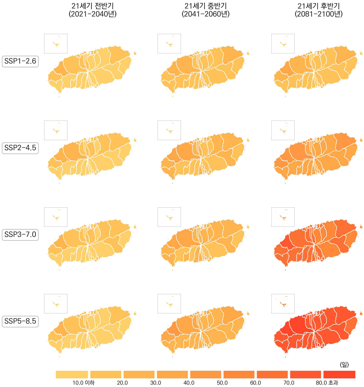
그림 4-18. 제주특별자치도의 폭염일수(일) 전망 분포도
