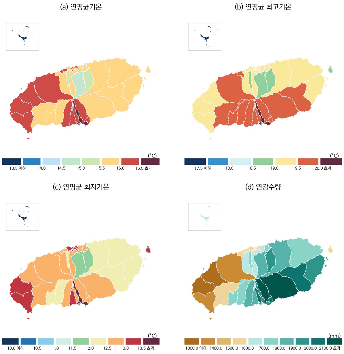
그림 3-1. 현재(2000-2019년) 제주특별자치도 기후요소 분포
