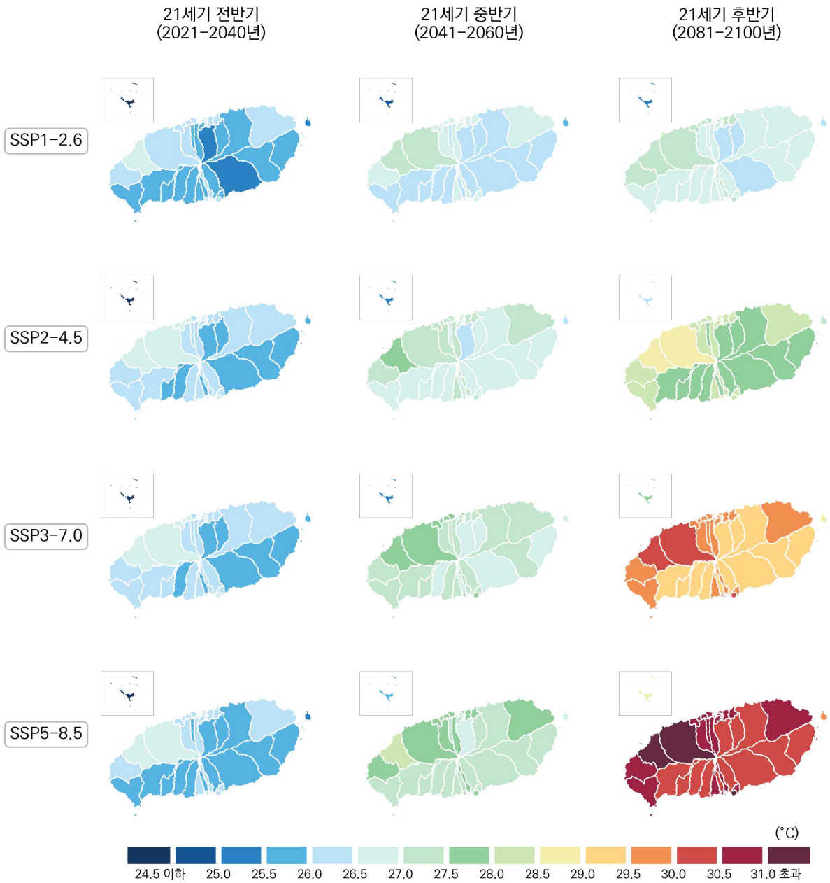
그림 4-3. 제주특별자치도의 여름철 연평균기온(°C) 전망 분포도
