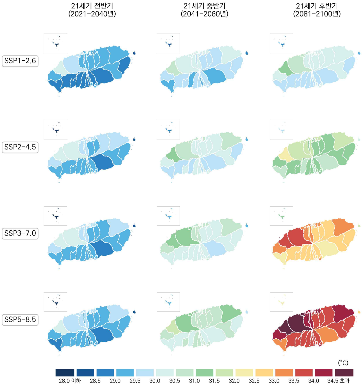
그림 4-8. 제주특별자치도의 여름철 연평균 최고기온(°C) 전망 분포도
