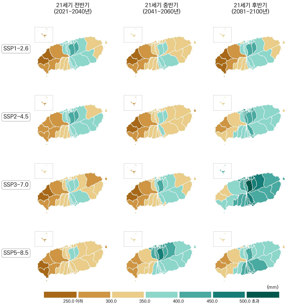
그림 4-37. 제주특별자치도의 5일최다강수량(mm) 전망 분포도
