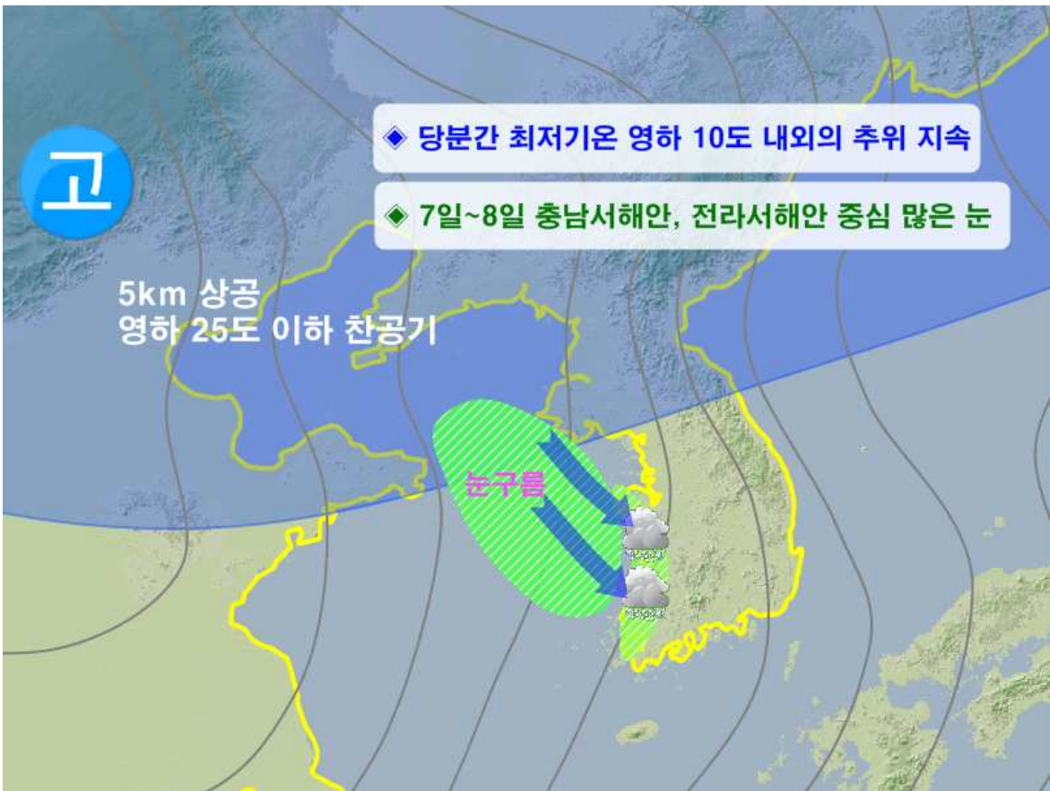
< 12월 7일~8일 기압계 모식도 >
