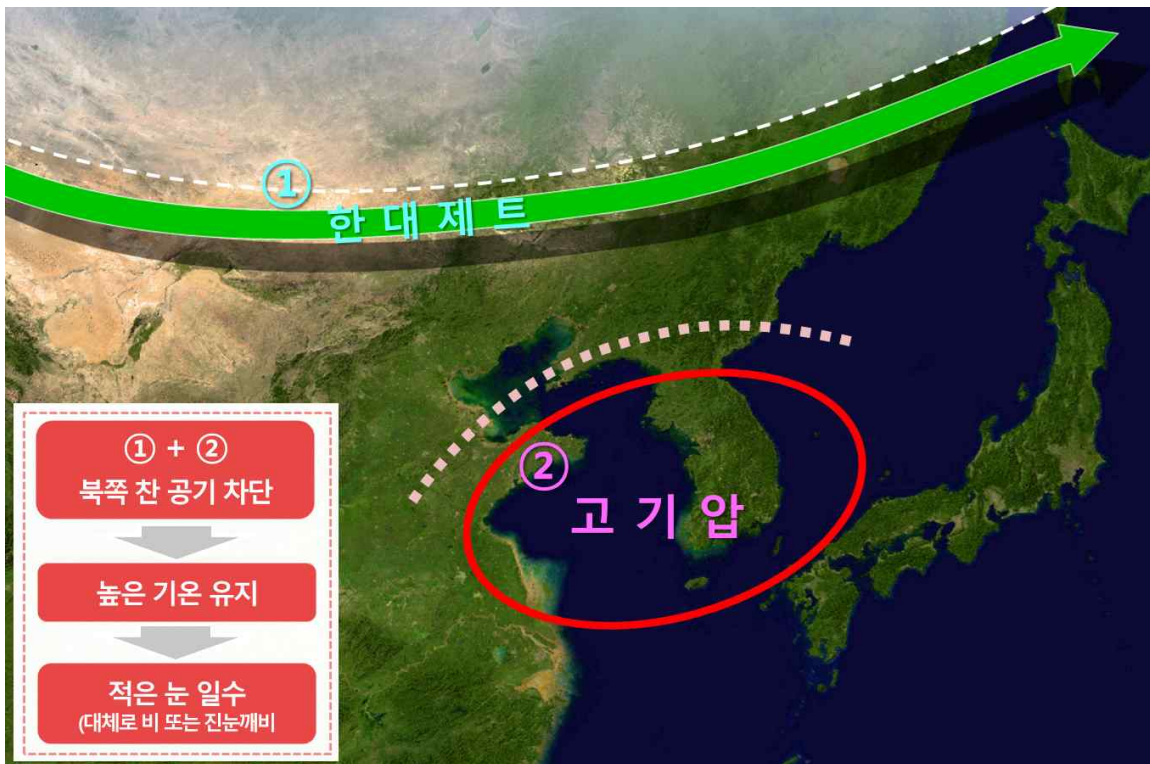
[최근 우리나라 주변 기압계 모식도]
