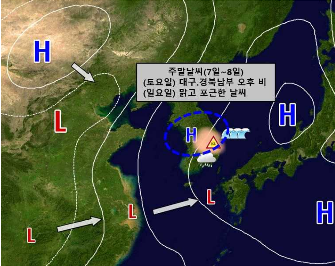
[ 3월 7~8일 ] 우리나라 주변 기압계 모식도
