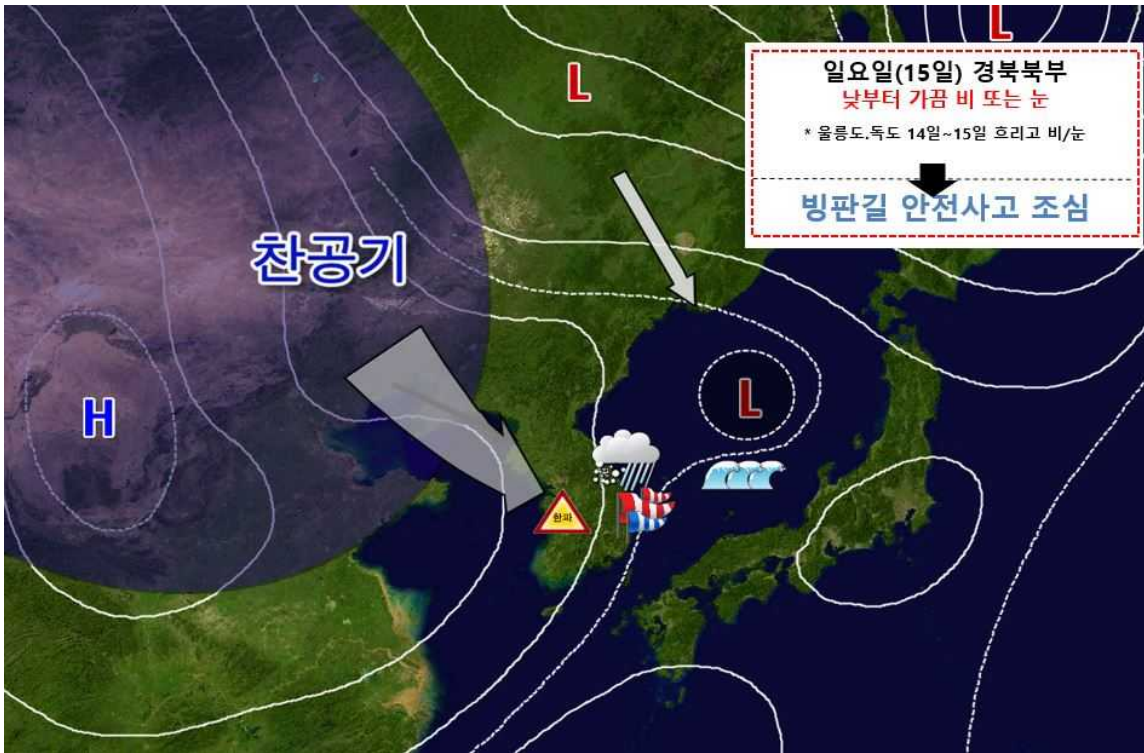
[ 3월 14~15일 ] 우리나라 주변 기압계 모식도
