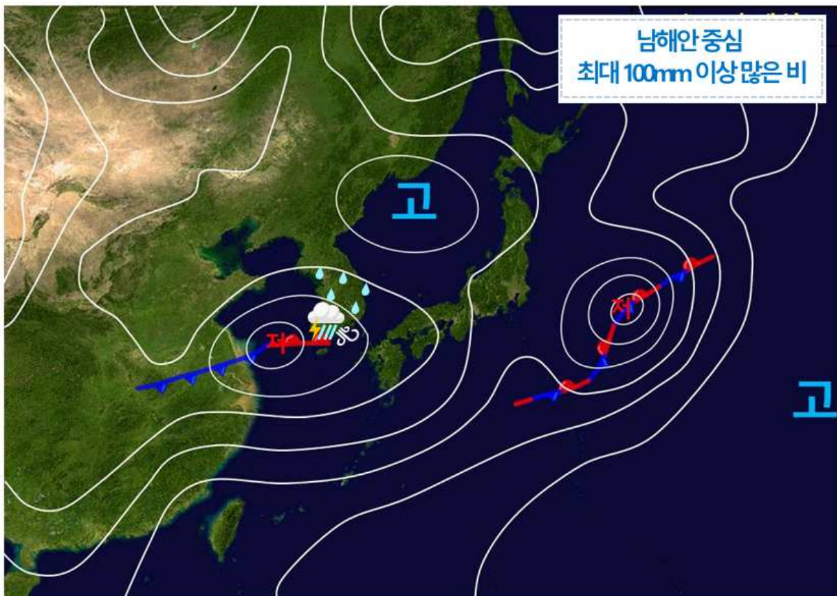
[ 6월 18일 아침 ] 우리나라 주변 기압계 모식도
