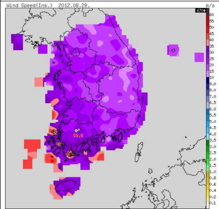
일 최대순간풍속 (8.28.)
