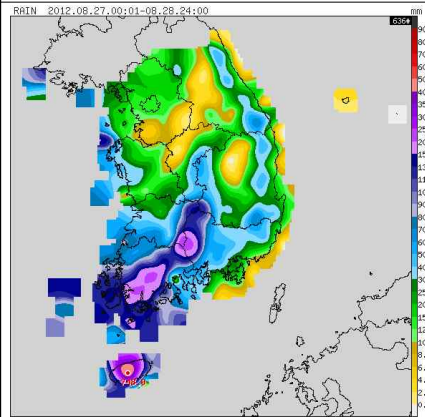
누적 강수량 (8.27.~8.28.)
