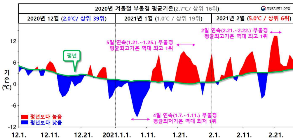
【그림 1】 2020년 겨울철 부울경 평균기온 일변화 시계열
