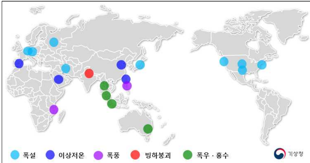
【그림 1】 2020년 12월~2021년 2월 전 세계 이상기후 현상별 발생 위치
