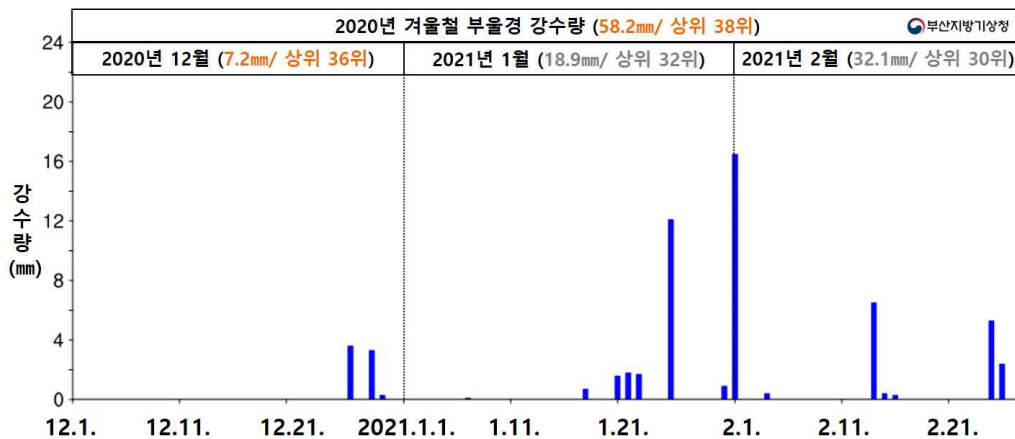
【그림 2】 2020년 겨울철 부울경 강수량 일변화 시계열
