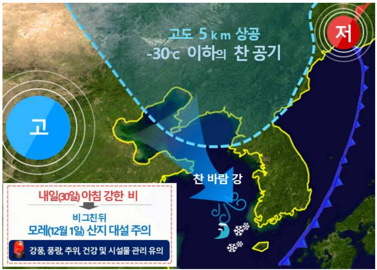
[ 11월 30일 밤 기압계 모식도 ]
