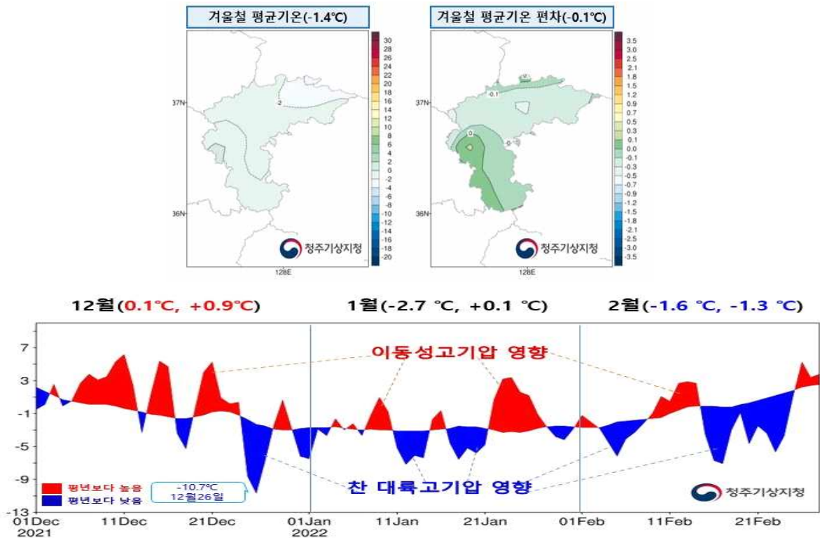
【그림1】 겨울철(2021년 12월~ 2022년 2월) 충북 평균기온 분포도 및 시계열
