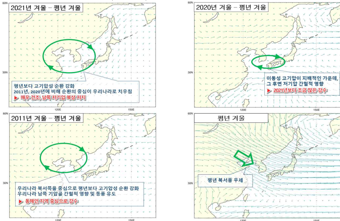
【그림 2】 850hPa(고도 약 1.5km 상공) 바람벡터
