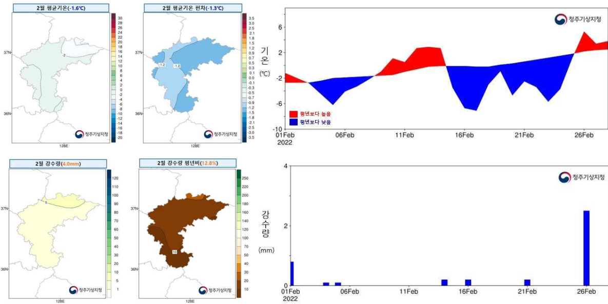
[그림 1] 충북 2월 평균기온과 편차 분포도 및 시계열(위), 강수량과 강수량 평년비 분포도 및 시계열(아래)
