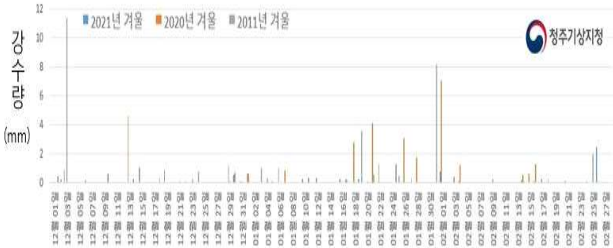
【그림 1】 2021년, 2020년, 2011년 겨울철 총북 일강수량 그래프
