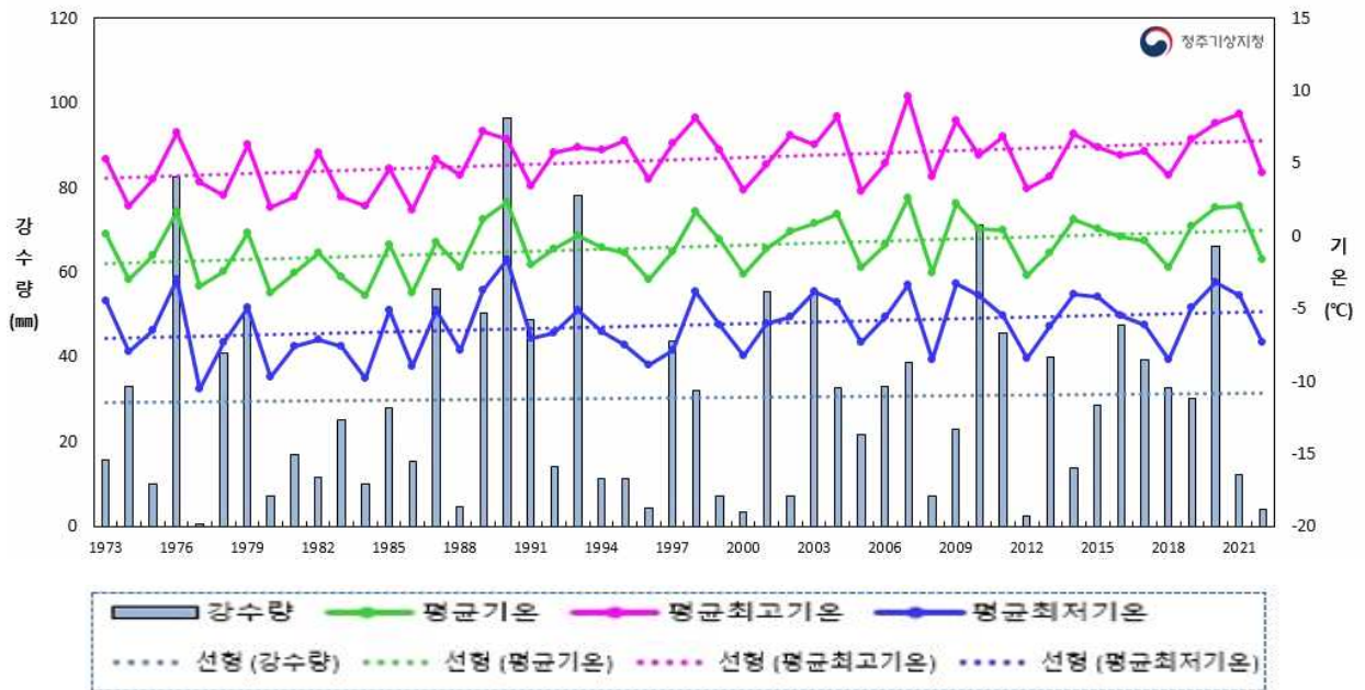
[그림 2] 2022년 2월 충북 기상자료 특성(1973~2022)
