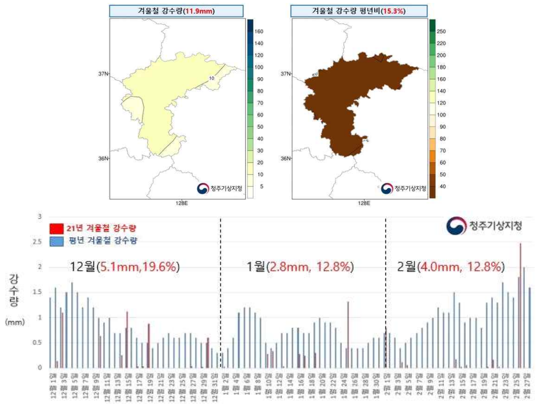
【그림2】 겨울철(2021년 12월~ 2022년 2월) 충북 강수량 분포도 및 시계열
