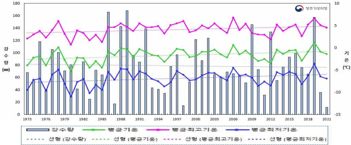
[그림 1] 겨울철 충북 기상자료 특성(1973~2021)
