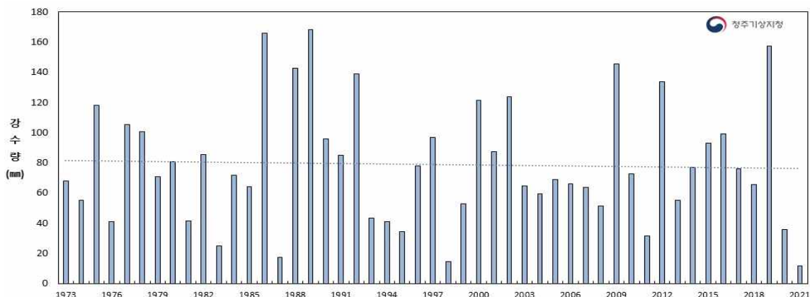
【그림 1】 충청지역 겨울철 강수량(1973~2021)
