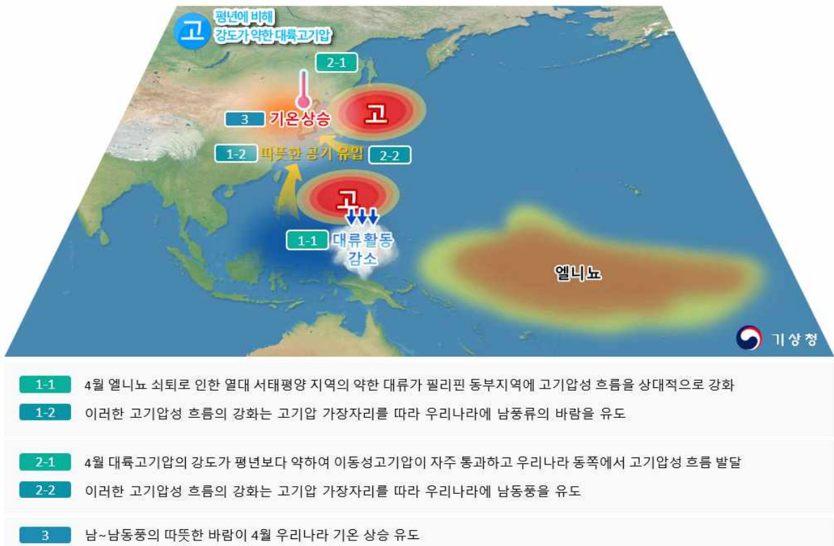
【그림 1】 2024년 4월 높은 기온 관련 기압계 모식도
