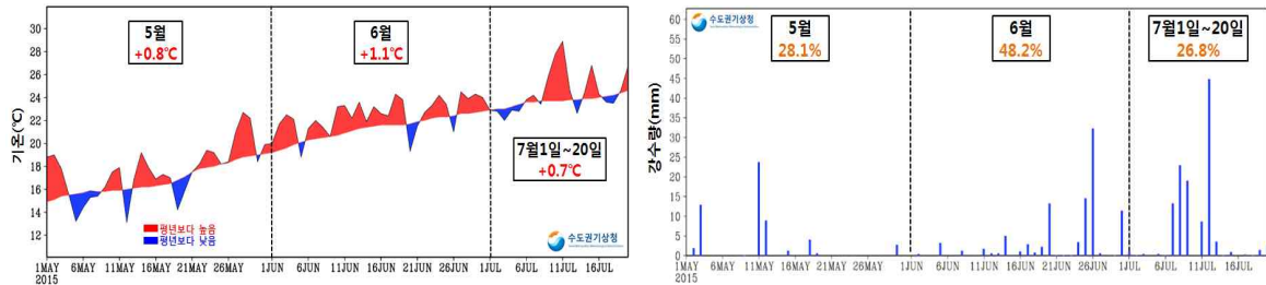
최근 3개월 평균기온(좌)과 강수량(우)의 일변화 (2015.5.1~2015.7.20)
