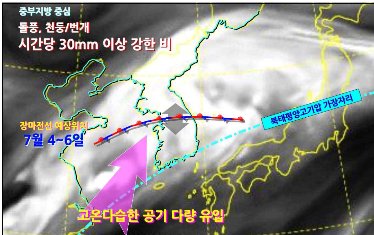
< 2016년 7월 4일~6일 장마 예상 모식도 >
