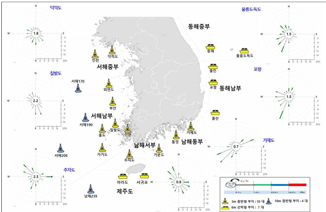
< '21년 5월 해양기상부이 해상풍 바람장미 >
